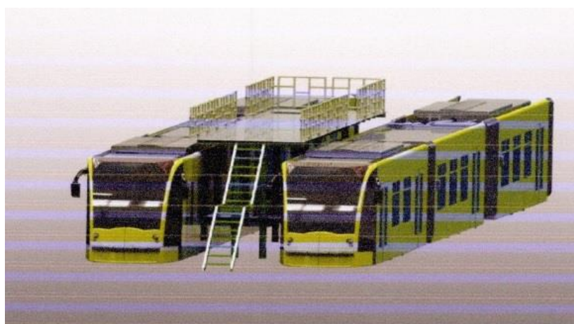
شکل ۹- تصویر عرشه‌های دسترسی (T Type-L Type) از تجهیزات ثابت قابل نصب در فونداسیون
