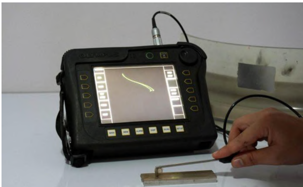
شکل ۲۱- دستگاه پرتابل التراسونیک شناسایی درز و ترک و خرابی های جوشکاری (Portable Ultrasonic flaw Detector)
