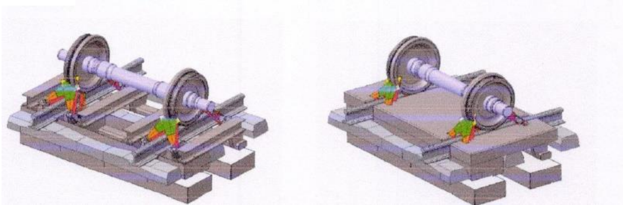
شکل ۱۳- تصویر شماتیک ایستگاه بازرسی چرخ از تجهیزات ثابت قابل نصب در فونداسیون
