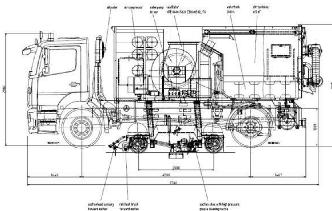
شکل ۱-۱-۱ ماشین شستشوی تونل
