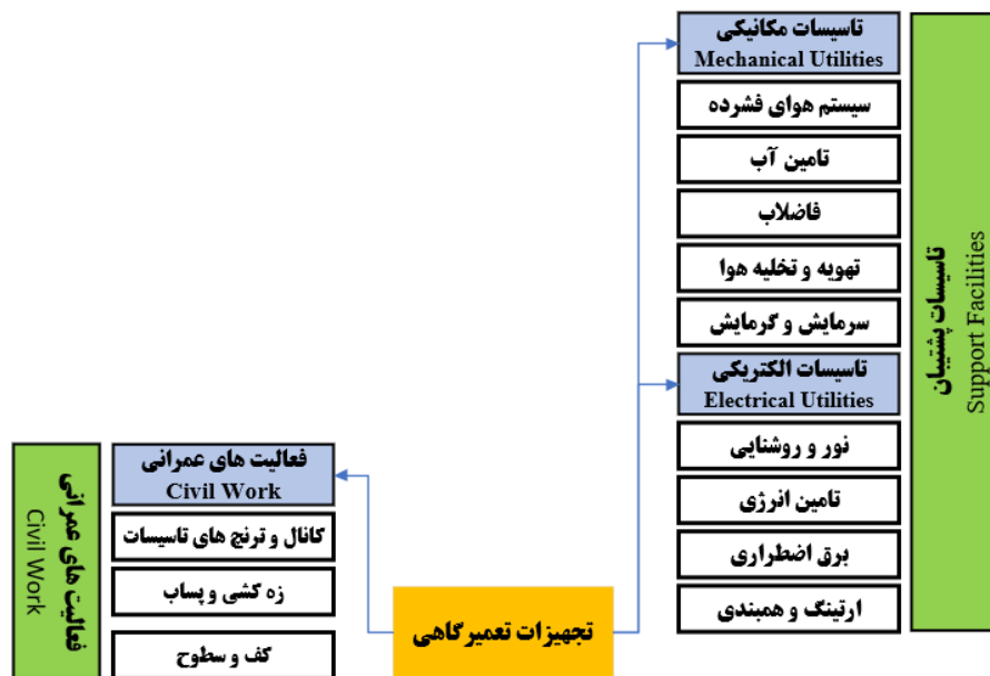
شکل ۲۷-۲۷ محدوده اینترفیس ماشین‌آلات مکانیزه (تجهیزات شستشو)
