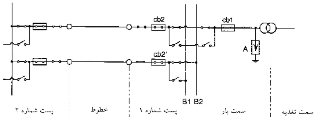
شکل ۲-۱۰: آرایش سیستم مورد استفاده در مثال طراحی
