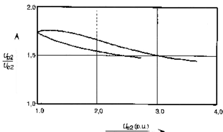
شکل ۲-۲: نسبت بین مقادیر ۲ درصدی اضافه ولتاژهای با شیب کند فاز به فاز و فاز به زمین
