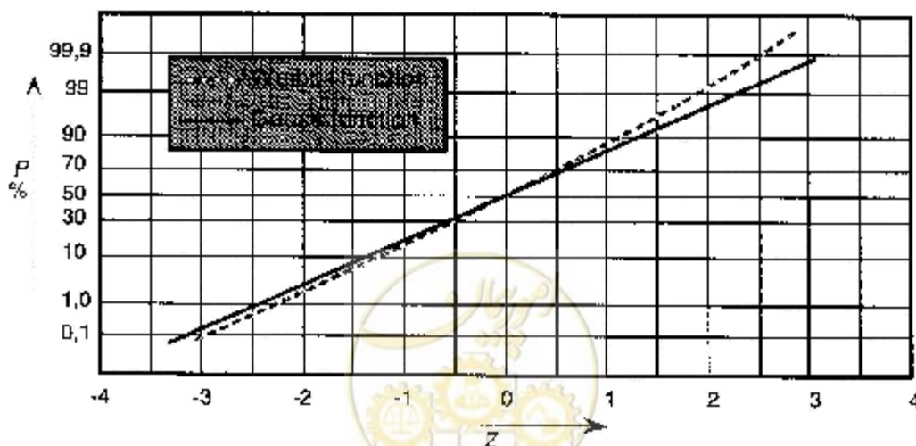
شکل ۲-۵: مقایسه توابع احتمال توزیع گوسی و توزیع وی بال براساس مقیاس گوسی
