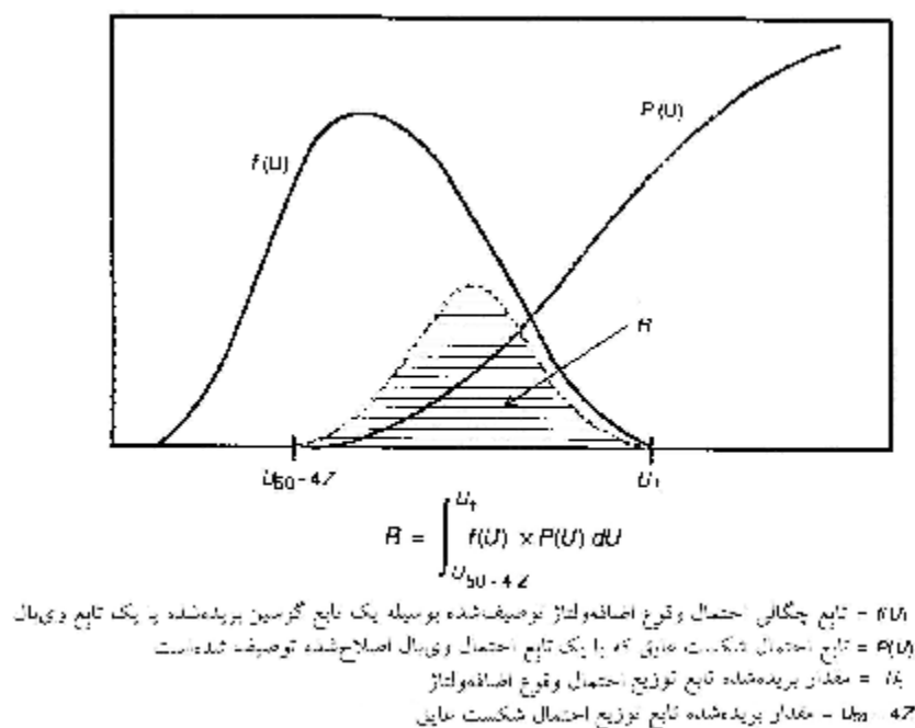
شکل ۷-۲: ارزیابی نرخ خطا در روش آماری هماهنگی عایقی امواج ضربه با شیب کند
