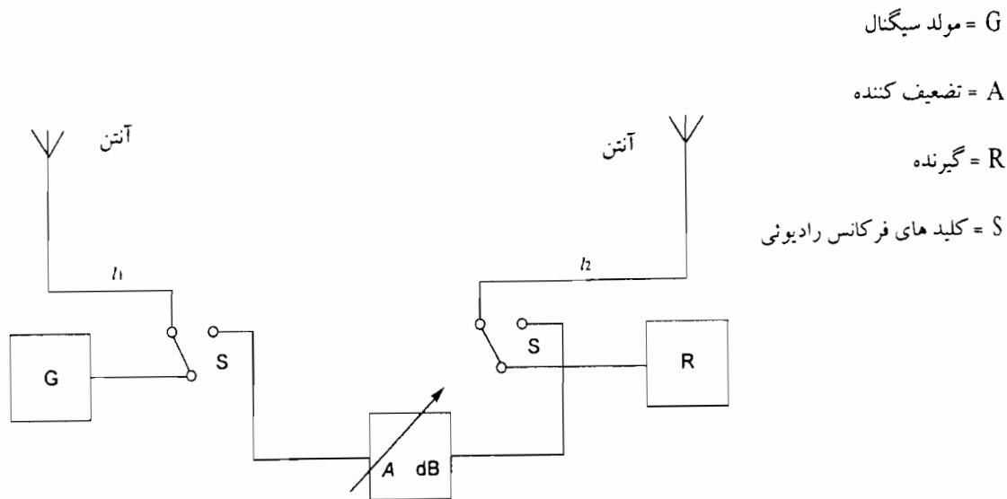
شکل ۴-۶ ترتیب مداری برای اندازه گیری اتلاف سیستم
