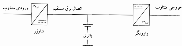
شکل ۸-۳ - سیستم یو - پی - اس ایستا برای مصارف کم و استفاده دائم
