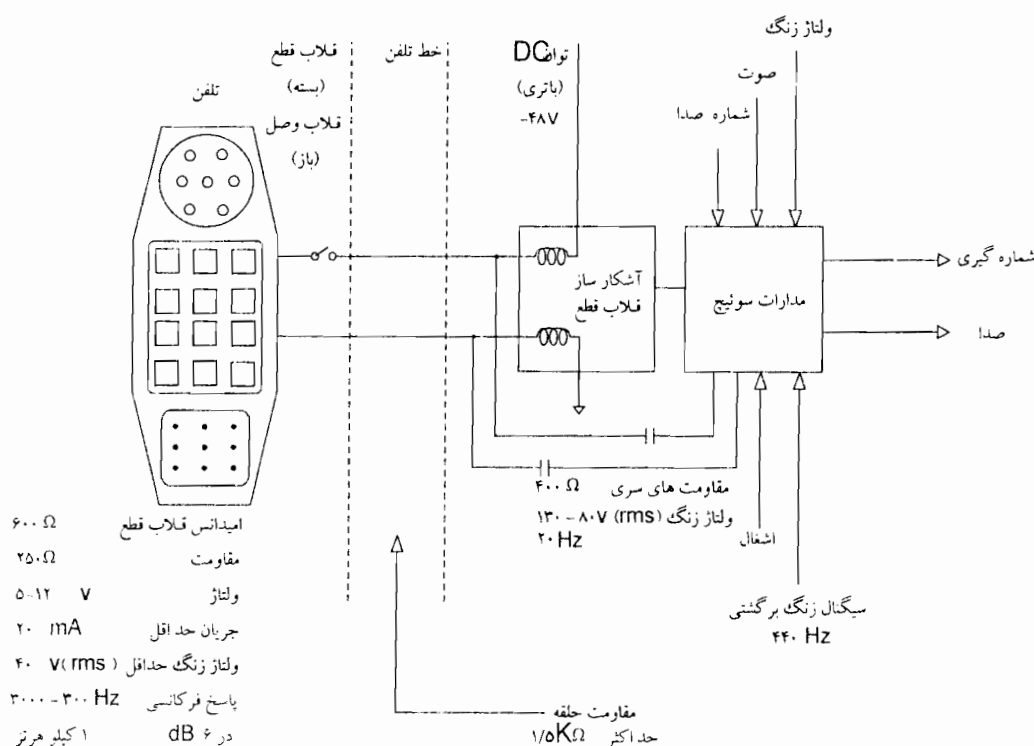
شکل ۶-۲: مشخصات اساسی تلفنهای و ارتباط آن با مراکز تلفن
