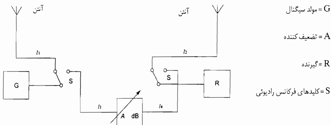
شکل ۴-۴ ترتیب مداری برای اندازه گیری اتلاف سیستم
