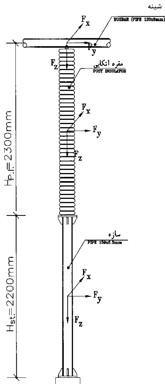
شکل ۳-۱: بارگذاری سازه نگهدارنده مقره اتکایی
