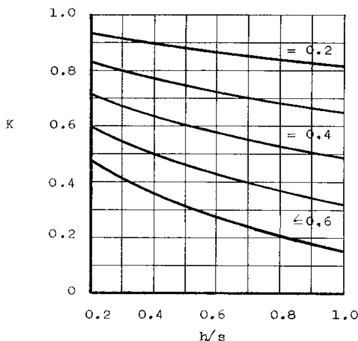
شکل ۲-۱: ضریب پوشش K به ازای Uهای متفاوت
