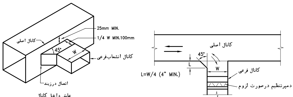
انشعاب کانال چهارگوش
