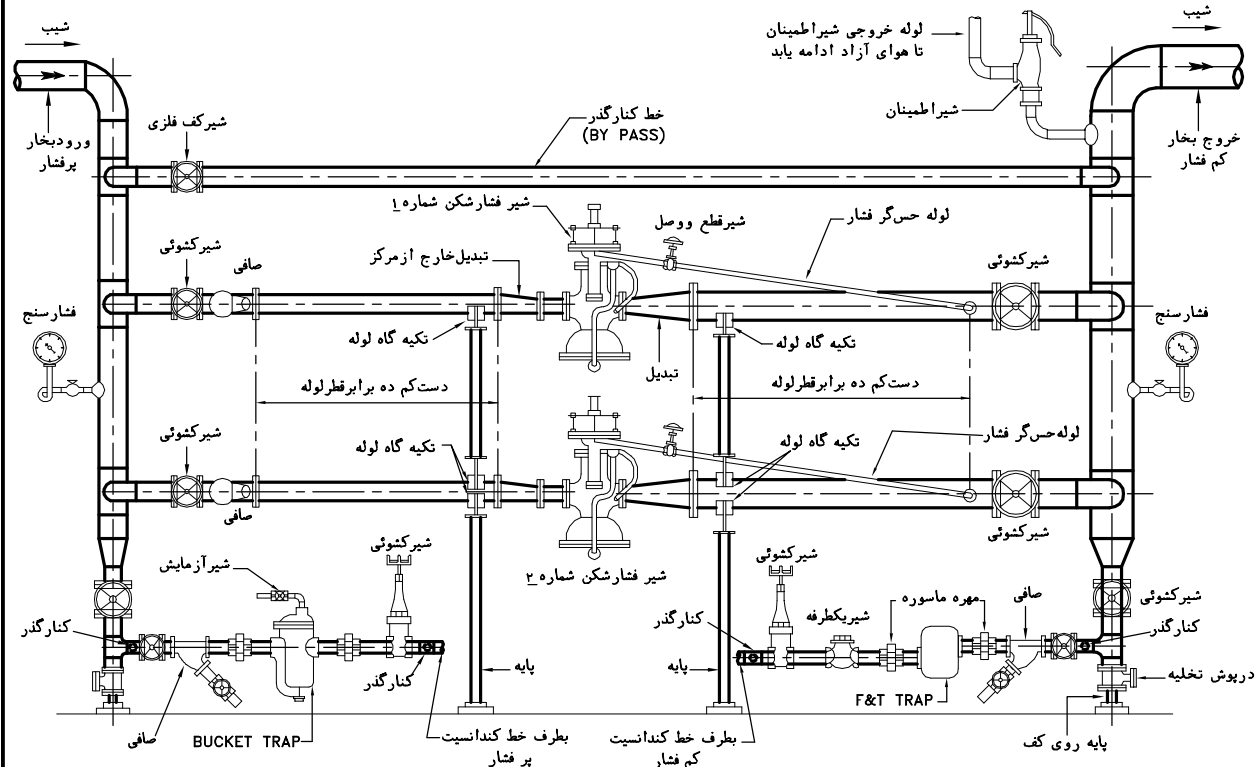
نمای ایستگاه تقلیل فشاربخار یک مرحله ای
