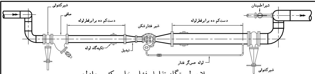
پلان ایستگاه تقلیل فشاربخار یک مرحله ای
