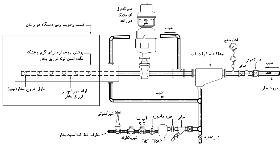
رطوبت زن بخاری با شیرکنترل دورا
