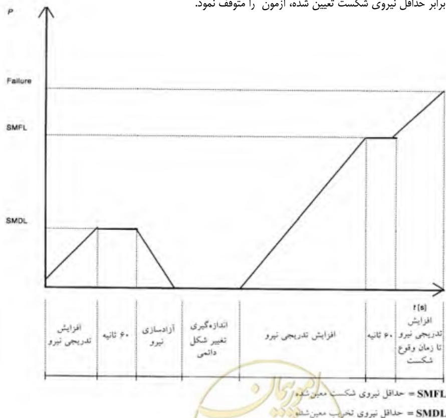
شکل ۳-۲: نحوه اعمال نیرو در آزمون نیروی تخریب و نیروی شکست مکانیکی مربوط به یراق آلات مجموعه مقره و یراق آلات سیم زمین
