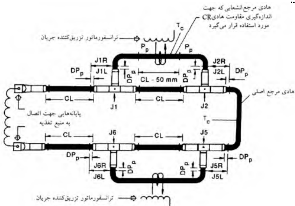
شکل ۳-۲۶: مدار نمونه جهت آزمون دوره حرارتی مفصل‌های رده B- سائز هادی‌های اصلی و انشعابی با هم متفاوت است.
