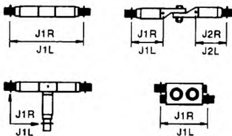
شکل ۳-۲۸: نقاط پتانسیل برای انواع مفصل‌های غیر کششی
