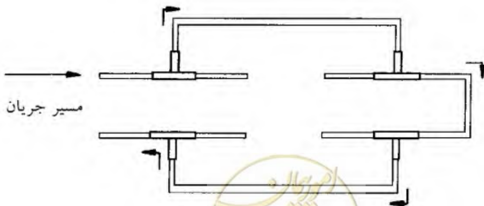
شکل ۳-۲۷: مدار نمونه جهت آزمون دوره حرارتی مفصل‌های رده B- سائز هادی‌های اصلی و انشعابی یکسان است.
