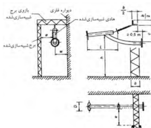
شکل ۳-۱۳: آرایش آزمونی برای ساختار کششی (آرایش دوم)
