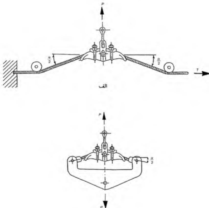
شکل ۳-۳: نحوه اعمالی نیرو در آزمون نیروی تخریب و نیروی شکست مکانیکی مربوط به کلمپ آویزی
