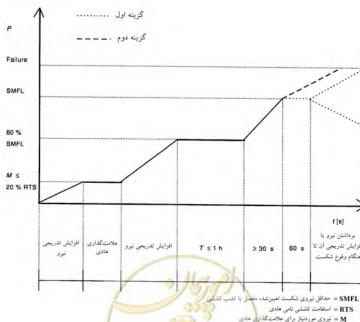
شکل ۳-۷: نرخ افزایش نیرو در آزمون کشش اعمالی به کلمپهای کششی، مفصل‌های کششی انتهایی و مفصل‌های کششی
