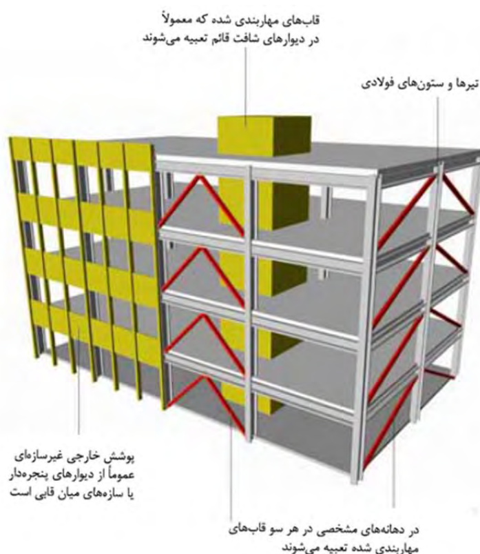
شکل 8-1- قابهای مهاربندی فولادی
