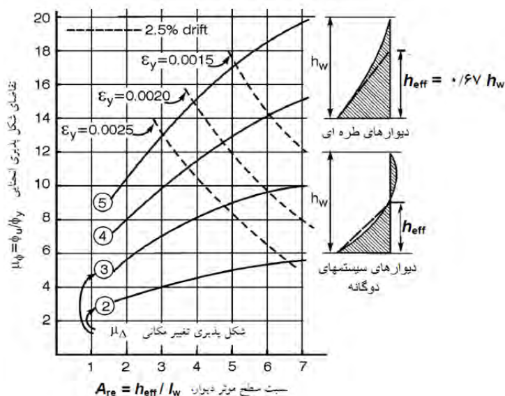
شکل الف-7- ظرفیت شکل پذیری انحنایی مورد نیاز در دیوارهای طره‌ای که تابع شکل پذیری تغییر مکانی تقاضا و نسبت سطح می‌باشد
