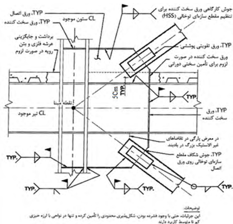
شکل 7-4- مهاربند ساخته شده از مقاطع سازه ای توخالی در اتصال تیر به ستون موجود در قابهای مهاربندی معمولی
