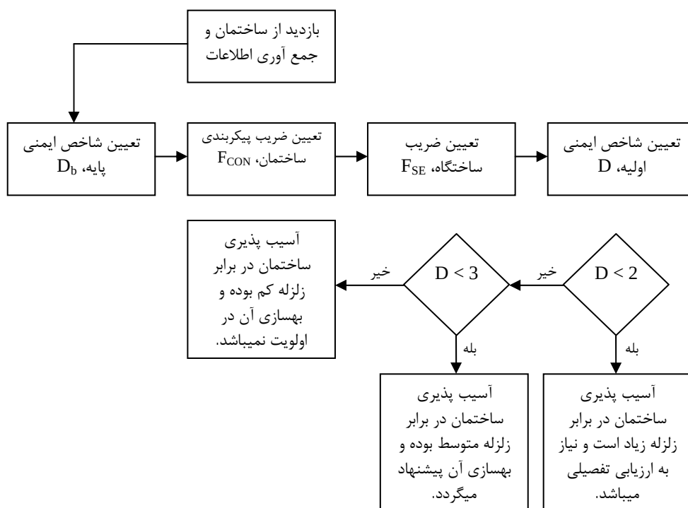
نمودار 1-2- فرآیند ارزیابی اولیه آسیب پذیری
