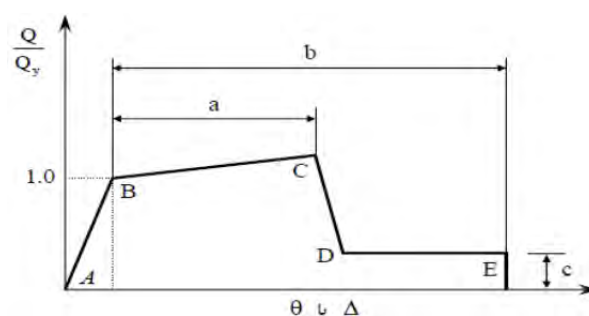
شکل 1-6- منحنی نیرو- تغییر شکل تعمیم یافته برای اجزای فولادی
