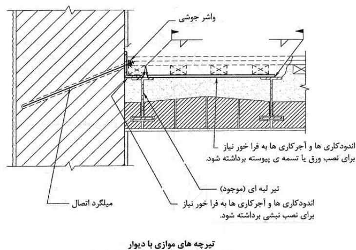
شکل 10-5- افزودن مهارهای دوخت و عضو مرزی دیوار به دیافراگم طاق ضربی - در صورت دسترسی از بالای کف
