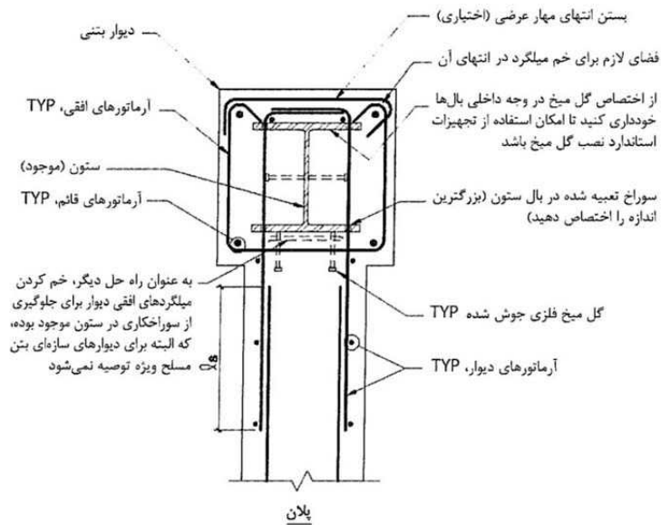
شکل 7-8- مدفون شدن ستون در دیوار بتنی درجا
