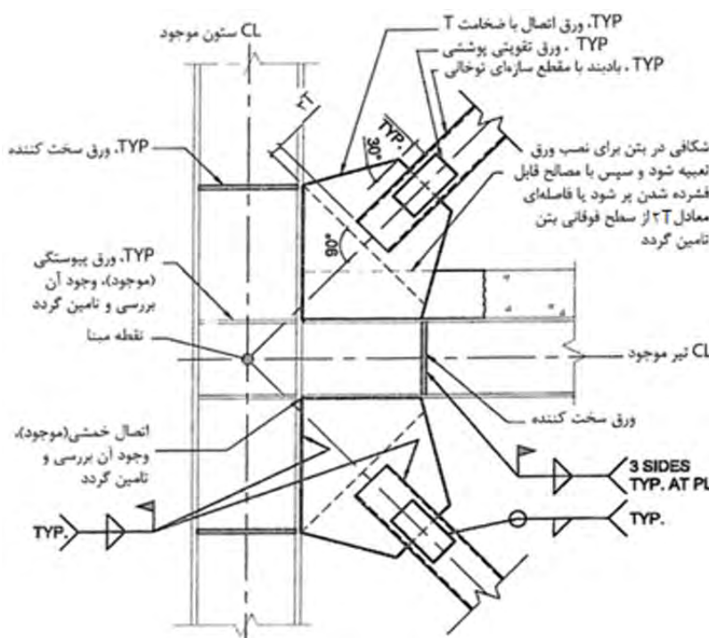
شکل 3-7- مهاربند ساخته شده از مقاطع سازه‌ای توخالی در اتصال تیر به ستون موجود در قابهای مهاربندی ویژه
