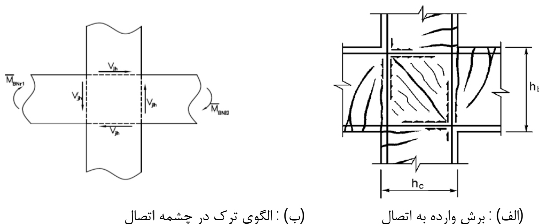
شکل الف-2- اتصال داخلی تیر - ستون در هنگام بارهای لرزه‌ای
