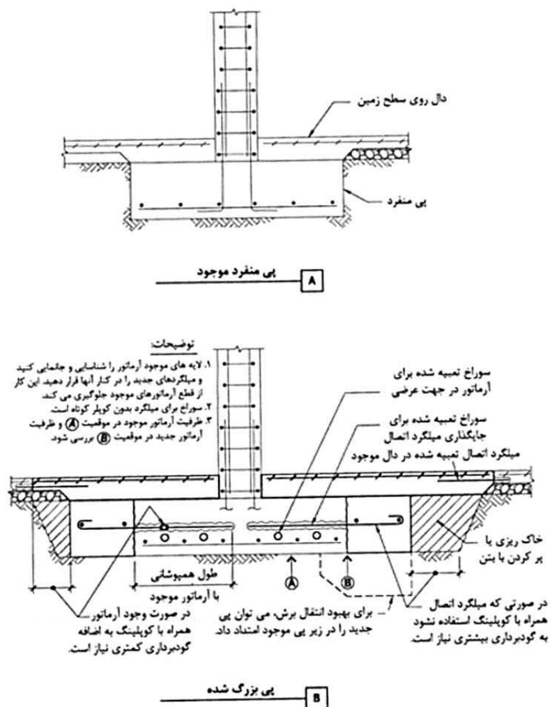
شکل 11-7- بزرگ کردن پی منفرد موجود
