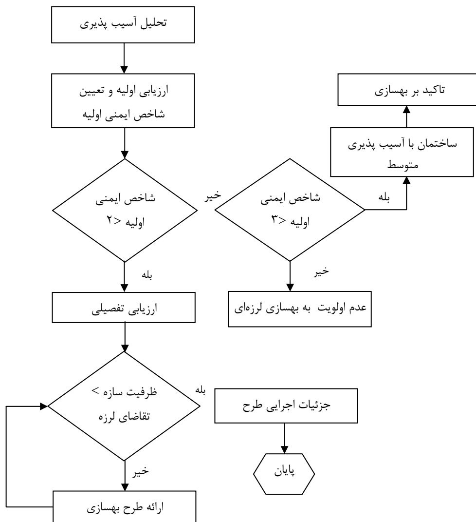
نمودار 1-1-1- روند تحلیل و ارزیابی آسیب پذیری
