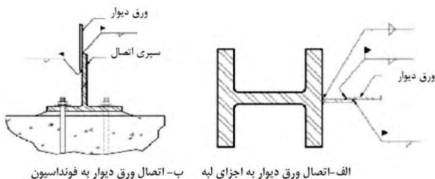
شکل 6-6- نمونه ای از اتصالات ورق دیوار
