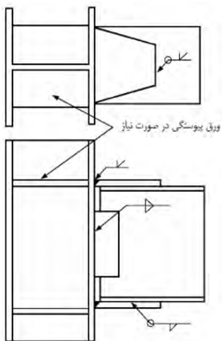
شکل 3-6- اتصال ورق به بال تیر با جوش
