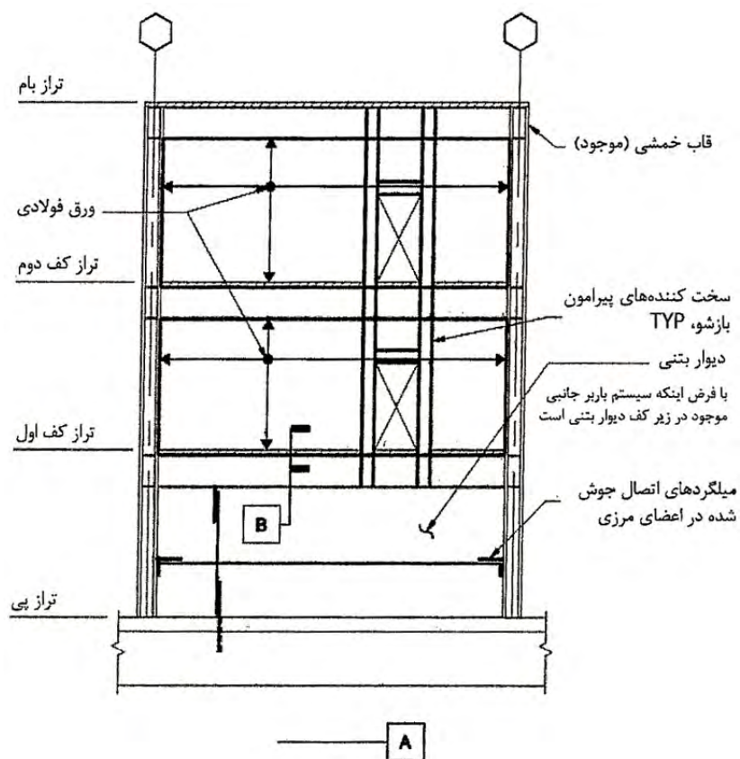
شکل 7-24- دیوار برشی فولادی بدون سخت‌کننده
