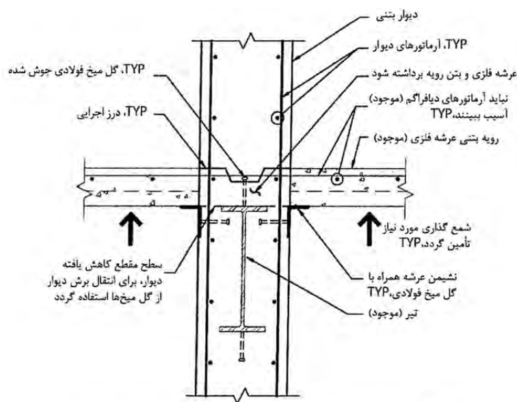
شکل 7-7- دیوار بتنی درجا در محل تیر موجود
