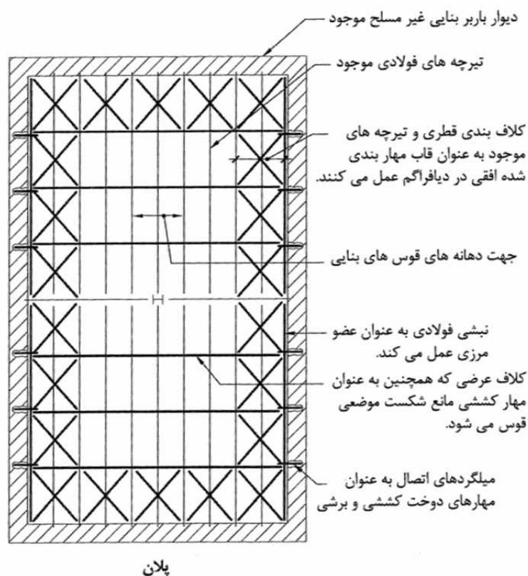
شکل 10-6- مقاوم سازی طاق ضربی
