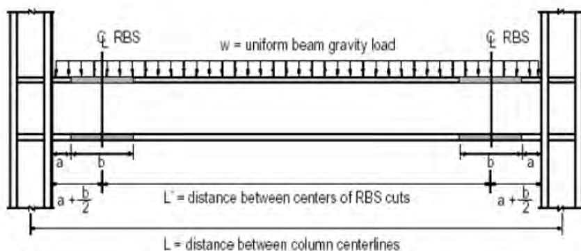
شکل 7-19- مقطع قاب با تیر RBS
