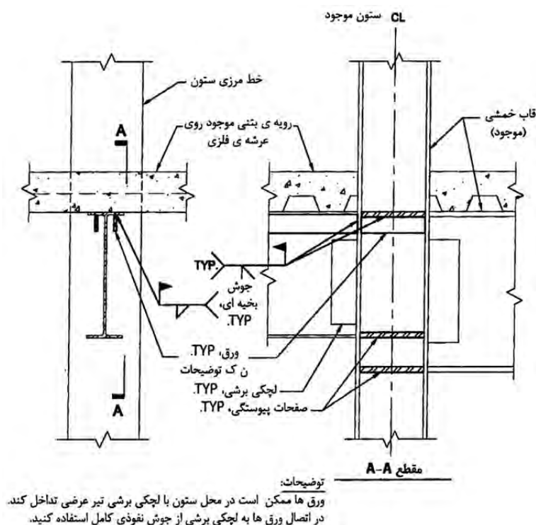
شکل 7-14- استفاده از ورق بعنوان جمع کننده در محل تیر موجود
