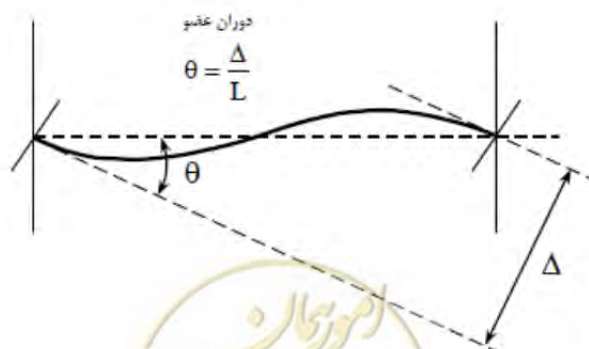
ب - مثال عضوی از یک قاب شکل 2-6- تعریف چرخش عضو
