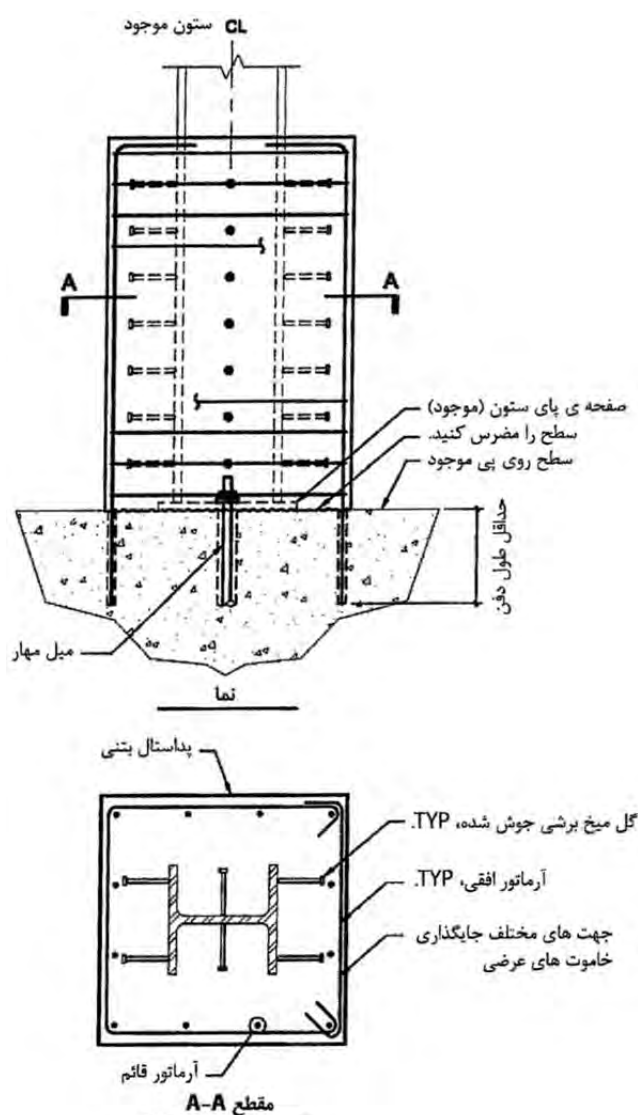
شکل 7-16- پداستال بتنی در محل ستون موجود
