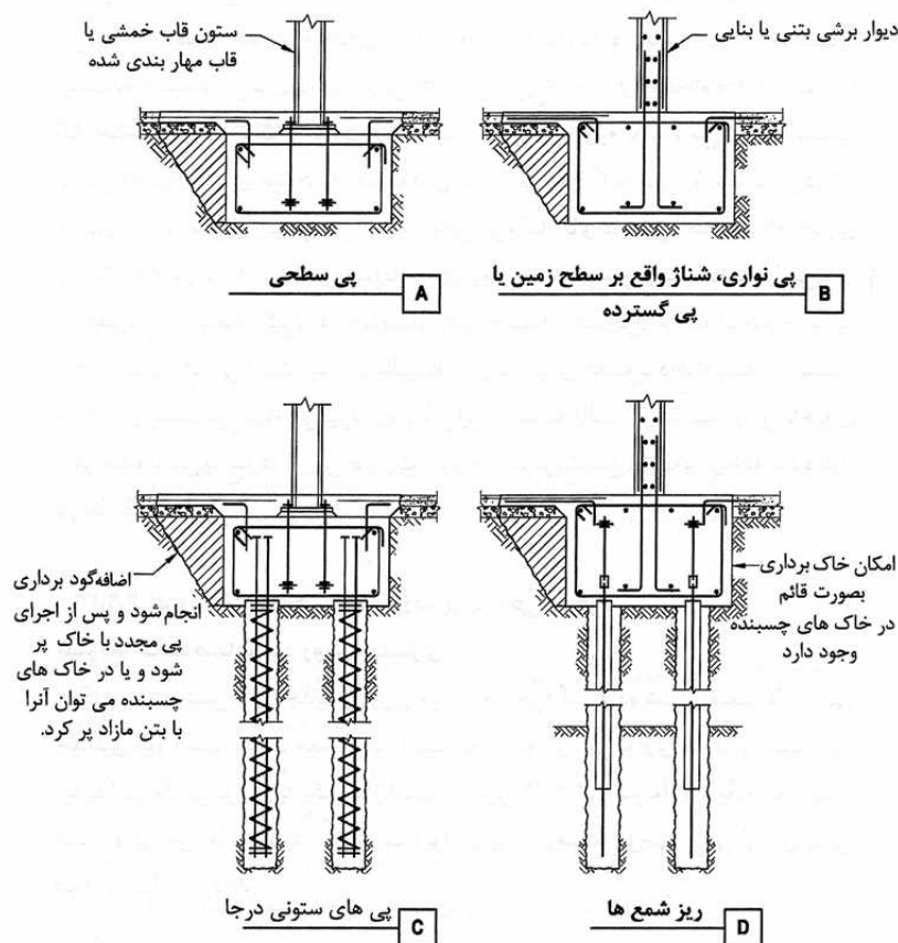
شکل 11-1- انواع پی‌های متداول در بهسازی لرزه ای
