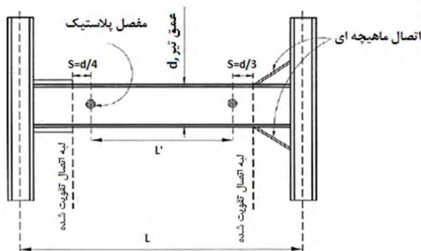
شکل 7-21- نمونه محل تشکیل مفاصل پلاستیک
