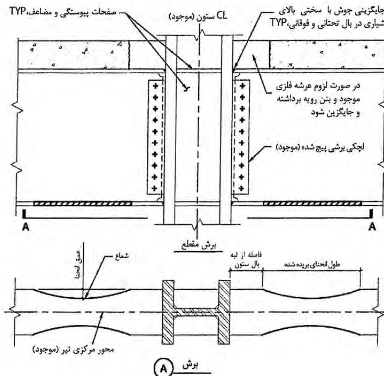
شکل 7-17- مقطع تیر کاهش یافته در بال تحتانی تیر موجود
