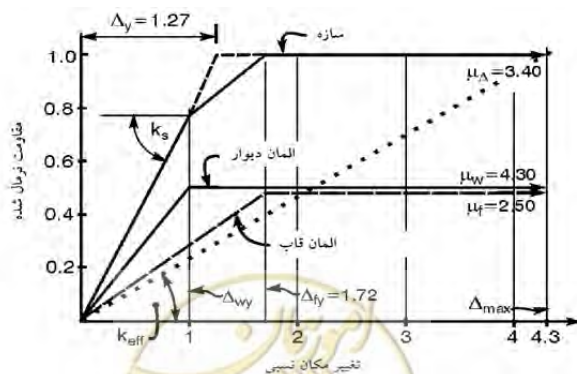
شکل الف-9- مدلسازی دوخطی از رفتار نیرو- تغییرمکان سیستم دوگانه
