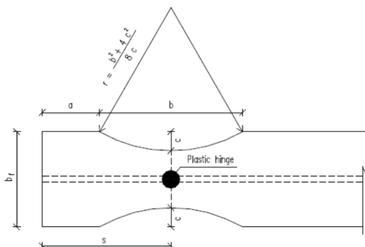
شکل 7-18- هندسه تیر RBS
