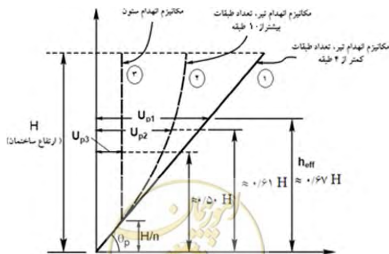
شکل الف-5- نمودار تغییر مکان غیرارتنجایی قابها
