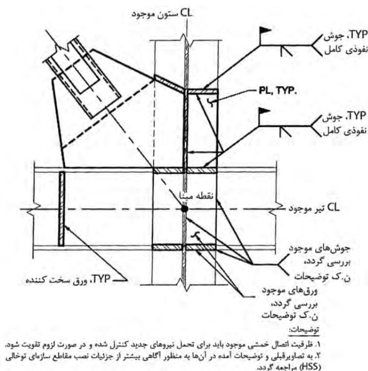
شکل 5-7- مه‌ار بند ساخته شده از مقاطع سازه ای توخالی در اتصال تیر به ستون موجود
