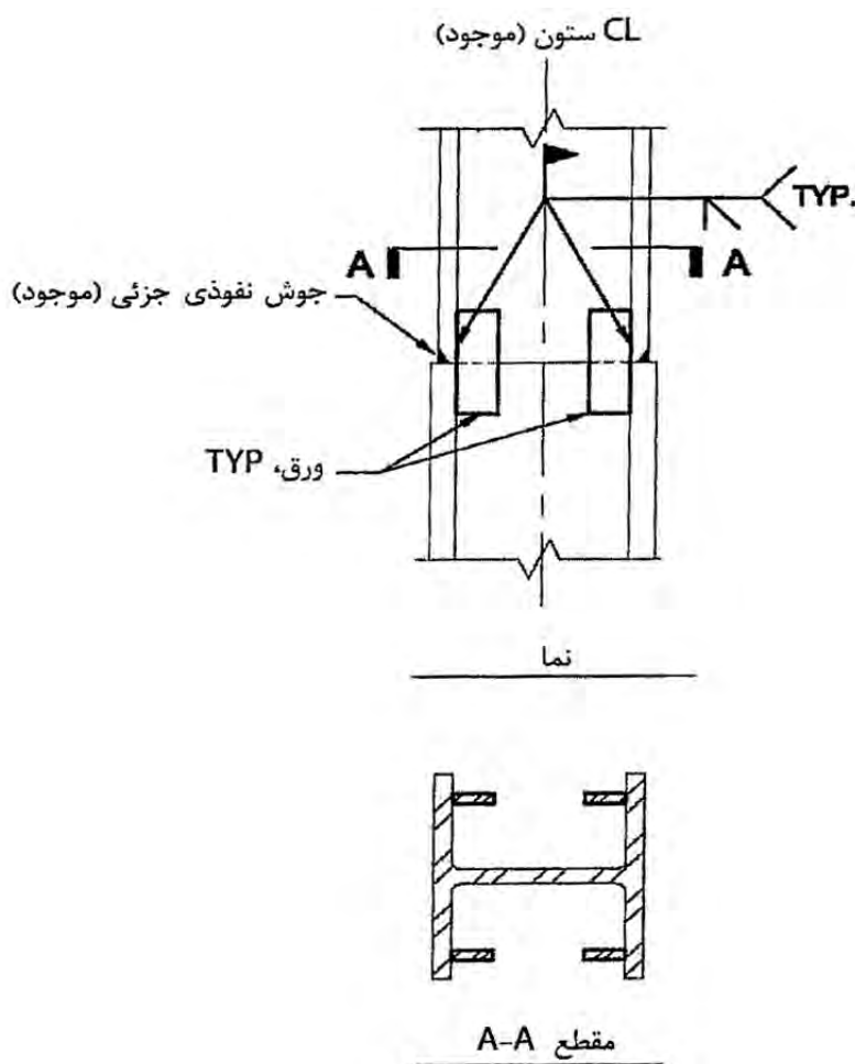
شکل 7-22- بهسازی وصله جوشی در ستون موجود
