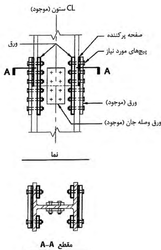
شکل 7-23- بهسازی وصله پیچی در ستون موجود
