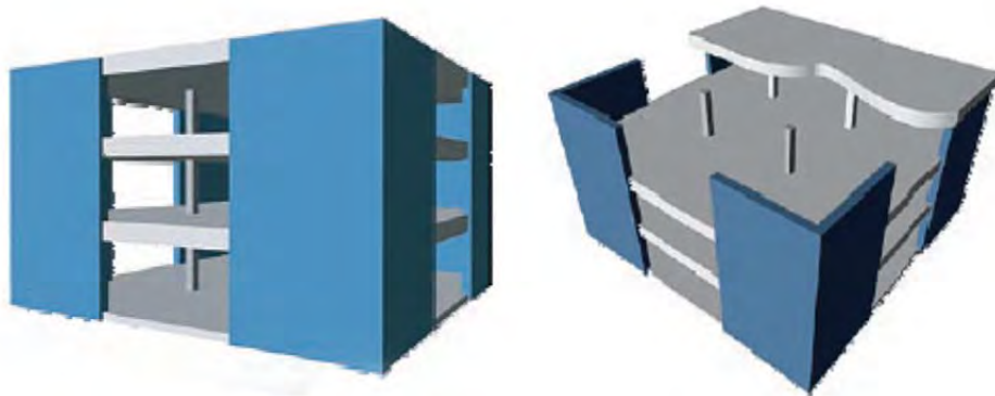
شکل 7-6- بهسازی لرزه‌ای قاب‌های موجود بوسیله افزودن دیوارهای برشی
