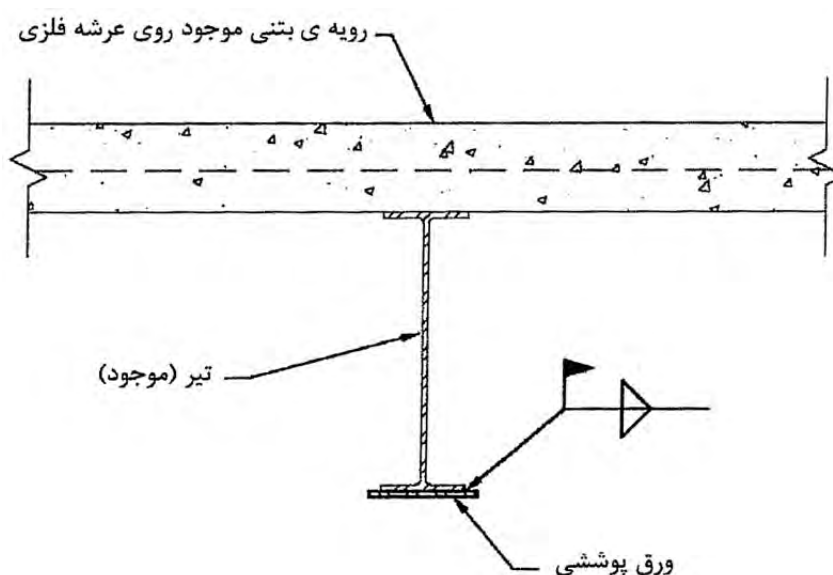
شکل 7-12- استفاده از ورق پوششی (تقویتی) در تیر موجود
