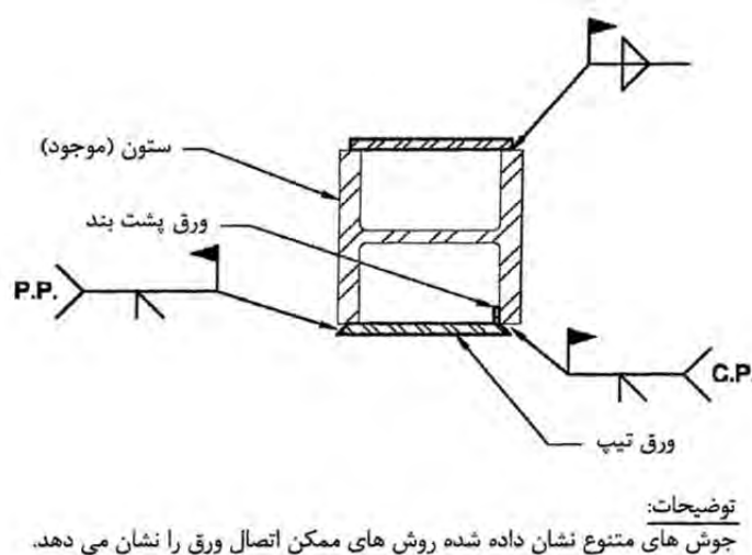
شکل 7-13- تبدیل مقطع ستون موجود به قوطی
