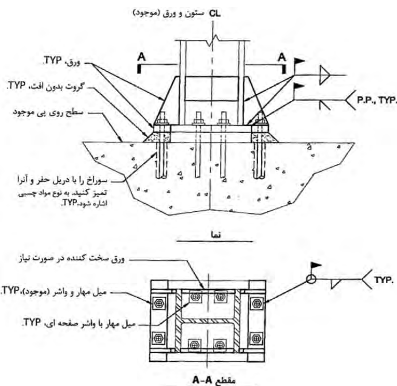
شکل 7-15- افزایش ظرفیت بلند شدگی در پای ستون
