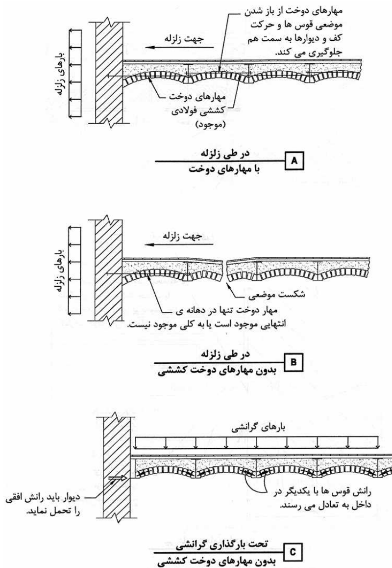
شکل 10-3- انواع شکست در طاق‌های ضربی
