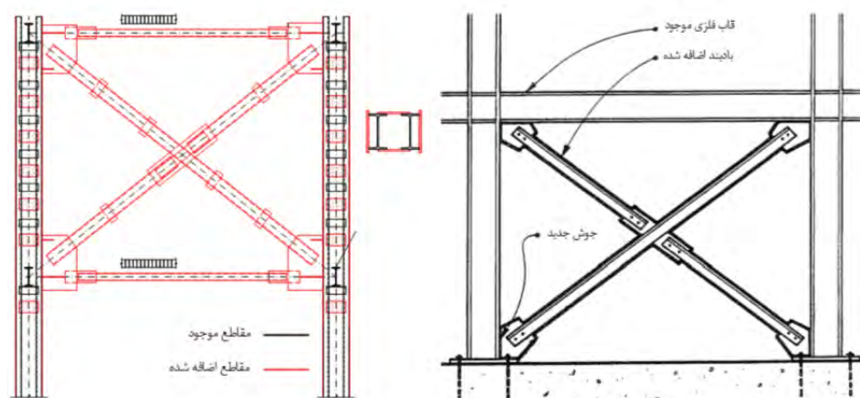
شکل 2-7- بهسازی لرزه‌ای قابهای موجود بوسیله افزودن مهاربندهای همگرا
