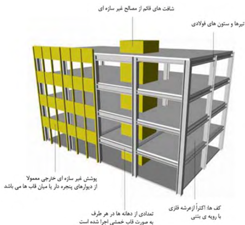
شکل 1-7- نمونه‌ای از قابهای خمشی فولادی
