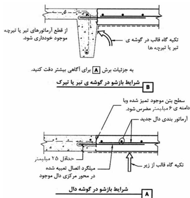
شکل 10-1- پر کردن بازشو در دیافراگم بتنی
