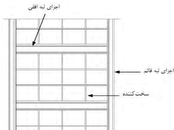
شکل 6-5- نمای دیوار برشی فولادی سخت شده
