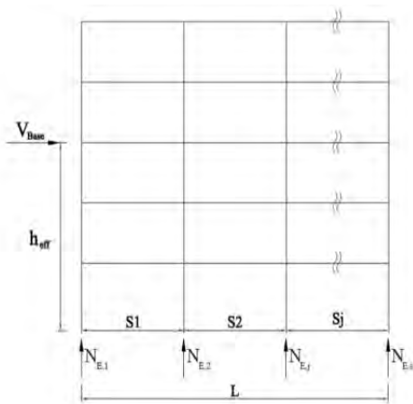
شکل الف-6- نیروی محوری ناشی از زلزله در پای ستونهای
