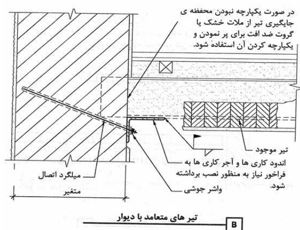
شکل 10-4- افزودن مهارهای دوخت و عضو مرزی دیوار به دیافراگم طاق ضربی - در صورت دسترسی از زیر کف
