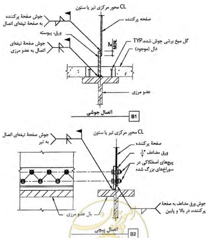
شکل 7-25- اتصال دیوار برشی با صفحه تیغه
