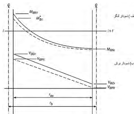
شکل الف-1- برش تیرها
