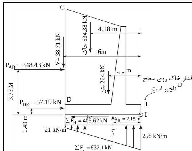
شکل ۹-۸- محاسبات پایداری
