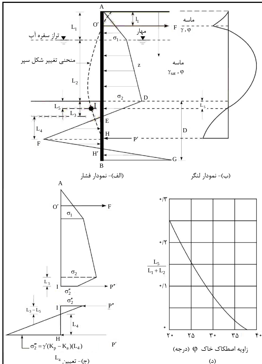
شکل ۱۹-۱۰- روش پای‌گیردار برای سپر کوبیده شده در ماسه
