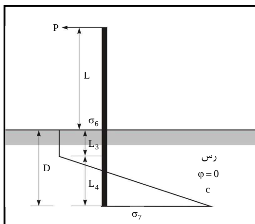
شکل ۱۰-۱۲- سپر طره‌ای کوبیده شده در خاک رسی با بار خطی در بالای سپر
