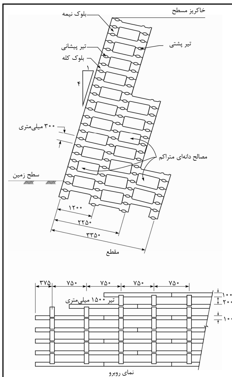
شکل ۱۱-۷- نمونه‌ای از دیوار صندوقه‌ای با تیرهای پیش‌ساخته‌ی بتنی (دیوار Criblock)
