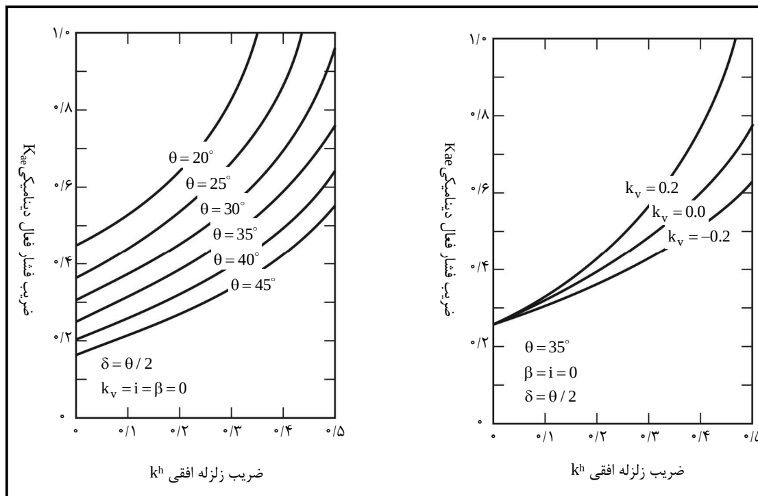
شکل ۱۴-۲- اثر ضریب زلزله و زاویه اصطکاک خاک بر ضریب فشار فعال لرزه‌ای
