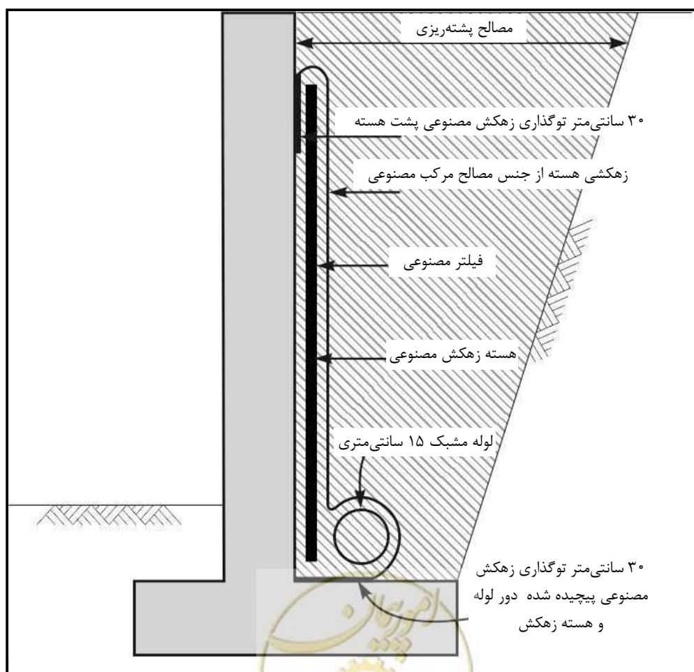
شکل ۶-۶- سیستم زهکش مصنوعی مرکب قائم (در مجاورت دیوار)
