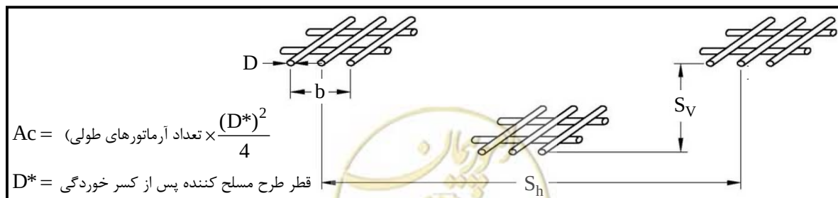
شکل ۱۳-۱۸- معرفی مشخصه های مسلح کننده های شبکه ای
