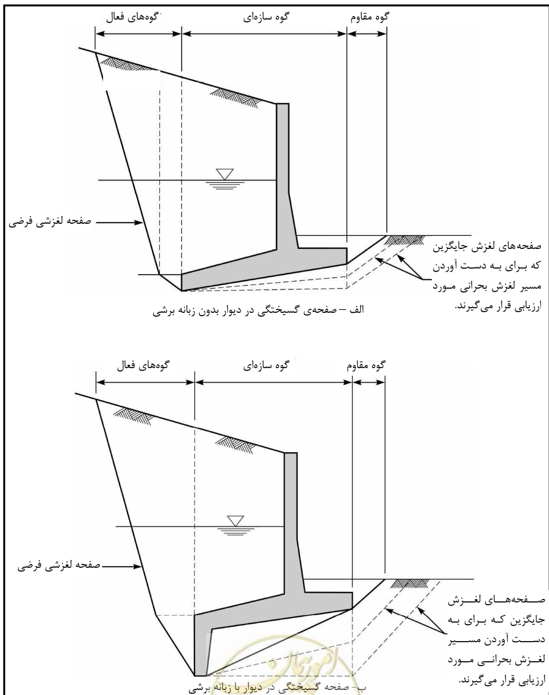
شکل ۸-۴ - سیستم کلی سازه - خاک با یک صفحه‌ی گسیختگی فرضی
