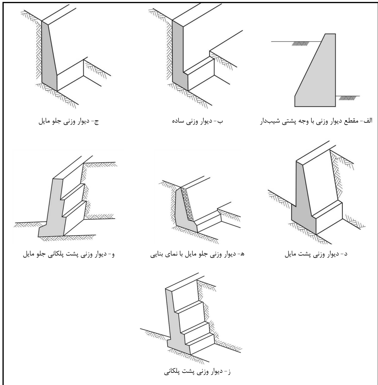
شکل ۱-۲- دیوارهای حایل صلب، دیوارهای حایل وزنی
