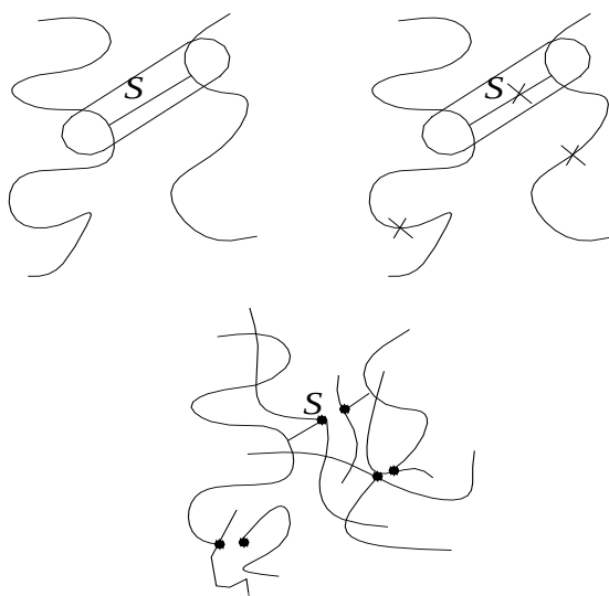
شکل ۲-۴- اثر اکسیداسیون بر روی مولکول‌های لاستیک
