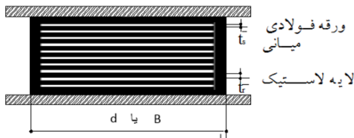
شکل ۵-۳- مقطع جداساز لاستیکی با ورق‌های فولادی
