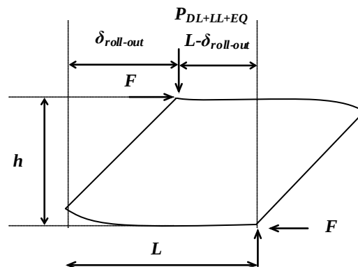
شکل ۳-۸- نمایش عامل‌های مورد نیاز در کنترل چرخش جداساز
