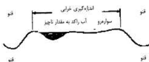
شکل ۹۷ سطوح شدت مقطع عرضی نامناسب.
