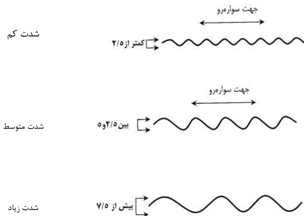
شکل ۹۳ سطوح شدت خرابی چین خوردگی.
