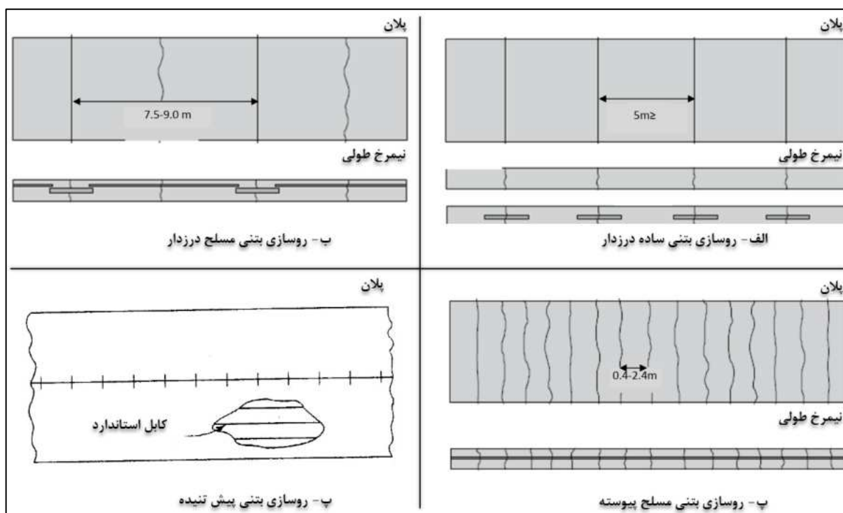
شکل ۲ چهار نوع اصلی روسازی بتنی
