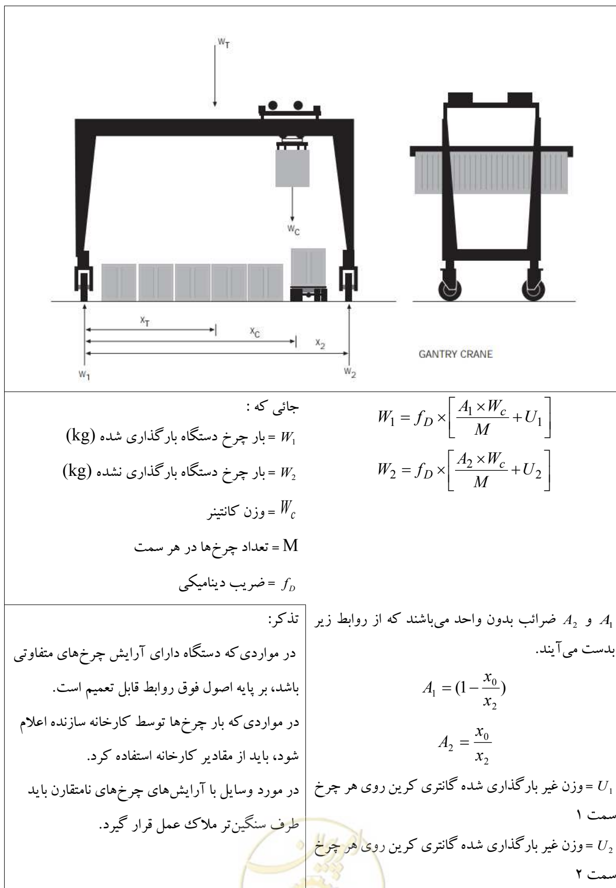
شکل ۳۱ نحوه محاسبه بار چرخ گانتري کرین
