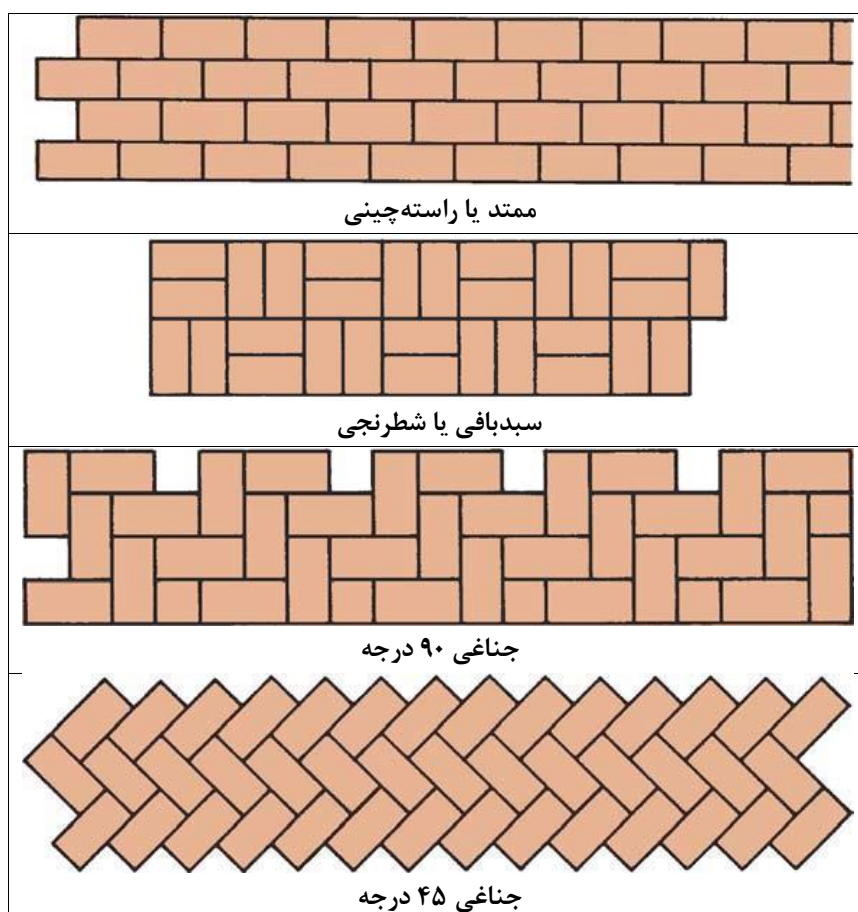
شکل ۱۲ انواع چیدمان بلوک‌های مستطیلی
