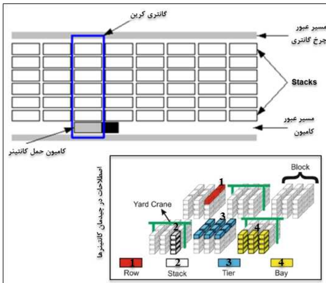
شکل ۸ تکرار بارگذاری در محوطه کانتینری - گانتی کرین و اصطلاحات در چیدمان کانتینرها
