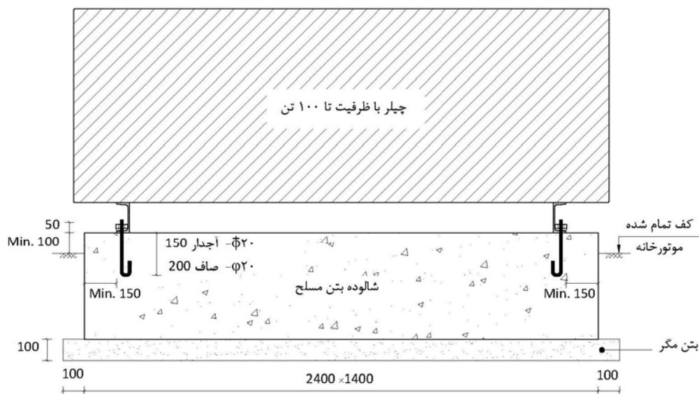
SEC. a-a
