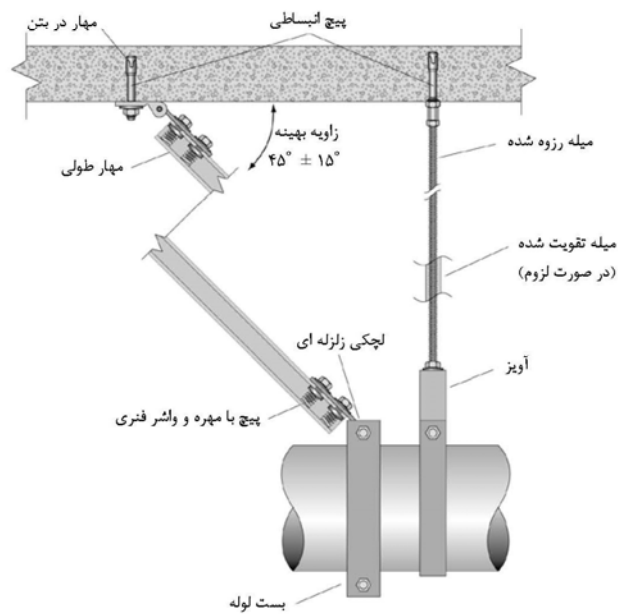
مهر طولی یک در میان
