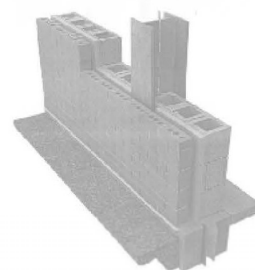
جزئیات اتصال دیوار نما به پدنه دیوار بنایی
