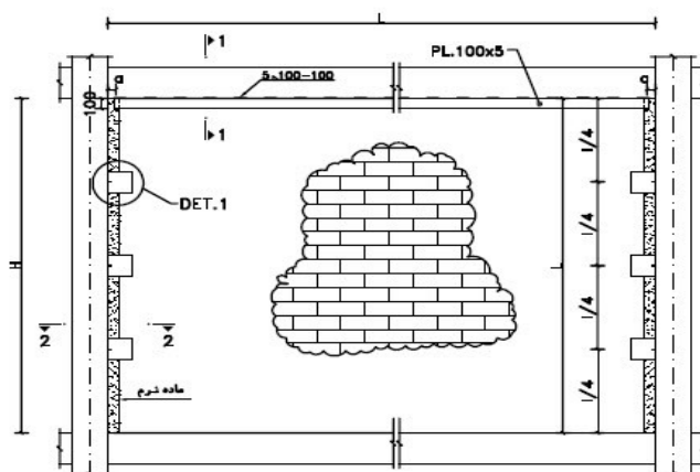
تیغه نوع سبک (نظیر سیپورکس) S.C.: 1/90 TYP. 4
