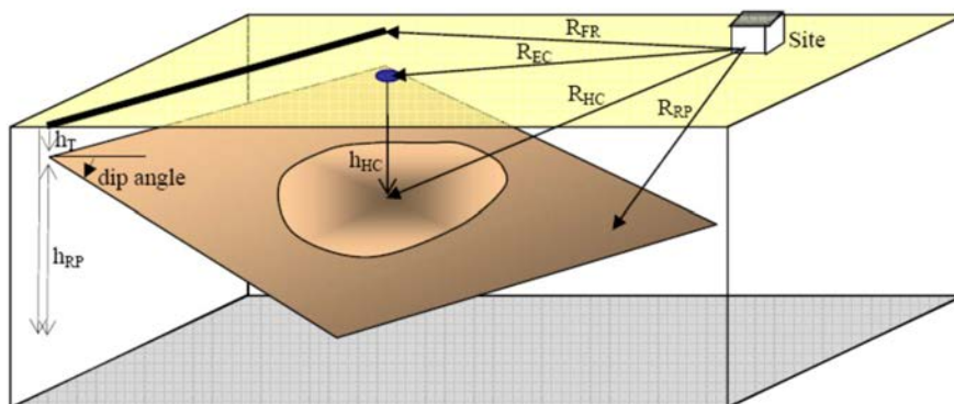
۱۷-۴- تعاریف مختلف فاصله منبع تا سایت به کار رفته در روابط کاهندگی (ذوالفقاری، ۲۰۰۹)
