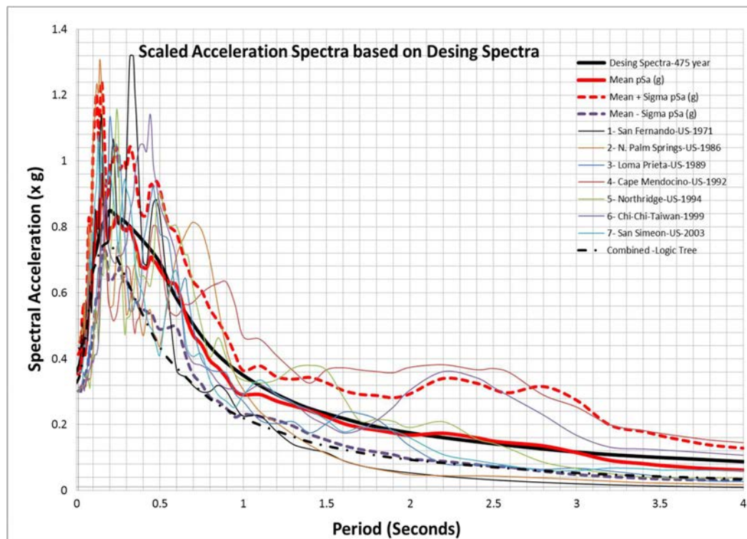
شکل ۴-۲۶- مقیاسه طیف‌های پاسخ یک درجه آزادی رکوردهای انتخابی و طیف پاسخ طراحی. مقادیر میانه و صدک ۱۶ و ۸۴ نیز در
