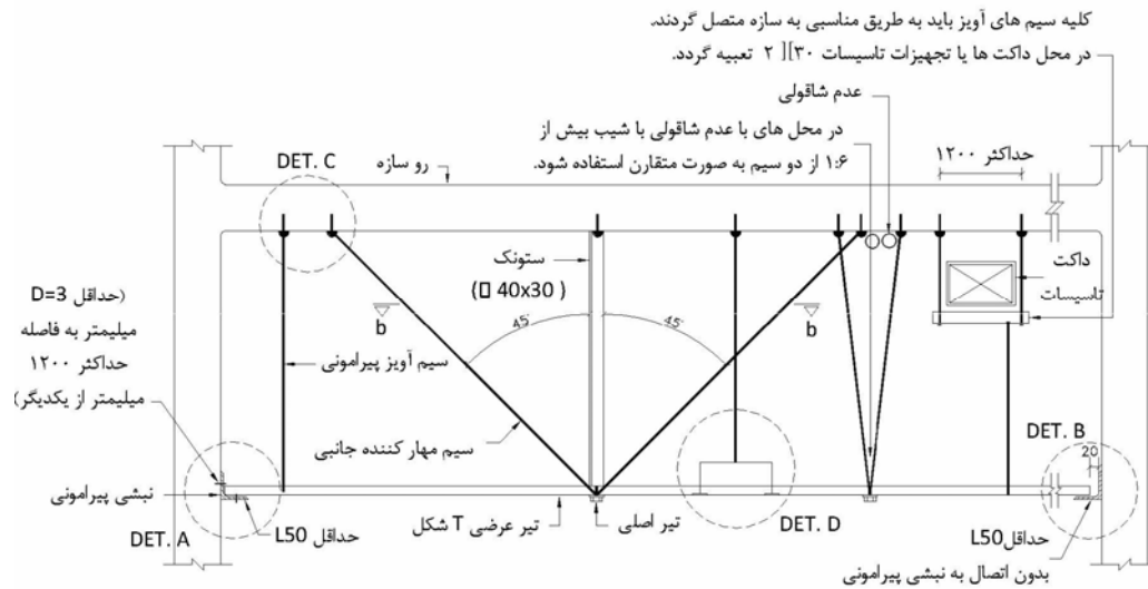
سقف کاذب معلق با مهار جانبی (مقطع عرضی)
