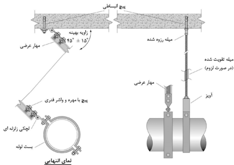
مهر عرضی یک در میان
