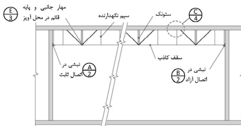
SEC. a-a
