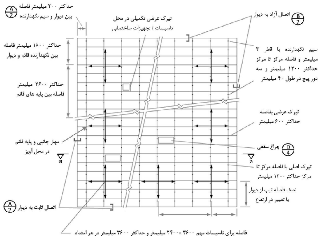
بلان سقف کاذب
