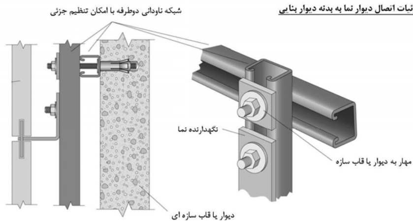
جزئیات اتصال دیوار نما به پدنه دیوار بنایی
