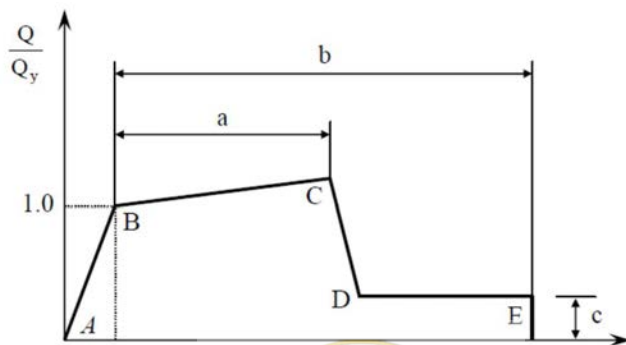
شکل ۱-۲- منحنی ساده شده نیرو-تغییر شکل اعضاء
