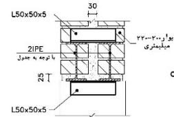
جزئیات اتصال به تیر یا کلاف بتنی S.C.: 1/10
