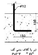
جزئیات اتصال به تیر یا کلاف بتنی S.C.: 1/10
