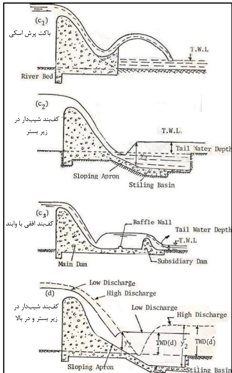
شکل ۴-۱۴- انواع توصیه فنی برای وضعیت‌های مختلف TW و y_2
