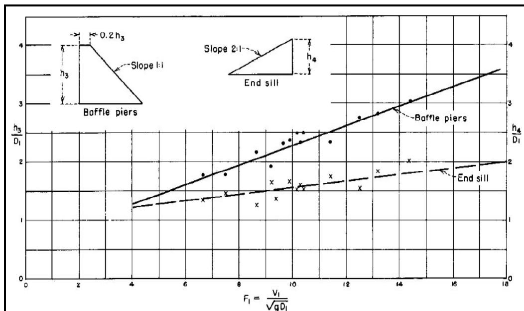
شکل ۴-۳- ارتفاع دیوار آرام کننده و آستانه انتهایی بر حسب F_1 و D_1 در حوضچه‌های نوع III و IV (U.S.B.R)
