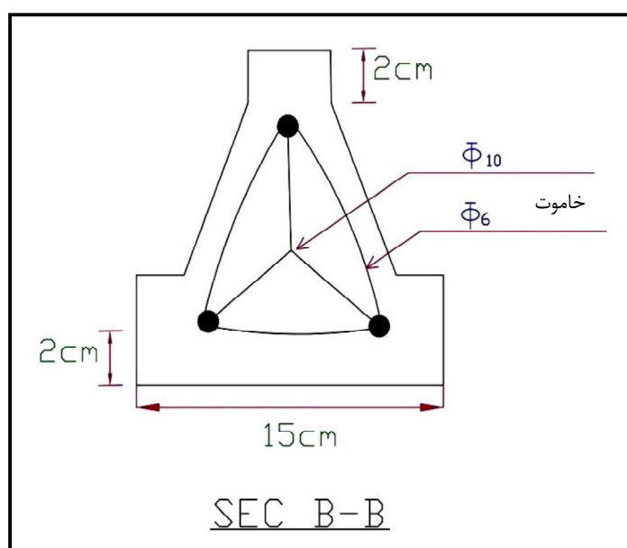
شکل ۶-۲- برش های A-A و B-B از بند پایه بتنی
