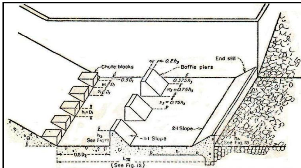
شکل ۴-۱۸- حوضچه آرامش نوع III (U.S.B.R.)
