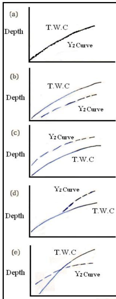
شکل ۴-۱۲- وضعیت T.W. و y_2 نسبت به یکدیگر
