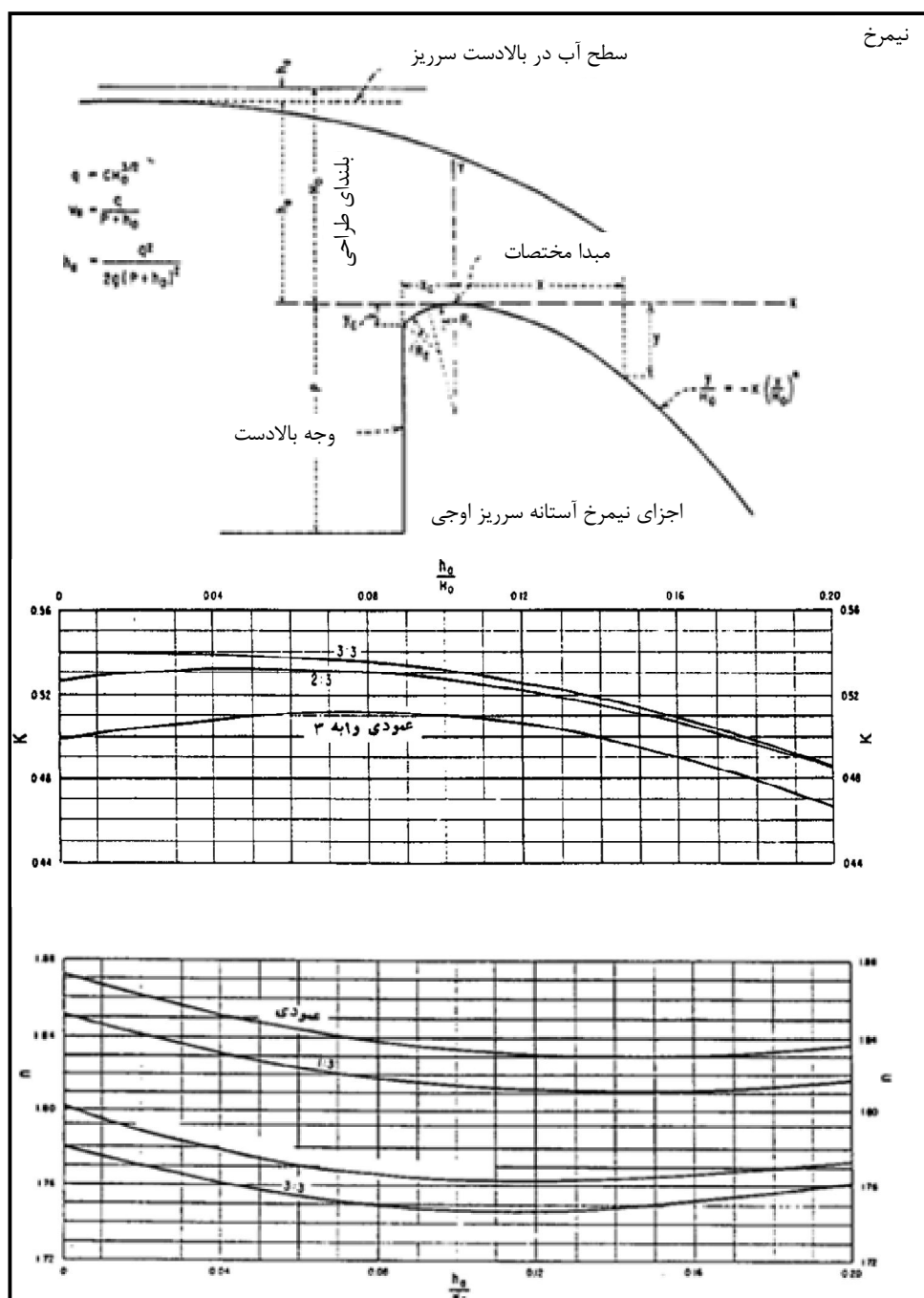
شکل ۴-۲۵- فاکتورهای تعریف پروفیل‌های تاج به شکل سرفه زیرین آب (nappe)
