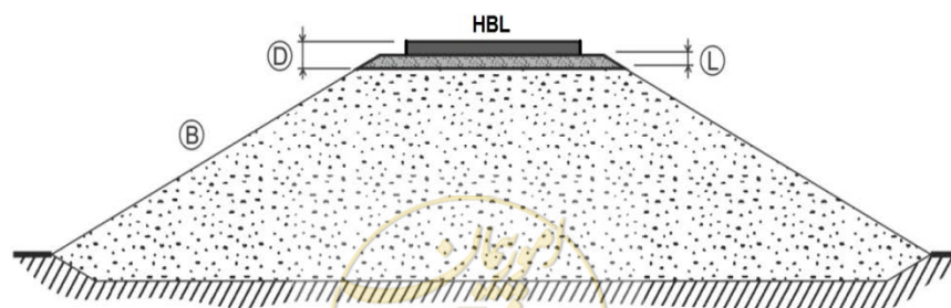
شکل ۵-۴- ساختار و بخش‌های تشکیل دهنده زیرسازی خاکی خطوط بتنی
