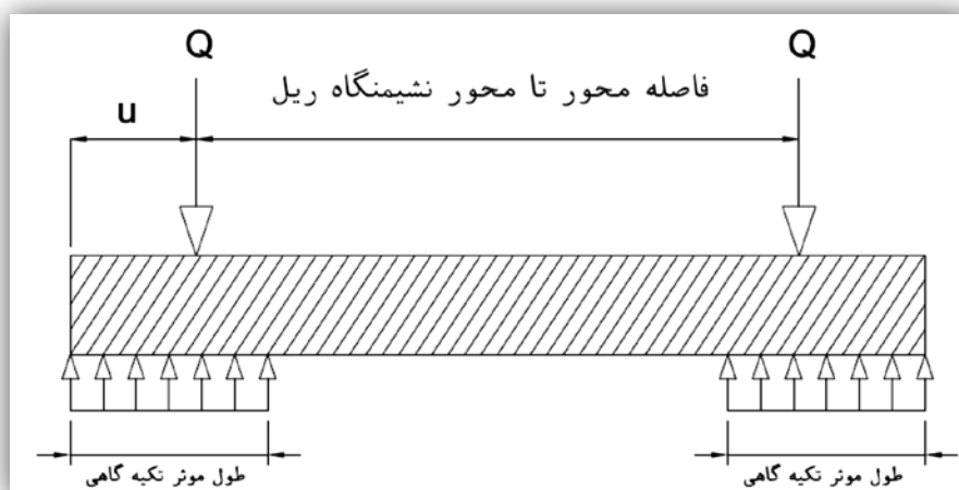
شکل ۱۰-۶- ناحیه موثر تکیه گاهی در دو انتهای تراورس
