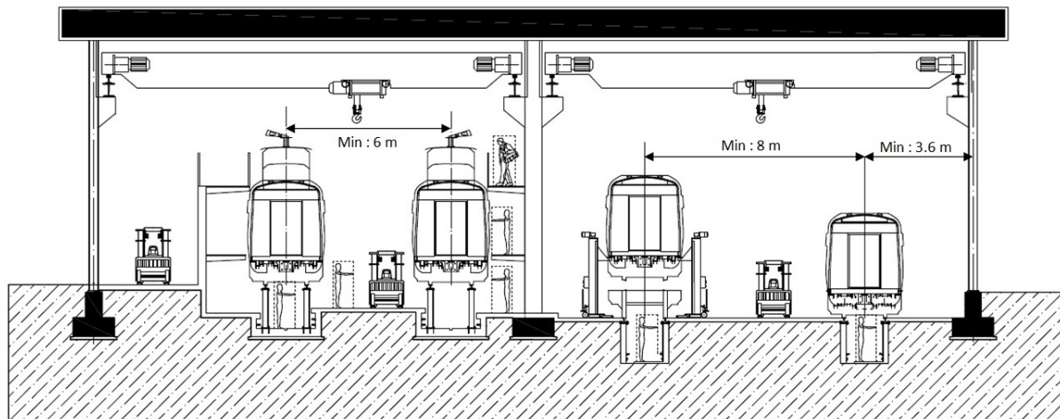
شکل ۱۱-۲- حداقل فواصل عرضی ساختمان تعمیرات
