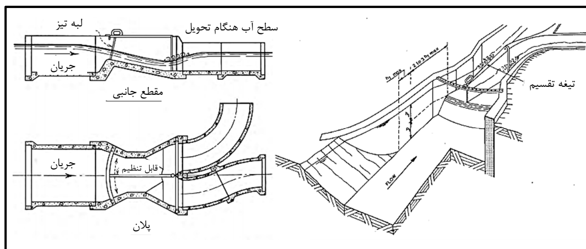
شکل ۴-۳۹- مقسم قابل تنظیم
