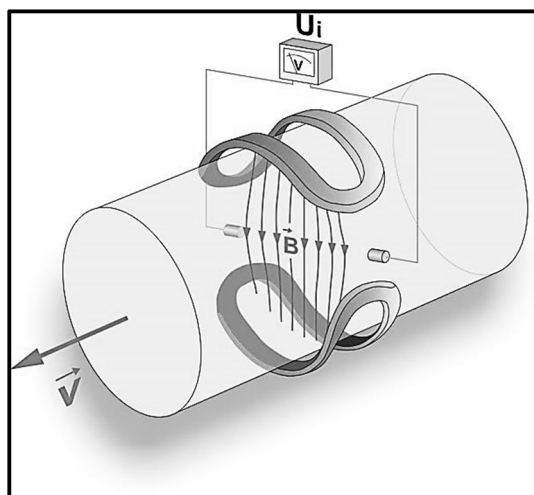
شکل ۵-۸- نمایی از جریان‌سنج الکترومغناطیسی
