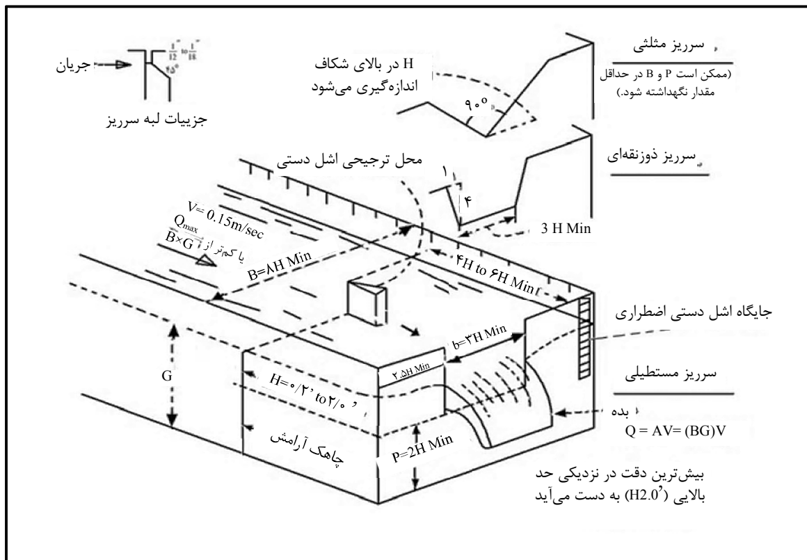
شکل ۹-۲- نسبت‌های استاندارد، برای سرریزهای مستطیلی، سیپولتی، مثلثی ۹۰ درجه
