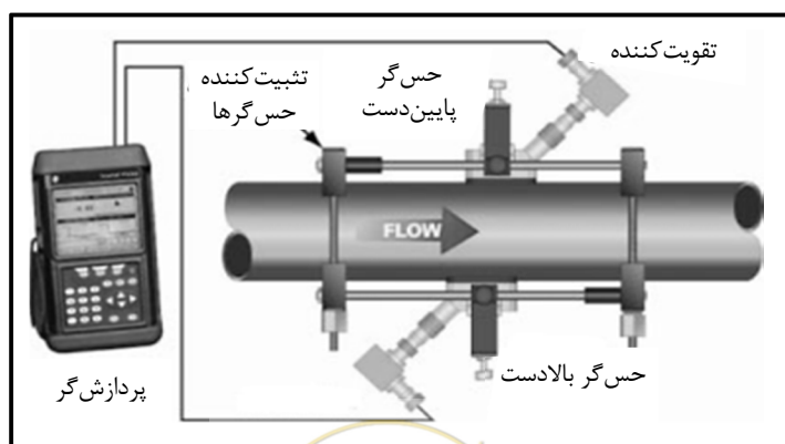
شکل ۶-۵- نمایی از تجهیزات نصب یک جریان‌سنج زمان-گذر فراصوتی
