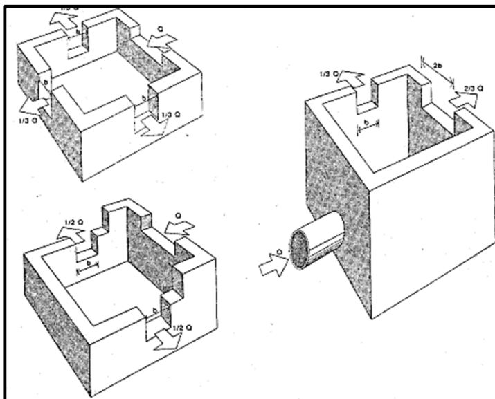
شکل ۴-۳۸- مقسم ثابت
