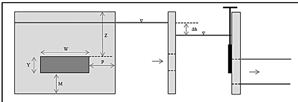
شکل ۴-۳- ابعاد روزنه مستطیلی کاملاً مستغرق انقباضی
