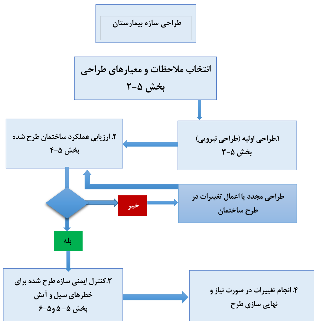
شکل ۵-۱ مراحل طراحی ساختمان بیمارستان
