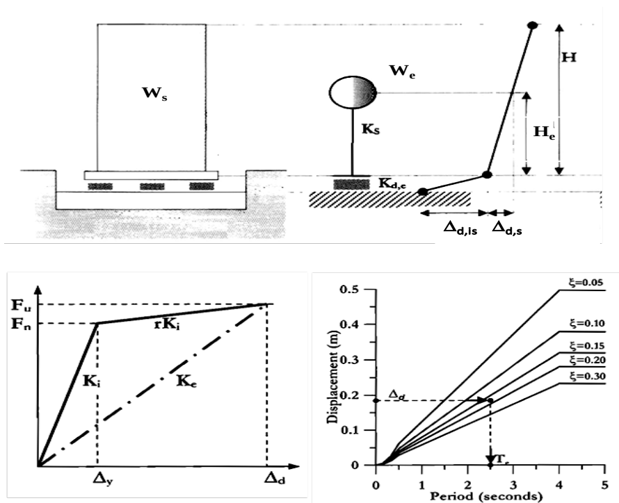
شکل ۶-۱ اصول روش مستقیم طراحی بر اساس تغییرمکان سازه جداسازی شده لرزه‌ای [۲۹]
