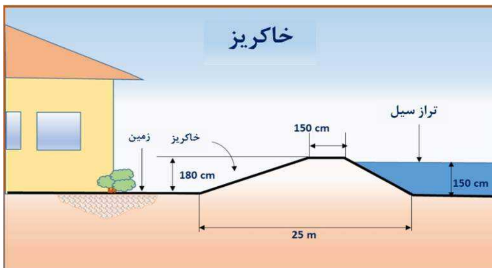
شکل ۵-۶ طرح شماتیک خاکریز متداول برای حفاظت بیمارستان در برابر سیل
