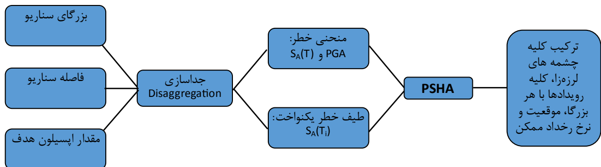
شکل ۳-۴ فرایند تحلیل تفکیک خطر زلزله برای آوردن سناریوی زلزله مبتنی بر تحلیل احتمالاتی زلزله
