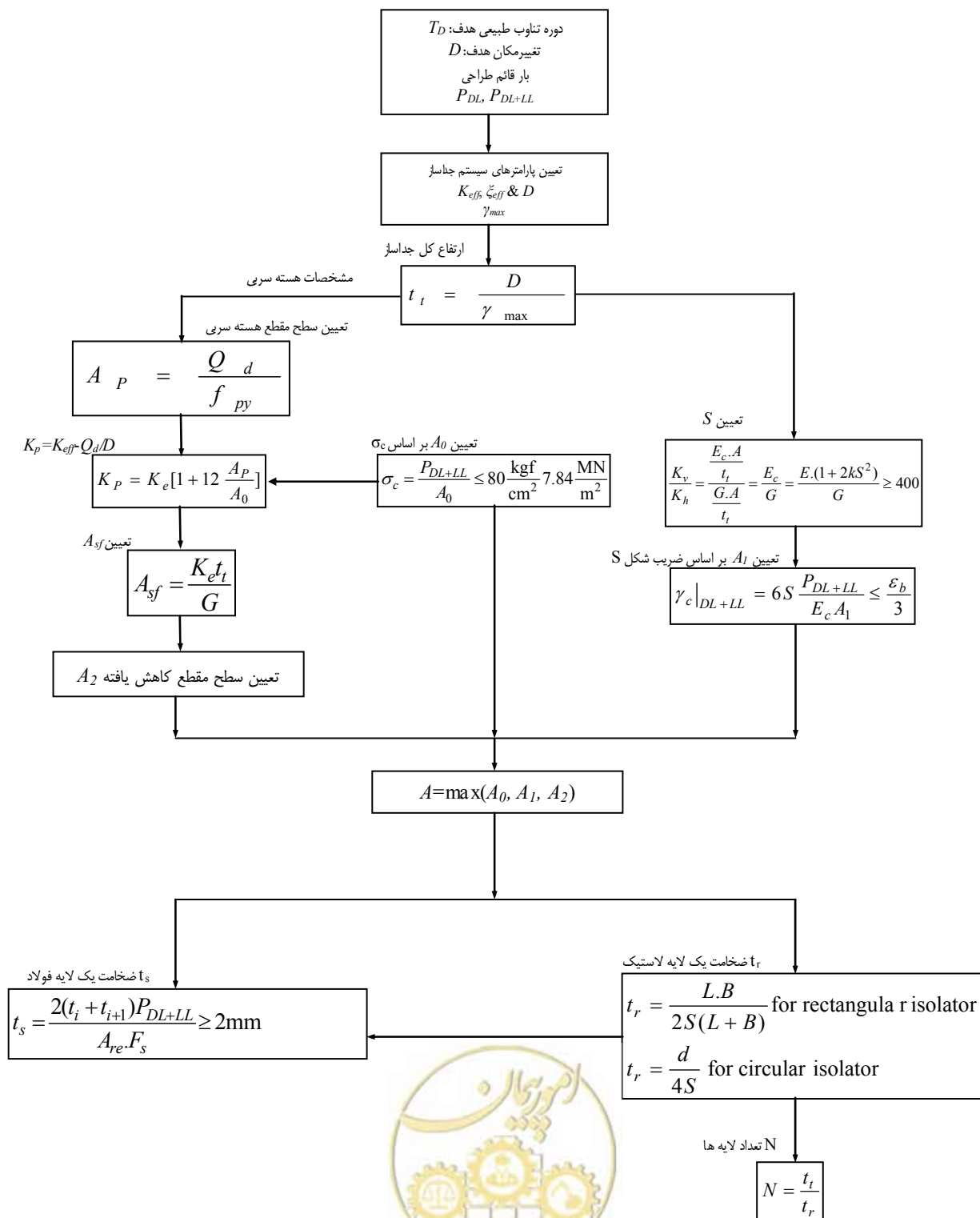
شکل ۳-۹- نمودار طراحی جداساز لاستیکی با هسته‌ی سری
