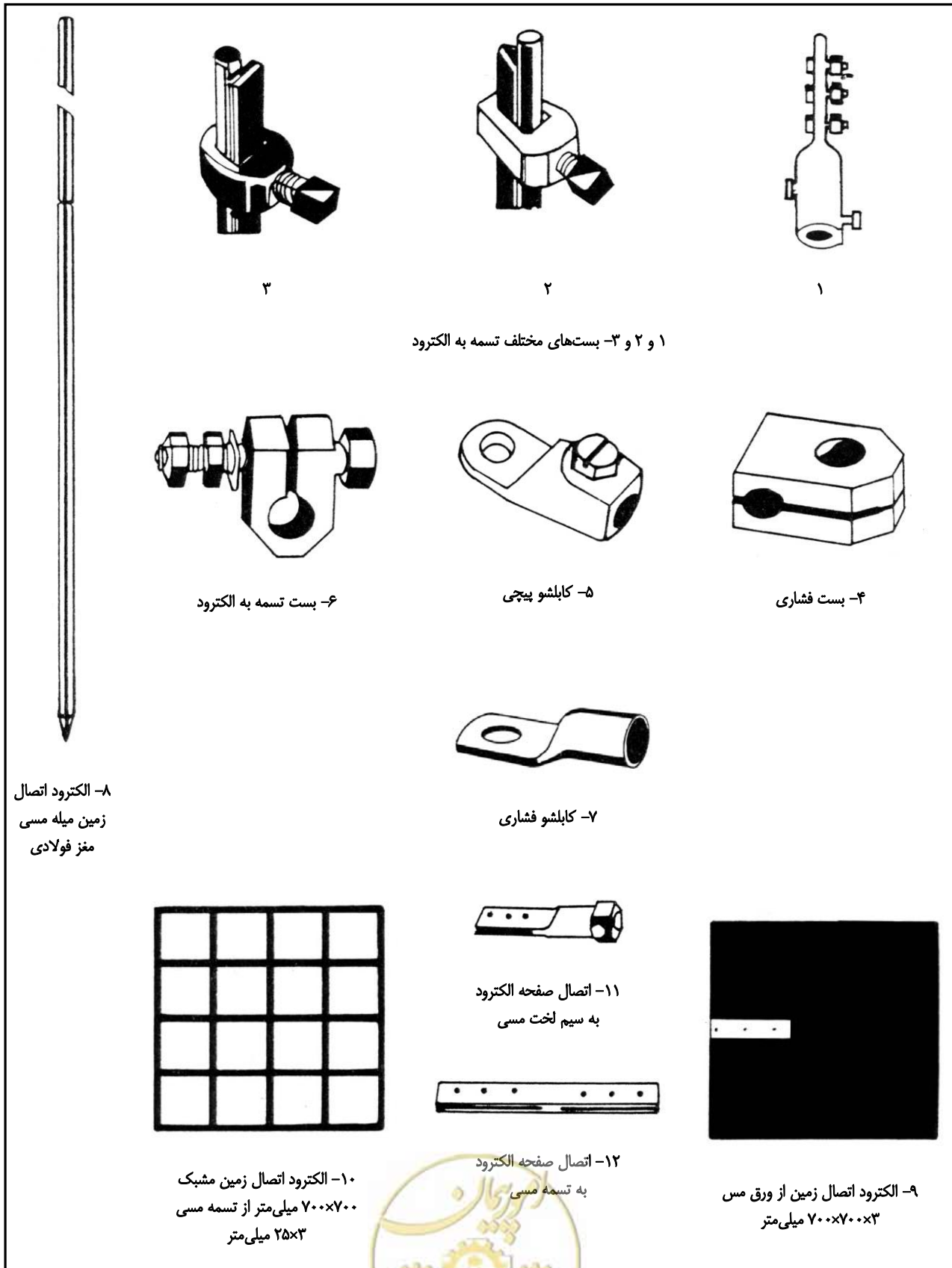
شکل ۱۵-۴: انواع الکترودهای اتصال زمین و بست‌های مربوطه.
