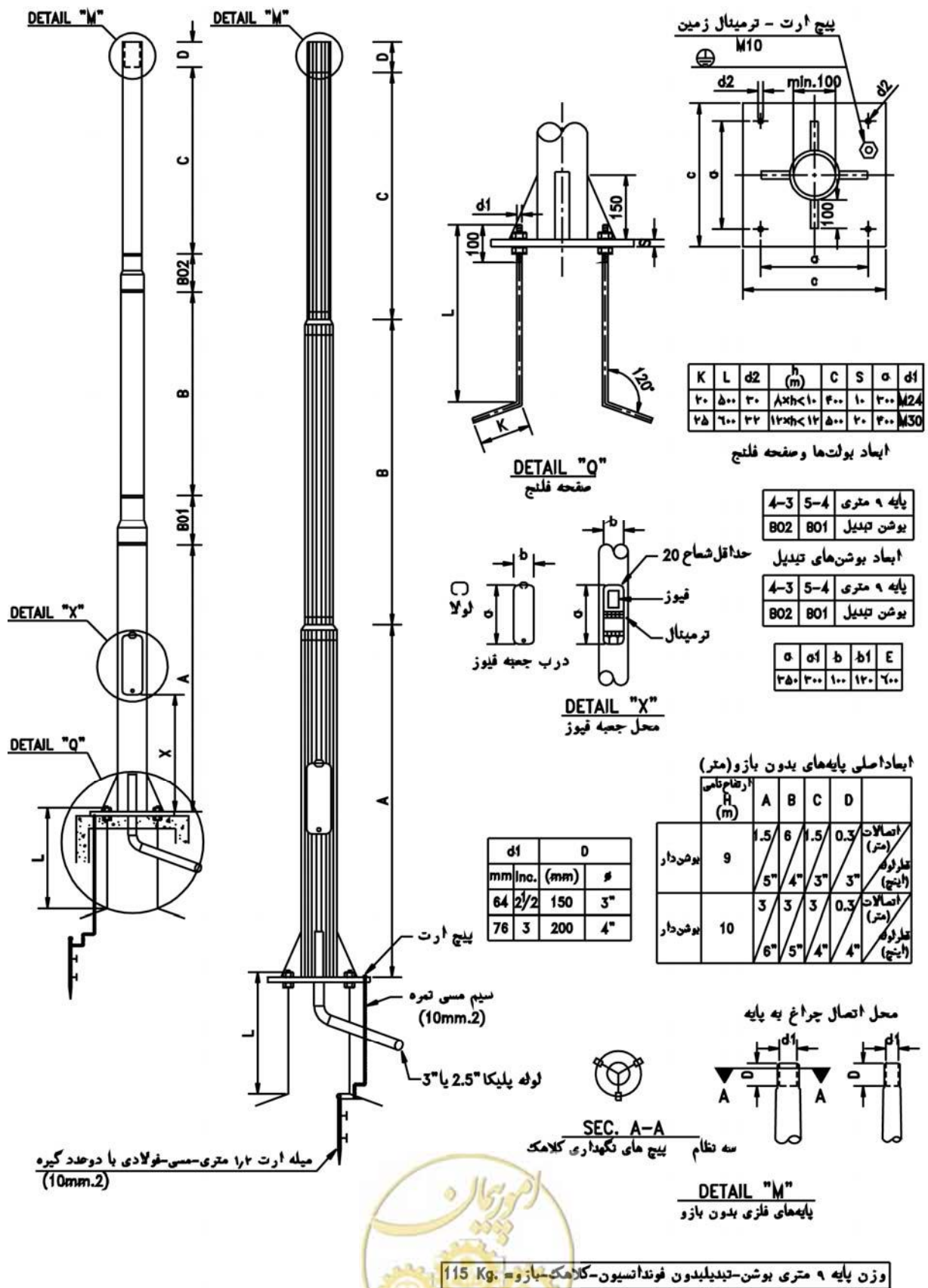
شکل ۱۳-۲: پایه فلزی لوله‌ای، نوع بوشن - تبدیل با صفحه فلنج (۹ و ۱۰ متری)
