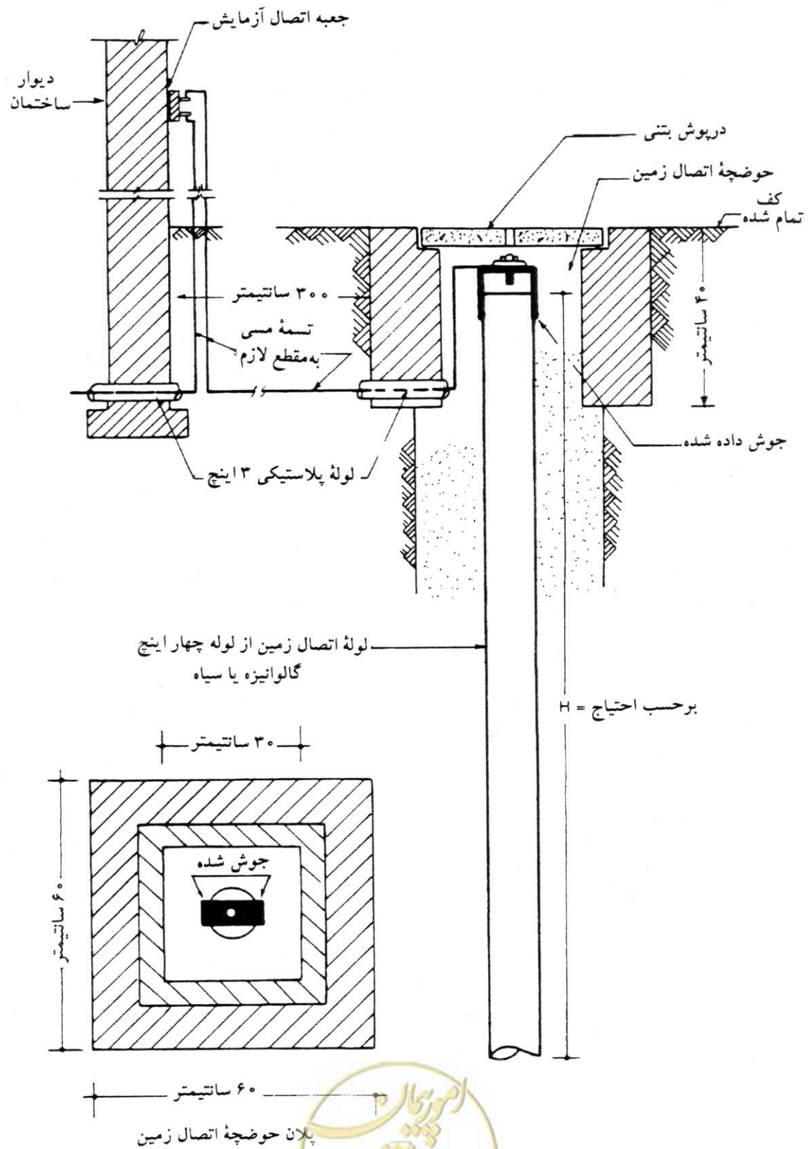
شکل ۱۵-۶: جزئیات نصب سیستم اتصال زمین با الکترو لوله‌ای.
