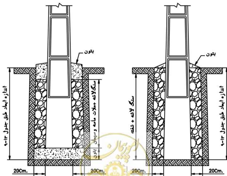
شکل ۱۳-۹: نصب پایه‌های مابانی ۱۳-۱۰: نصب پایه‌های انتهایی، زوایا، و نگهدارنده ترانسفورماتور
