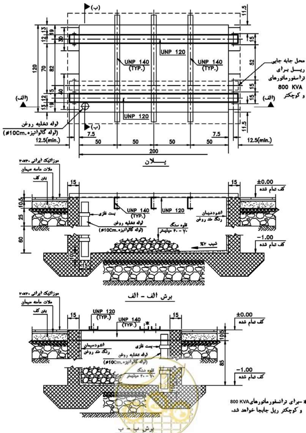
شکل ۱۰-۱: نمونه جزییات حوضچه روغن و ریل گذاری ترانسفورماتور برابر استاندارد وزارت نیرو - امور برق
