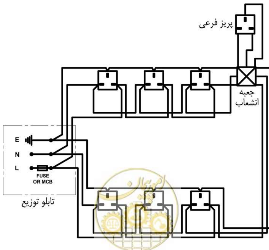
شکل ۳-۲: سیستم سیم‌کشی حلقوی مدار پریزها
