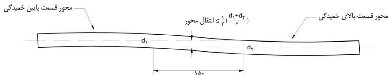
شکل ۵-۱۳: خمیدگی کوتاه تیر، حالت اول
