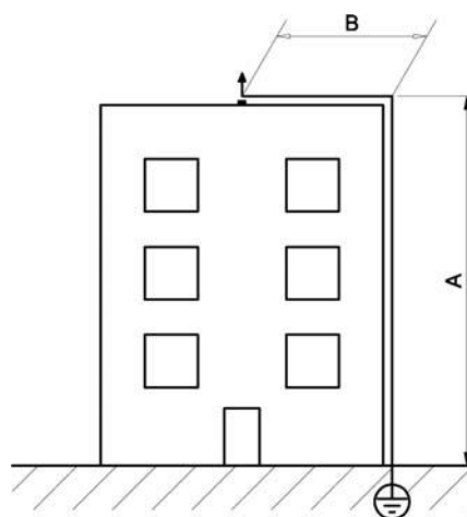
(الف) اتصال پایانه‌های هوایی الکترونیک به یکدیگر با اختلاف سطح حداکثر ۱/۵ متر
