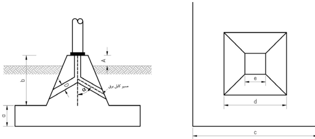
شکل ۱۳-۱۲: نمای نمونه فونداسیون بتنی پیش‌ساخته
