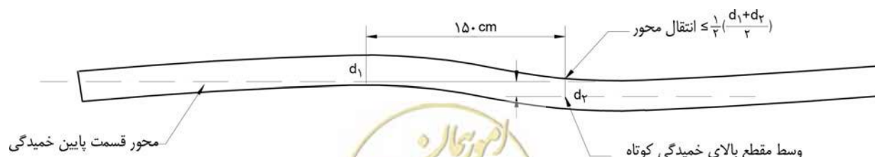
شکل ۷-۱۳: خمیدگی کوتاه تیر، حالت سوم
