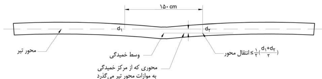
شکل ۶-۱۳: خمیدگی کوتاه تیر، حالت دوم
