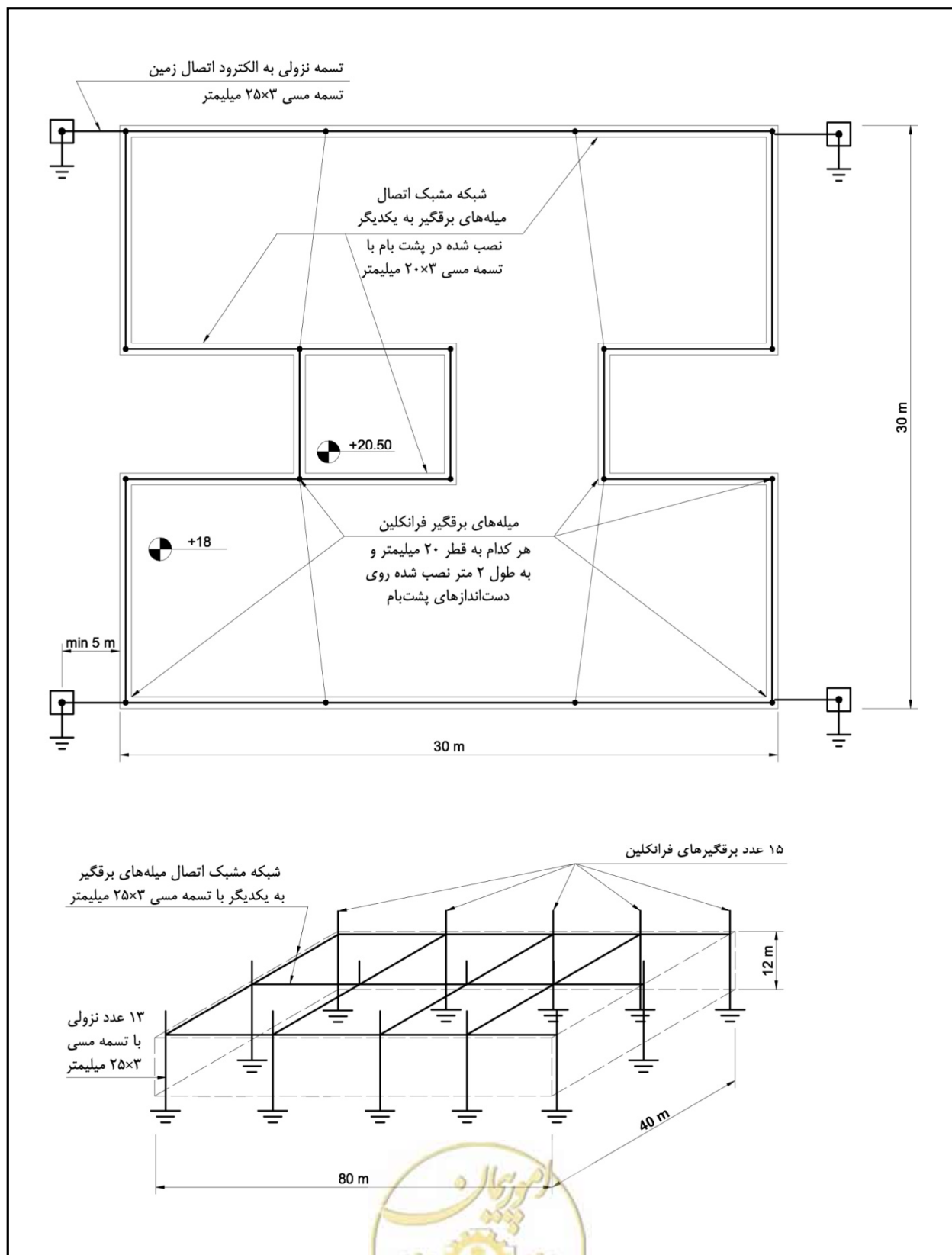
شکل ۱۴-۱۴: نمونه و روش کلی نصب سیستم برقگیر قفس فاراده
