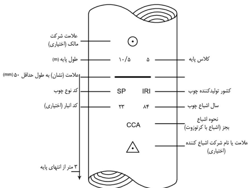
شکل ۸-۱۳: نمونه‌ای از علامت‌گذاری روی پایه‌های چوبی
