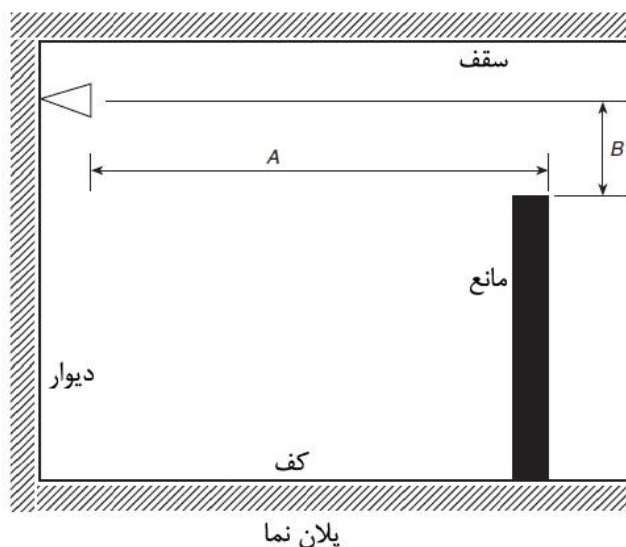
شکل ۸-۷-۵-۲- مانع پایین زن یا قرار گرفته روی زمین (اسپرینکلر دیواری اسپری کننده استاندارد) صرفاً در تصرفات پرخطر
