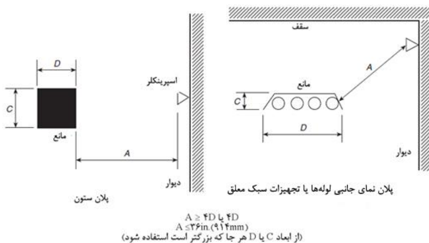
شکل ۸-۹-۵-۲-۱-۴- حداقل فاصله از موانع (اسپیرینکلرهای اسیری کننده دیواری پوشش گسترده)
