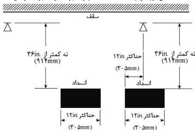
شکل ۸-۱۱-۵-۴ مانع بزرگتر از ۳۶in (۹۱۴mm) زیر اسپرینکلر (اسپرینکرها CMSA)
