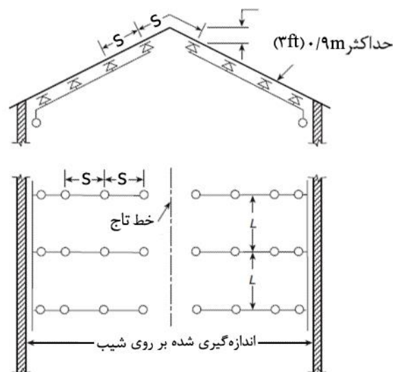
شکل ۸-۶-۴-۱-۳-ب- اسپرینکرها در سقف شیب دار (فاصله تا بام)، شاخه ها در امتداد شیب ها
