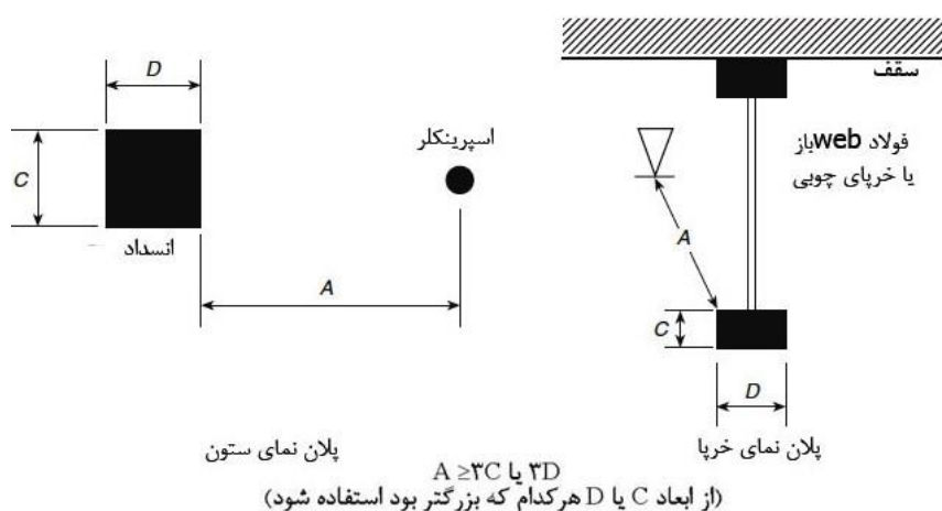
شکل ۸-۱۱-۵-۳-۱ حداقل فاصله از مانع (اسپرینکلرهای CMA)
