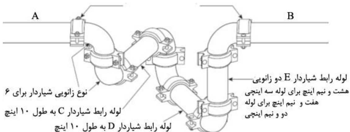
شکل ۹-۳-۴- مجموعه جداساز لرزه‌ای با فاصله جداسازی ۲۰۰mm (۸in) در محل تقاطع لوله‌ها با قطر اسمی تا ۱۰۰mm (۴in). (برای سایر فواصل جداسازی و اندازه لوله‌ها، طول‌ها و فواصل باید متناسباً اصلاح شوند)
