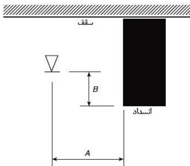
شکل ۸-۱۲-۵-۱ جانمایی اسپرینکلرها از مانع به منظور جلوگیری از تاثیر بر تخلیه آب (اسپرینکلرهای ESFR)
