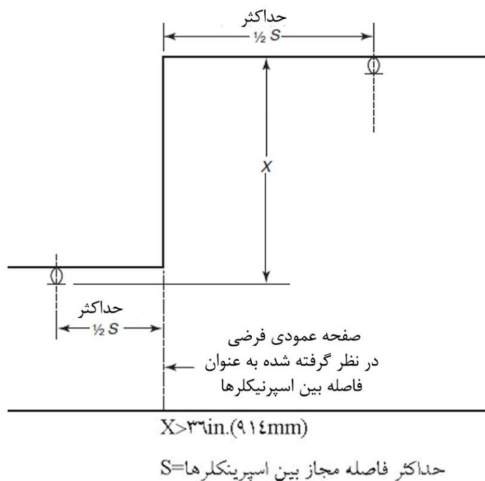
شکل ۸-۶-۴-۱-۳-الف- تغییر عمودی در ارتفاع سقف بزرگتر از 36in. (914mm)
