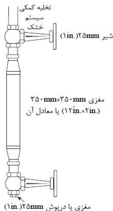
شکل ۸-۱۶-۲-۵-۳-۵- تخلیه کمکی سیستم خشک
