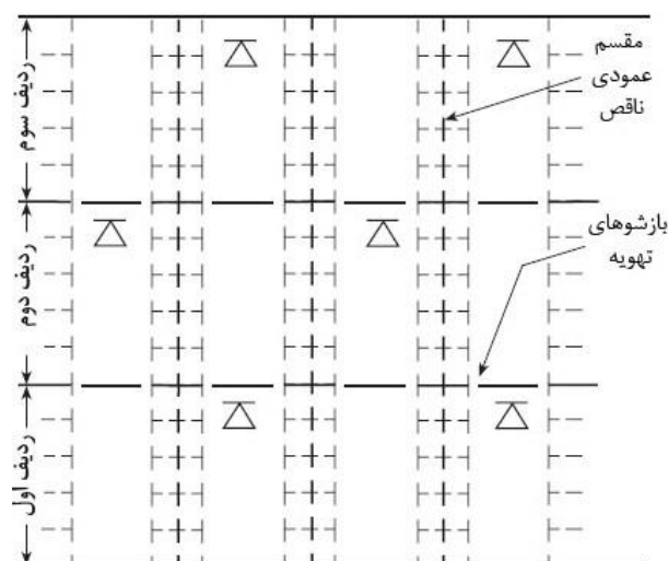
شکل ۸-۱۵-۱۰ ب- اسپرینکلرها در قفسه‌های کتاب چندردیفی با تقسیم‌کننده‌های عمودی غیر کامل
