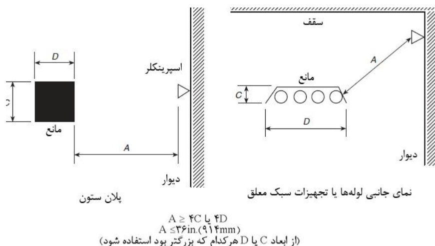
شکل ۷-۱-۲-۷-۱۰-۸- حداقل فاصله از موانع (اسپرینکلهای دیواری اسپری‌کننده مسکونی)
