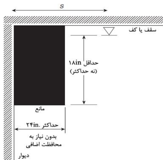
شکل ۸-۱۰-۶-۲-پ- موانع مقابل دیوار (اسپرینکلرهای اسپری کننده بالازن و پایین زن مسکونی)
