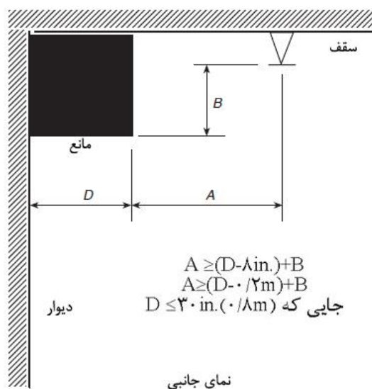
شکل ۸-۱۰-۶-۲-ب- موانع مقابل دیوار (اسپرینکلرهای اسپری کننده بالازن و پایین زن مسکونی)
