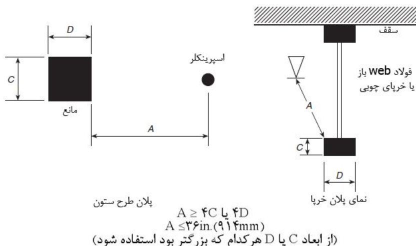
شکل ۸-۱۰-۶-۲-۳ - حداقل فاصله از موانع (اسپرینکلرهای اسپری کننده بالازن - پایین‌زن مسکونی)
