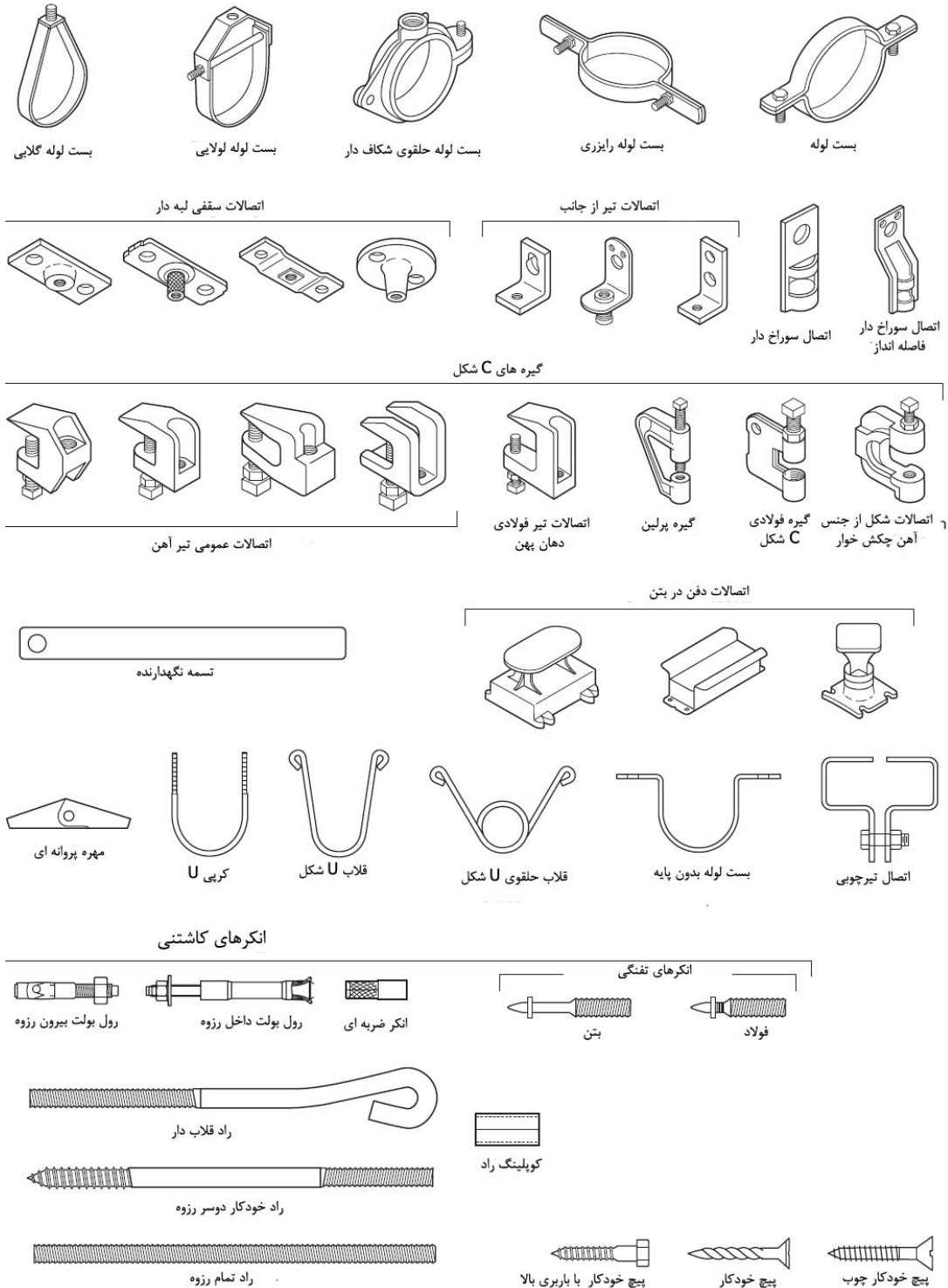
شکل ۹-۵-۱- انواع متداول آویزهای قابل قبول
