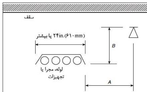
شکل ۸-۱۱-۵-۳-۲ مانع کاملاً زیر اسپرینکلر قرار گرفته است (اسپرینکلرهای CMA)
