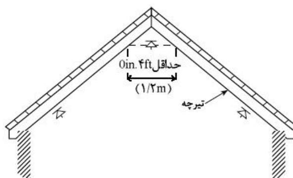
شکل ۸-۶-۴-۱-۳-۳- فاصله افقی برای اسپرینکرها در تاج سقف منظم
