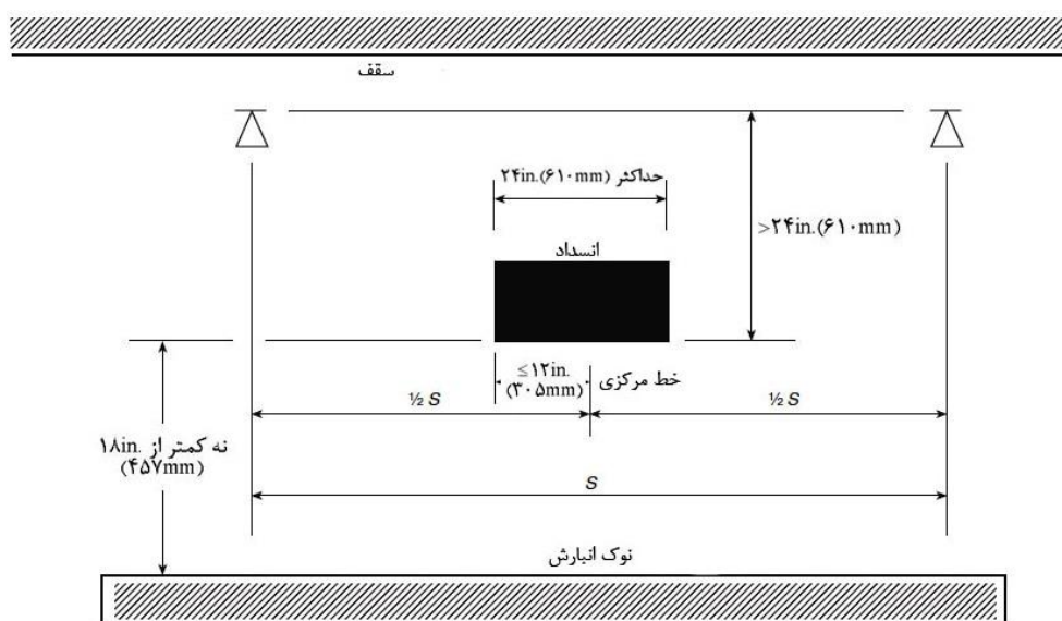
شکل ۸-۱۱-۵-۳ مانع بزرگتر از ۲۴in (۶۱۰mm) زیر اسپرینکلر (اسپرینکرها CMSA)
