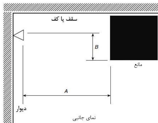
شکل ۸-۱۰-۷-۳- جانمایی اسپرینکلرها برای جلوگیری از موانع (اسپرینکلرهای اسپری کننده دیواری مسکونی)
