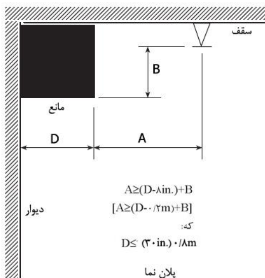
شکل ۸-۶-۵-۲-ب - مانع در مقابل دیوار (SSU/SSP)
