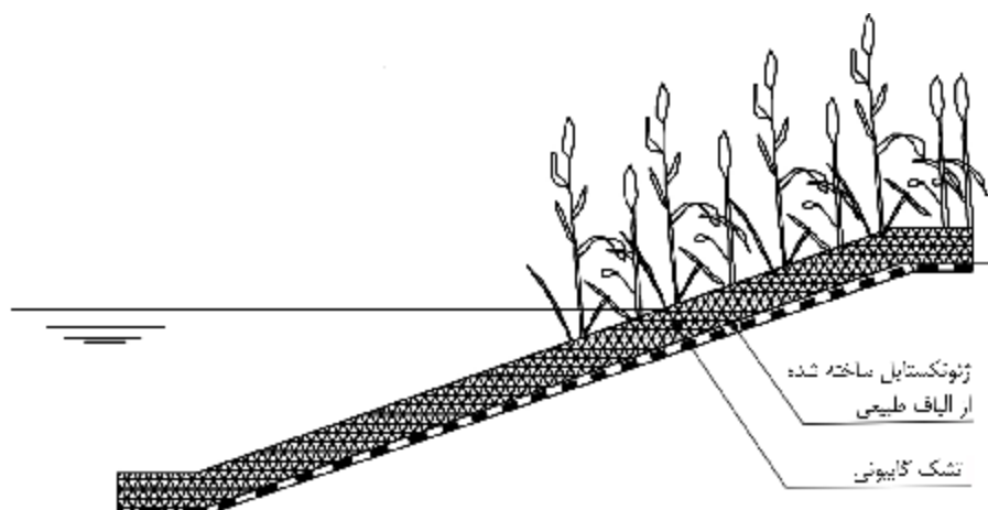
شکل ۱-۵-۱- تشک گابیونی
