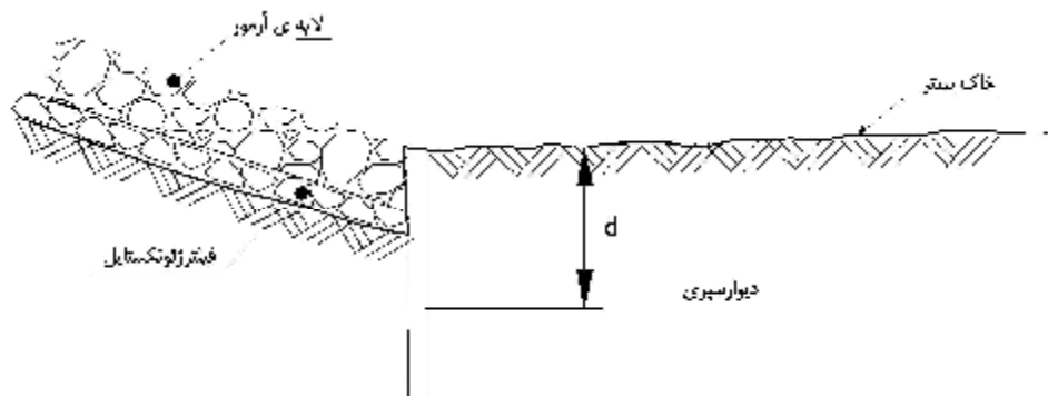
شکل پ-۳-۱۳- پاشنه‌ی منتهی به دیواره‌ی سپری
