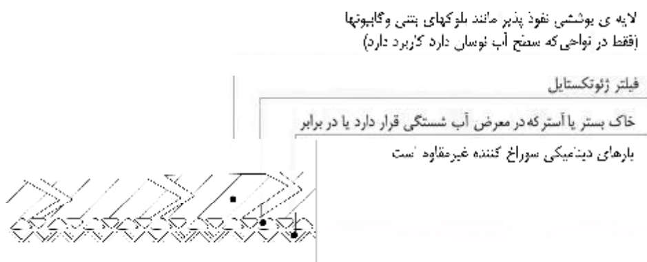
شکل پ-۳-۱۹- لایه‌های متداول آرمور برای حفاظت شیب و بستر
