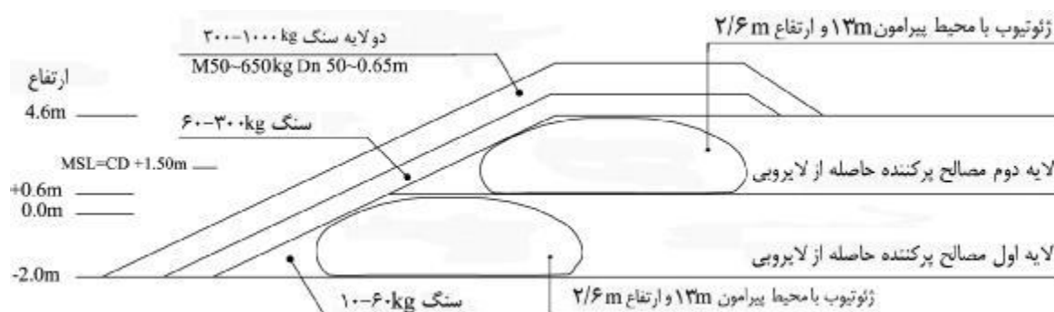
شکل ۸-۹- سطح مقطع سازه‌ی حفاظت ساحلی پیرامون جزیره
