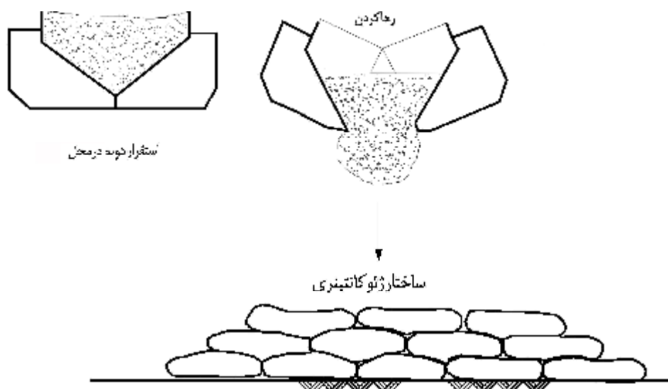
شکل ۲-۸- مراحل پراکنش و نصب ژئوکانتینرها به صورت شماتیک
