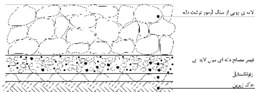
شکل پ-۴-۳- مصالح دانه ای بین لایه های بین ژئوتکستایل و لایه ی رویی (ر.ک. ۶-۵)
