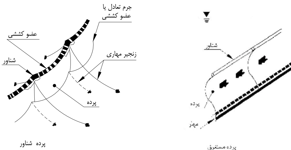
شکل ۲-۱۰- نمونه‌هایی از صفحه‌های شناور
