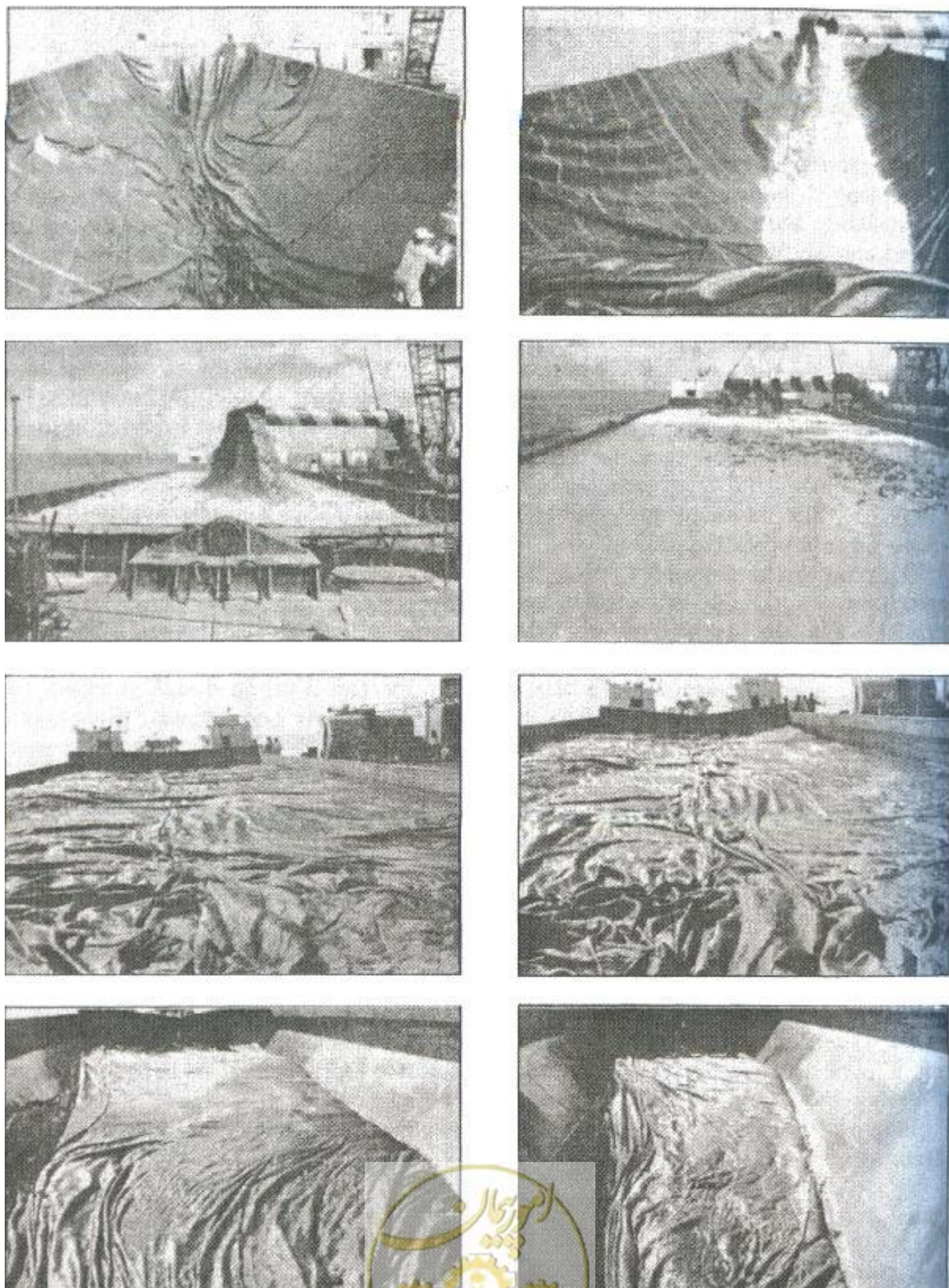
شکل ۲-۹- تصاویری از مراحل پرکردن و استقرار ژئوکانتینرها
