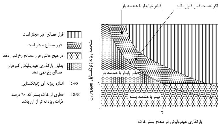
شکل ۱-۴- کاربرد انواع فیلترها در انواع مختلف خاک بستر
