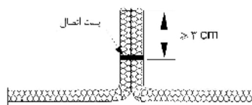
شکل پ-۳-۱۶- اتصال ژئوتکستایل با سطح غیر صفحه‌ای (مانند دیواره سپری) - گزینه ۲
