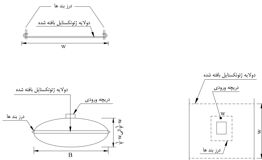
شکل ۲-۴-۱-۱ جزای ژئوتیوب
