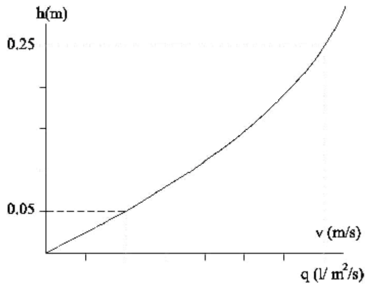
شکل ۴-۱- تغییر سرعت جریان و دبی در واحد طول جریان بر حسب ارتفاع ستون آب (h)
