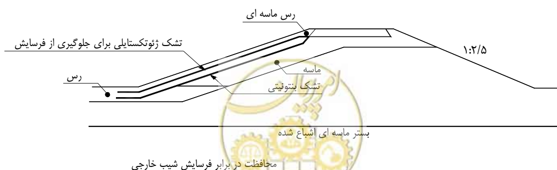
شکل ۱-۱۶ - نمونه هایی از کاربرد ژئوتکستایل ها در مقاوم سازی بندهای خاکی
