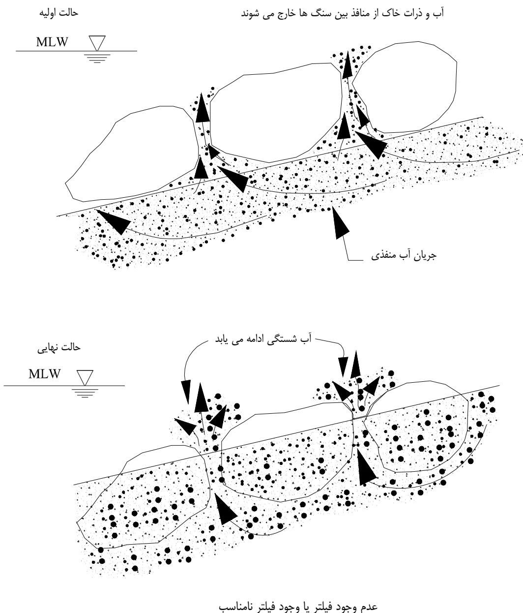
شکل ۱-۵- نمونه‌ای از دو حالت عدم وجود فیلتر یا وجود فیلتر نامناسب مصالح سنگی
