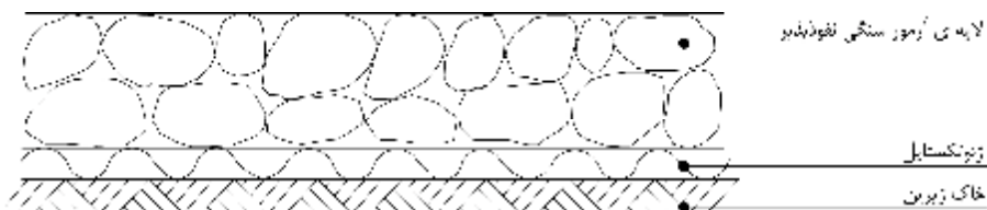
شکل پ-۱-۳- ژئوتکستایلی که مستقیماً بر روی خاک زیرین قرار گیرد: کاربرد متداول (ر.ک. ۶-۲)
