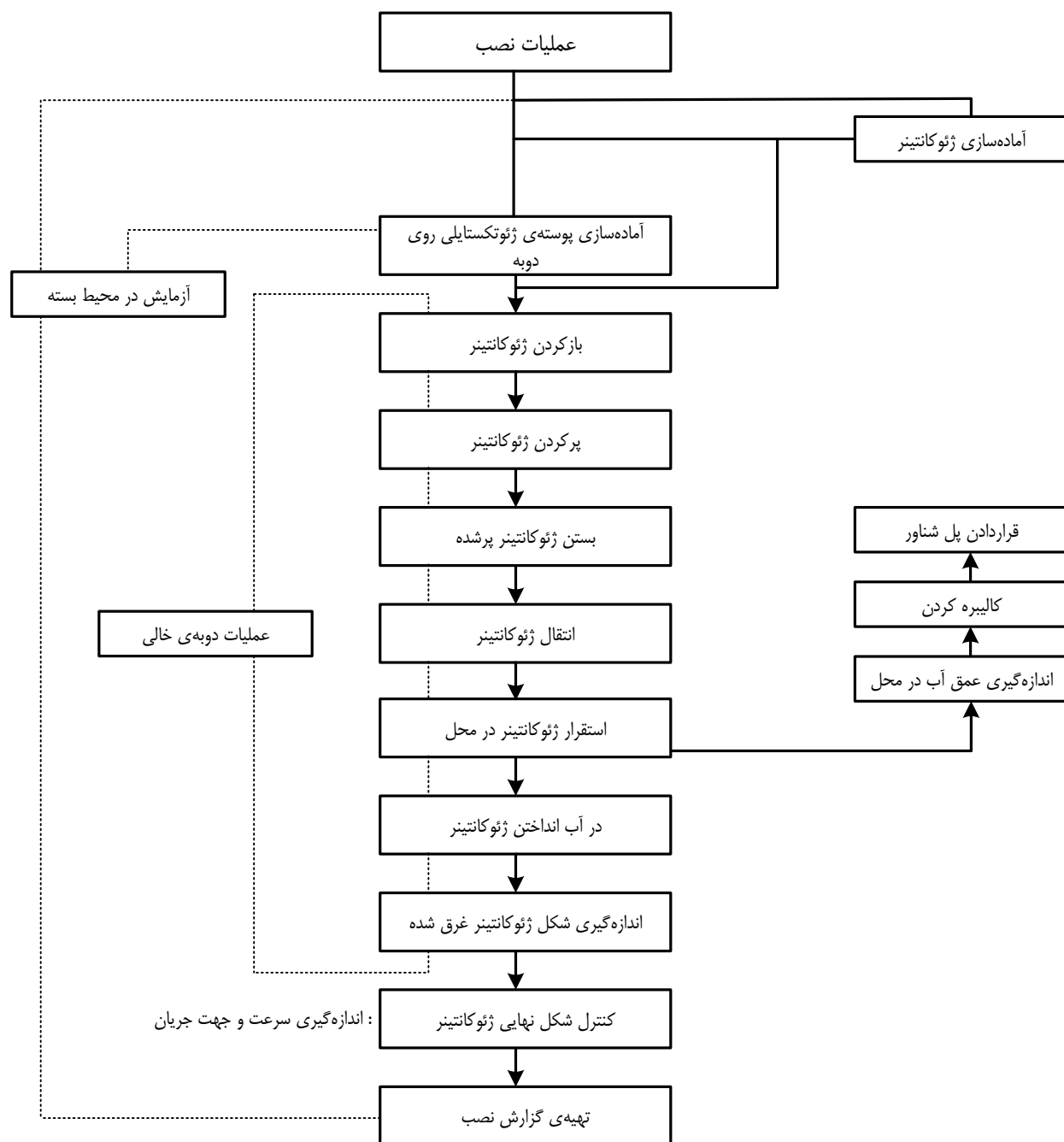
شکل ۲-۷- فلوچارت نصب ژئوتکستایلها
