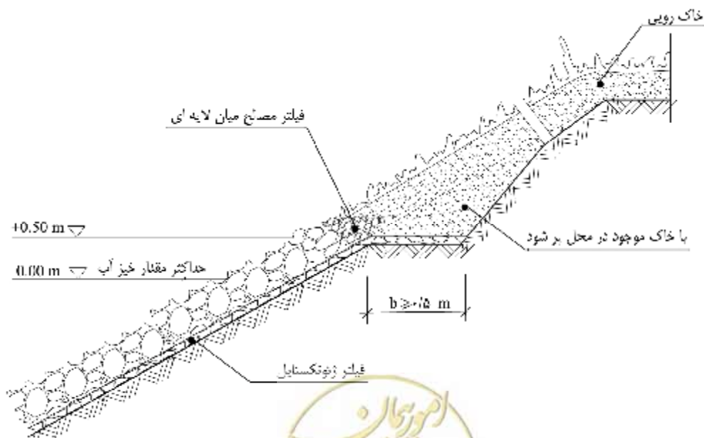
شکل پ-۳-۱۰- لبه‌ی بالایی فیلتر در حالت شیب طولانی یک سازه با ارتفاع آزاد زیاد
