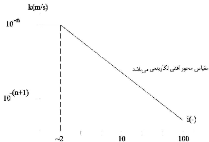
شکل ۴-۲- تغییر ضریب نفوذپذیری بر حسب گرادیان هیدرولیکی
