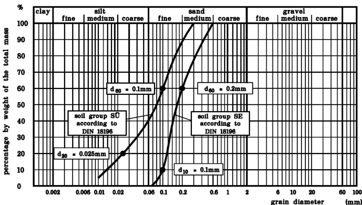
شکل پ-۱-۷- بازه ی دانه بندی خاک بستر
