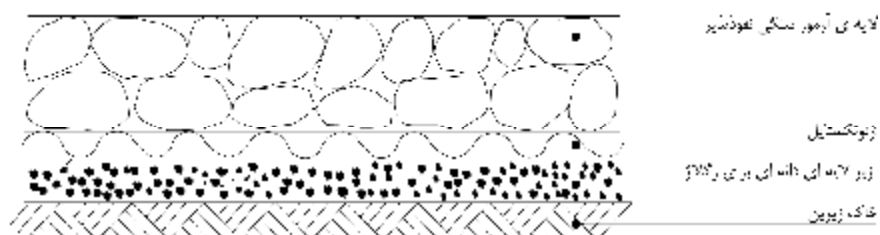
شکل پ-۲-۳- ژئوتکستایل بر روی زیر لایه ی رگلاژ از مصالح دانه سنگی (ر.ک. ۶-۳)
