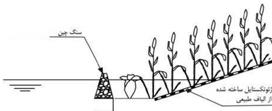
شکل ۱۱-۱- سازه‌ی حفاظتی دائمی از نوع سنگ‌چین
