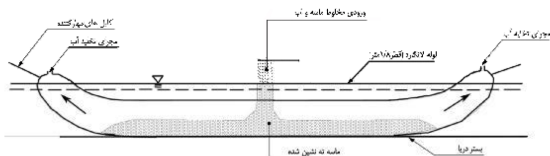
شکل ۱-۲- روش پرکردن لوله‌ی لانگارد (سطح مقطع)
