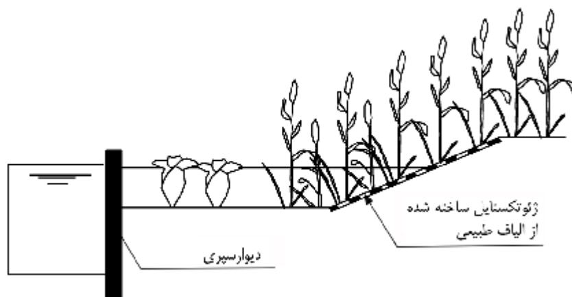
شکل ۱۰-۱- سازه‌ی حفاظتی دائمی از نوع دیوار سبیری
