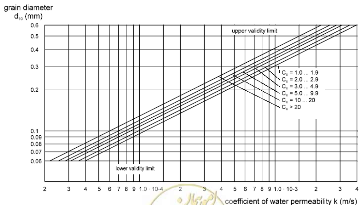
شکل پ-۴-۲- ضریب نفوذپذیری برحسب ضریب یکنواختی و اندازه‌ی d_{10} ذرات خاک
