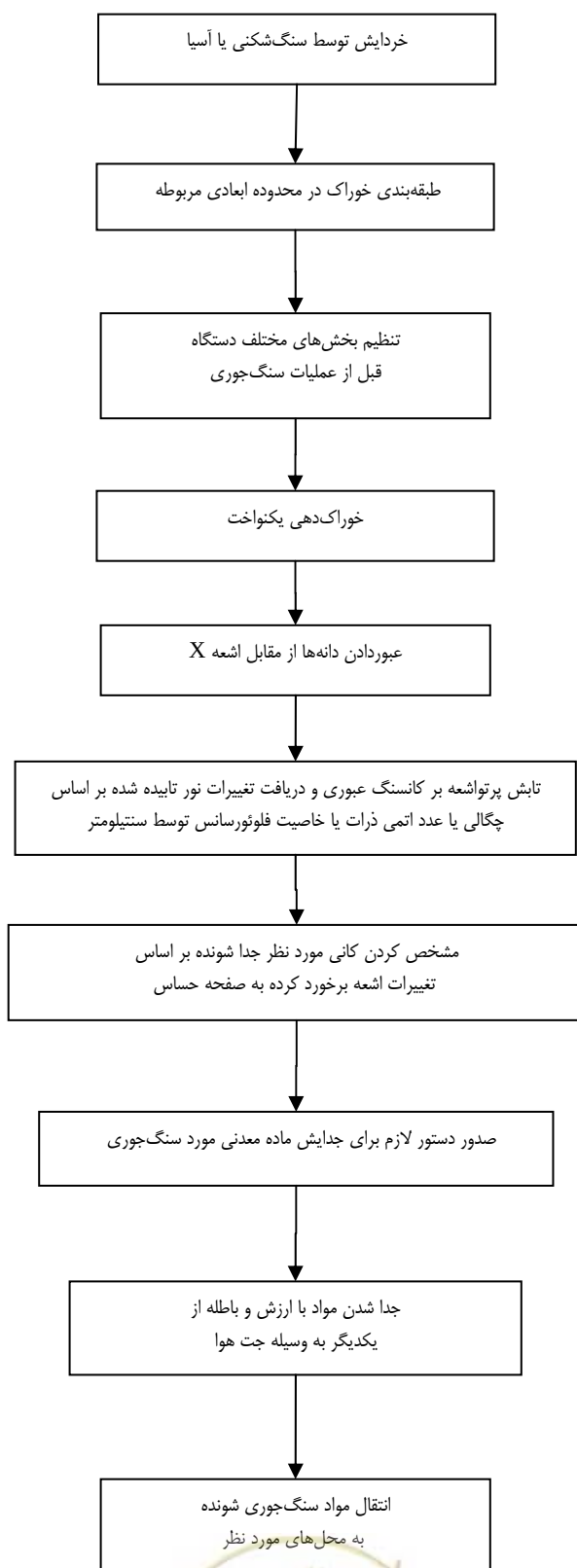
شکل ۳-۶- روند نمای سنگ‌چوری با استفاده از پراش اشعه X
