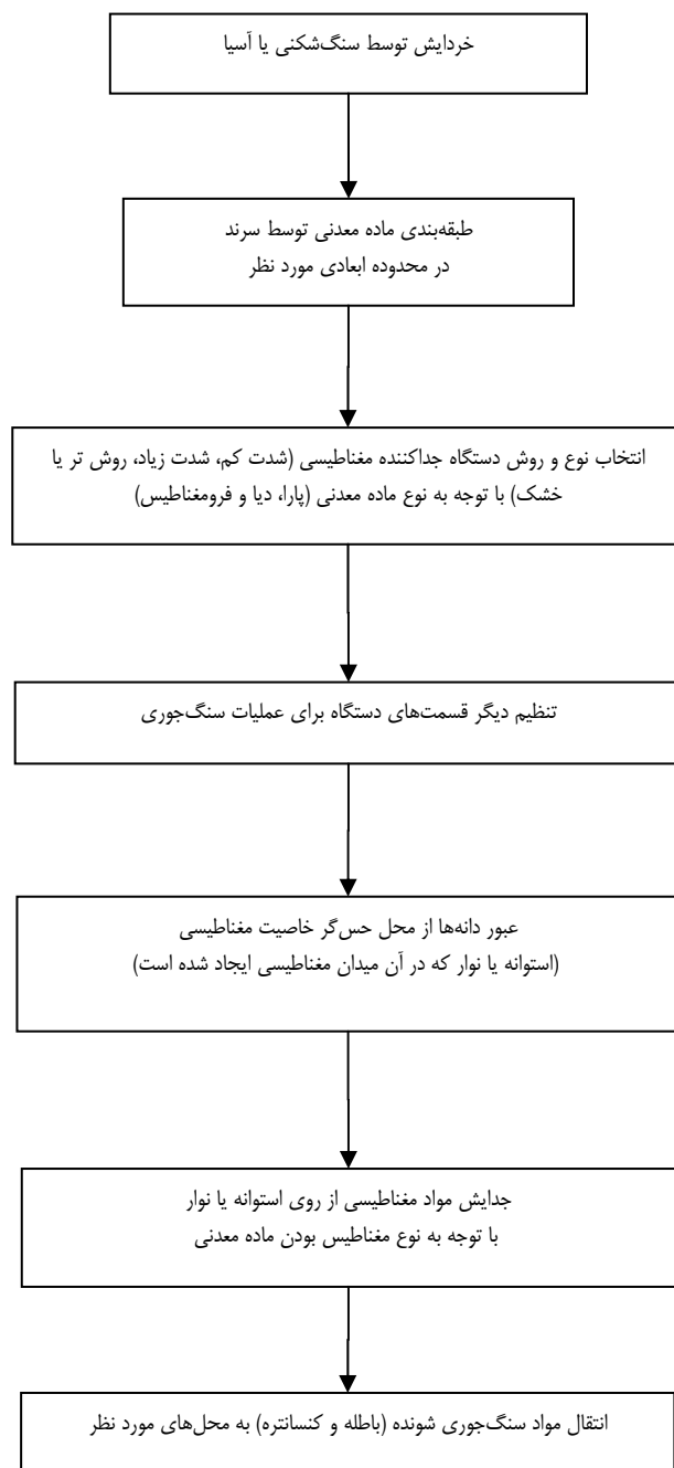
شکل ۳-۹- روند نمای سنگ‌جویری با استفاده از خاصیت مغناطیسی
