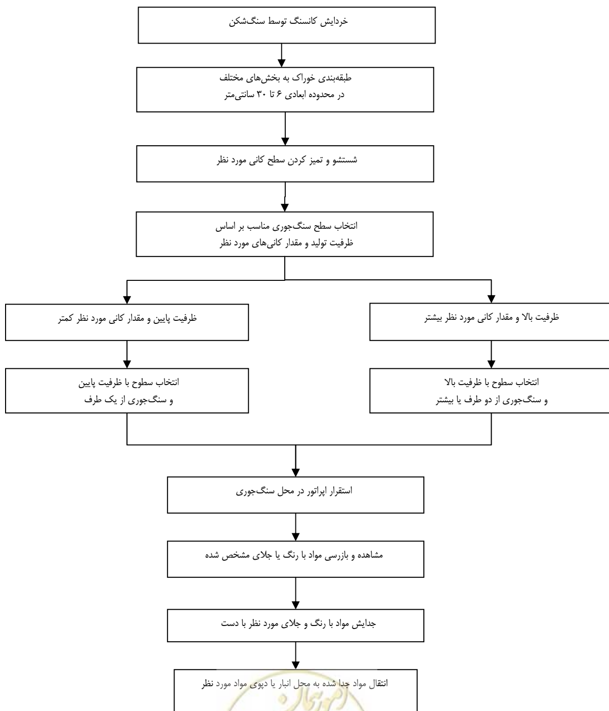
شکل ۳-۲- روندنمای سنگ‌جوری دستی بر اساس رنگ و جلا
