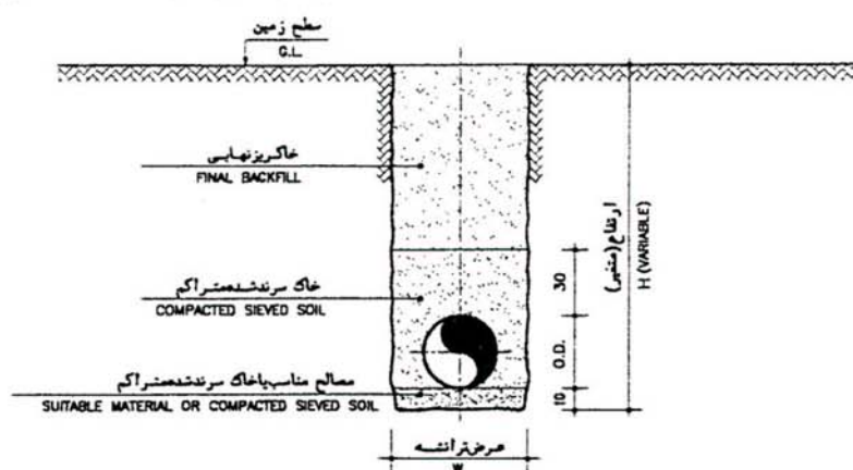
مقطع ترانشه TRENCH SECTION N.T.S
