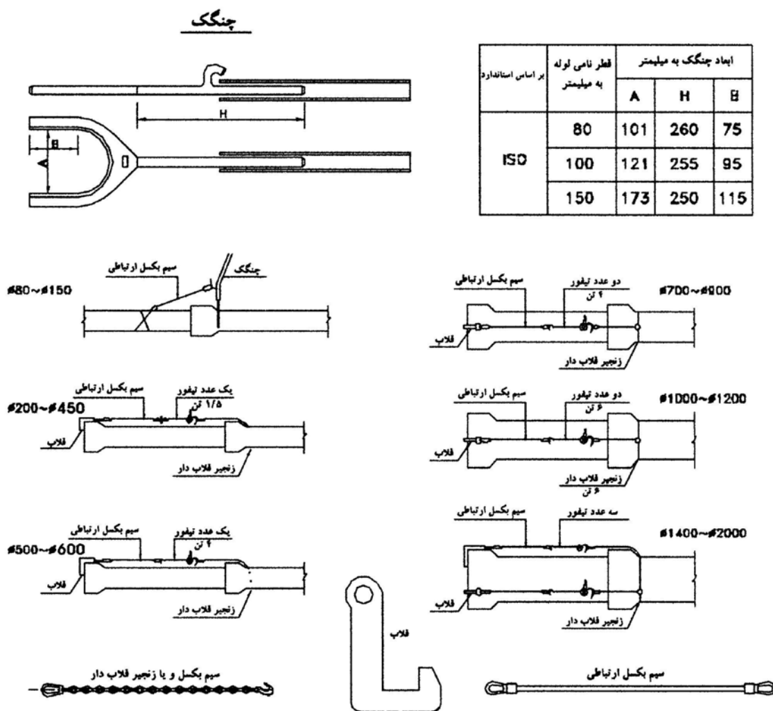
شکل ۲-۲-۱۲: ابزار و تجهیزات معمول برقراری اتصال لوله‌های چدن نشکن (برای اتصالات فشاری و مکانیکی)
