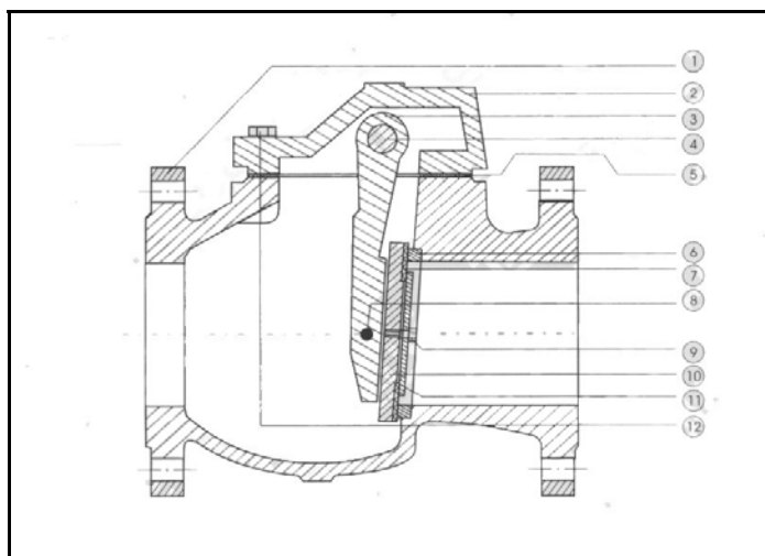
شکل ۴-۲-۳۵: اجزای شیر یکطرفه لولایی (اطلاعات شکل در جدول ۴-۲-۱)
