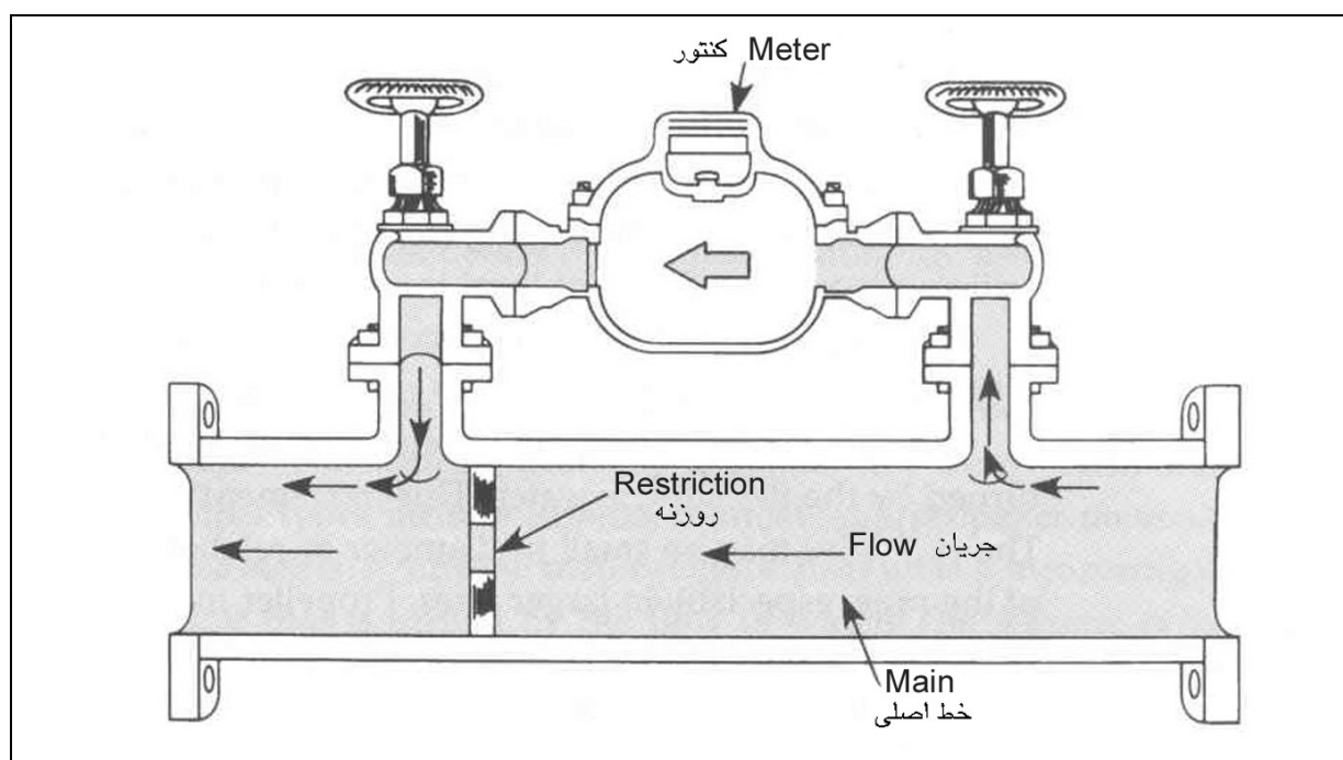
شکل ۴-۲-۵۵: کنتور تناسبی
