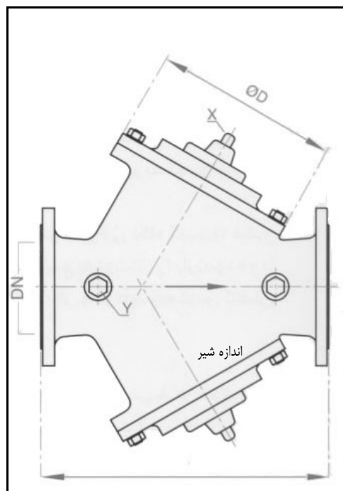
شکل ۴-۲-۲: شیر کنترل پایلوت دار مایل با دو محفظه کنترل
