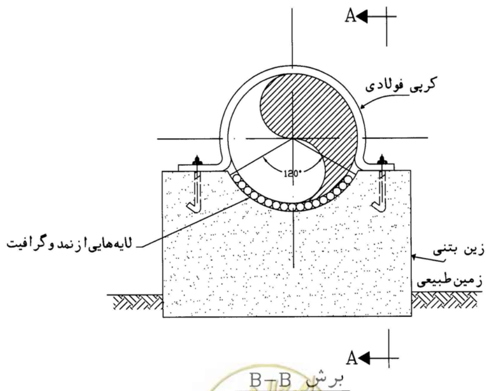
شکل ۱-۲-۷: تکیه‌گاه از نوع زین بتنی
