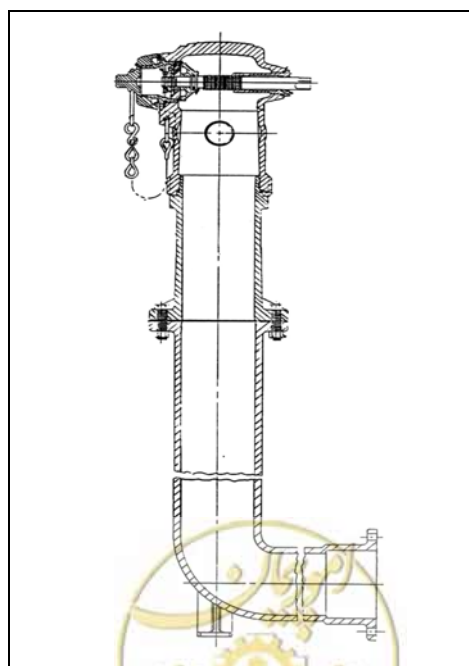
شکل ۴-۲-۴: شیر آتش نشانی ایستاده با محفظه تر
