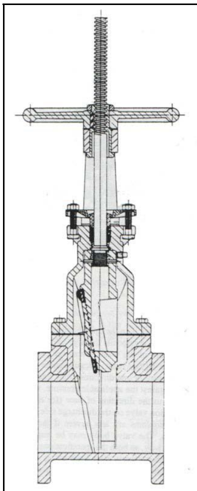
شکل ۴-۲-۱۰: شیر کشویی با ساقه بالارونده
