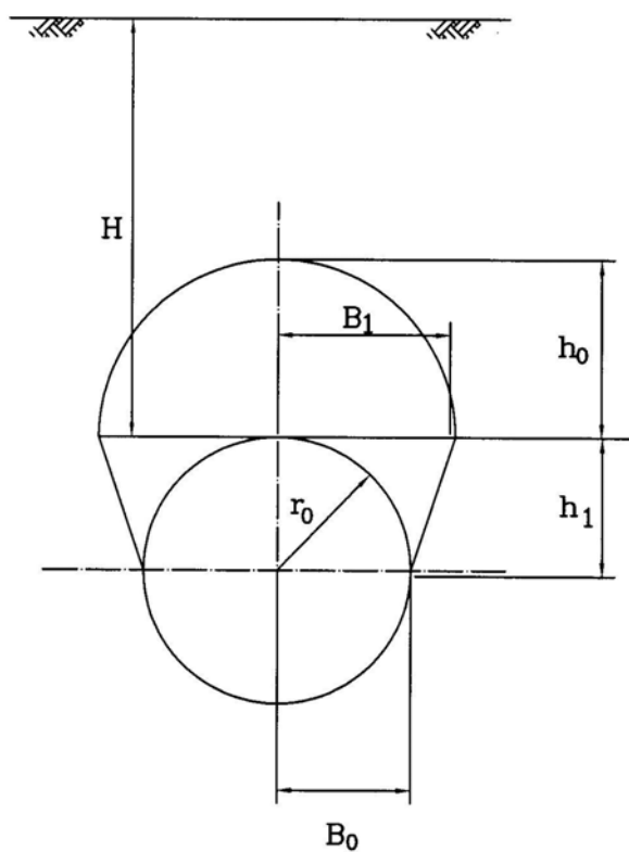
شکل ۶-۳: فشارهای وارد بر لوله در حین جک‌زنی
