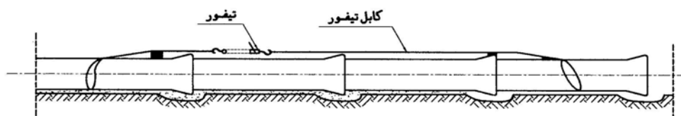
برقراری نهایی اتصال توسط کشش از طریق بدنه خارجی لوله
