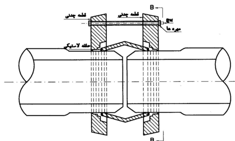
مقطع (A-A) اتصال ژئو- پلیمر بعد از بست کردن مهره ها
