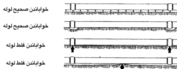
شکل ۱-۲-۲: نحوه خواباندن صحیح لوله در ترانشه
