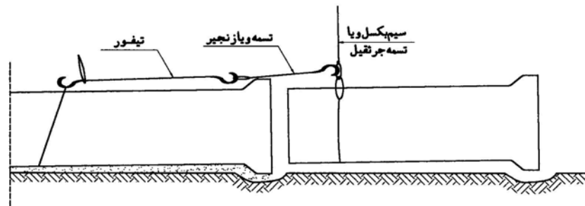
برقراری اتصال لوله ها توسط جرثقیل و تیغور
