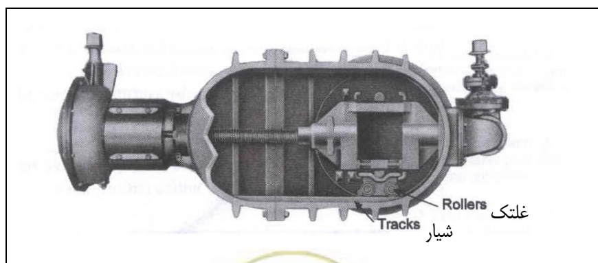
شکل ۴-۲-۱۱: شیر کشویی افقی
