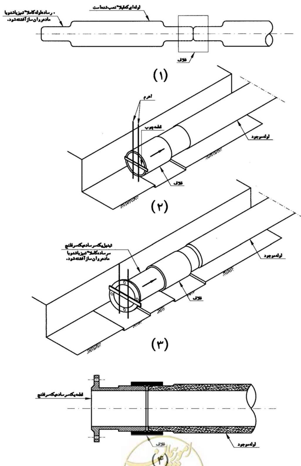
شکل ۲-۴-۱۲: اصول، نحوه و مراحل نصب قطعه یک سر ساده و یک سر فلنج به سر ساده لوله‌های آریست سیمان
