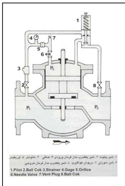
شکل ۴-۲-۲: شیر رهاکننده فشار
