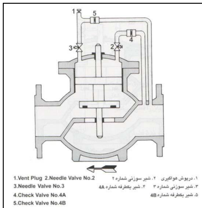
شکل ۴-۲-۲۷: شیر یکطرفه پایلوت‌دار
