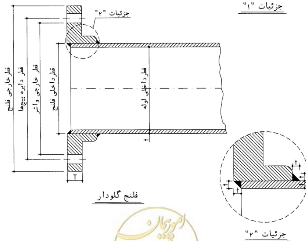
شکل ۲-۱-۴: جوشکاری اتصال فلنجی
