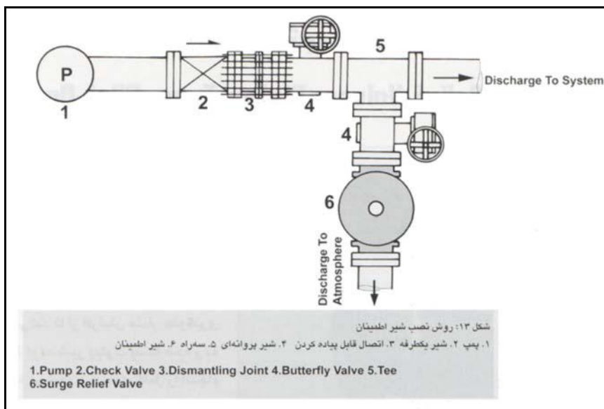
شکل ۴-۲-۲۶: شیر اطمینان کاهنده ضربه قوچ
