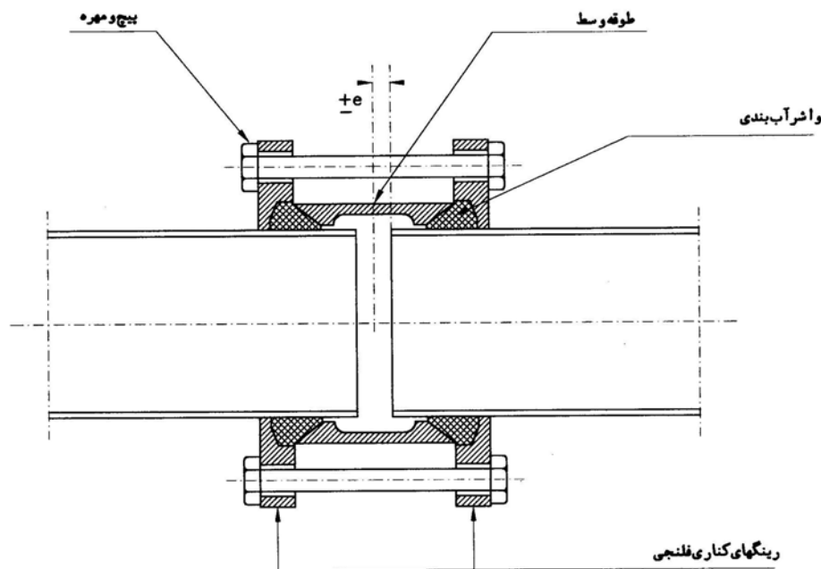
شکل ۱-۱-۴: قطعه قابل انعطاف
