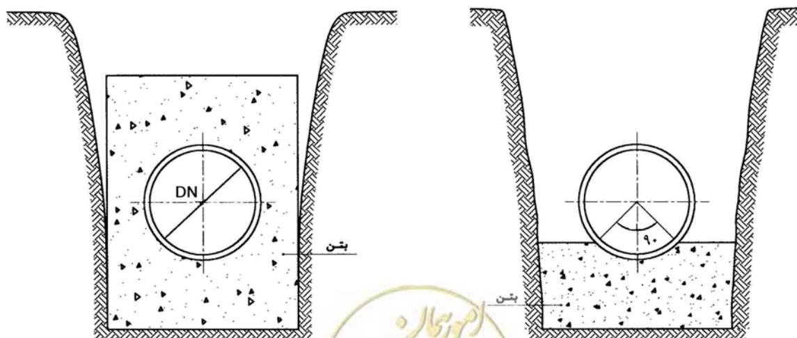
شکل ۲-۳-۱۵: کارگذاری و مهار لوله‌های بتنی تحت فشار در شیب
