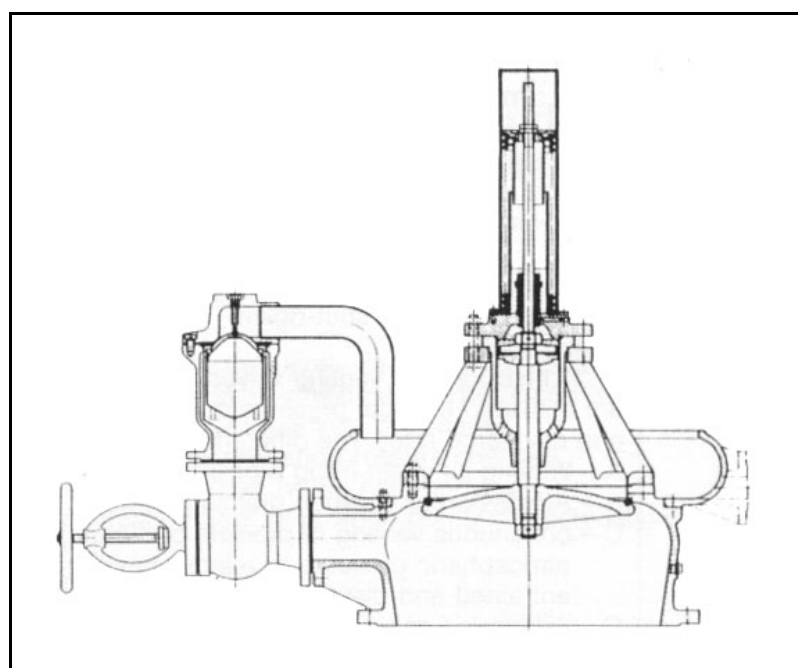
شکل ۴-۲-۴۰: شیر خلا شکن
