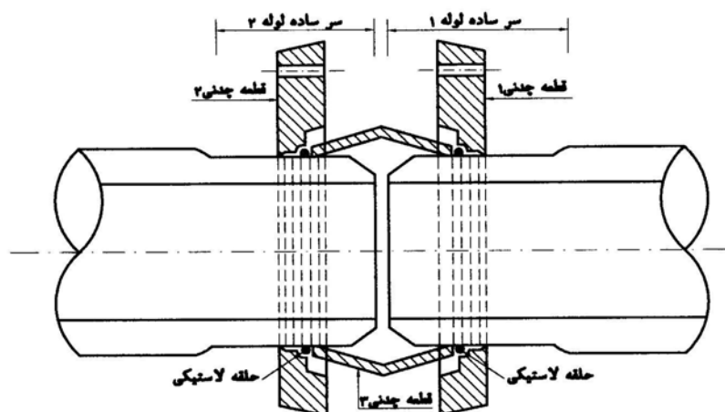
مقطع (A-A) اتصال ژئو- پلیمر قبل از بست کردن مهره ها
