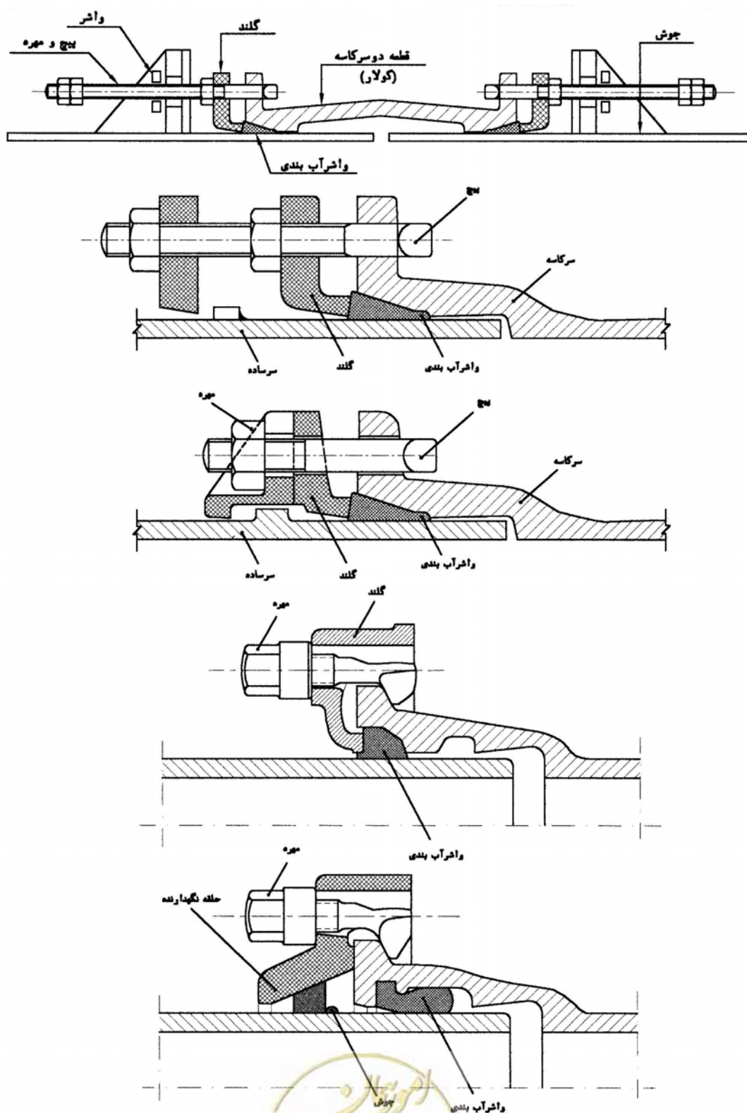
شکل ۲-۲-۵: انواع خاص اتصال مکانیکی
