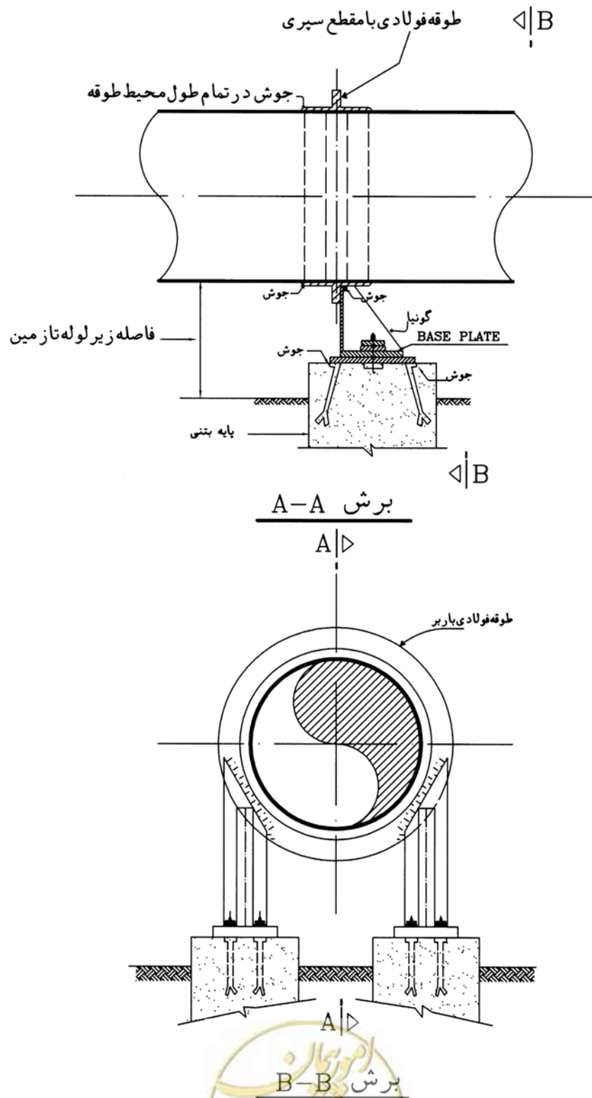
شکل ۲-۱-۸: تکیه گاه از نوع طوقه باریک
