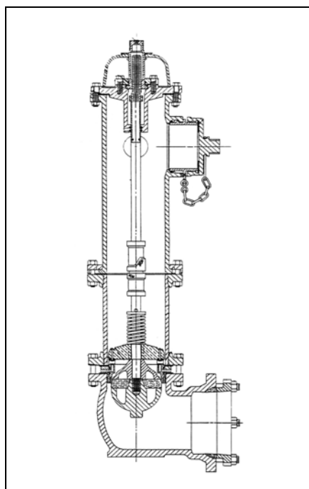
شکل ۴-۲-۴: شیر آتش نشانی ایستاده با محفظه خشک
