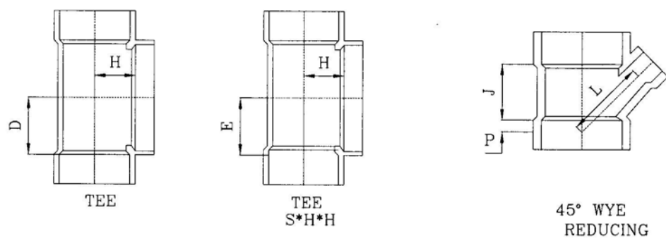
شکل ۴-۱-۵-۱۹: سه راهی به شکل Y یا T در لوله اصلی
