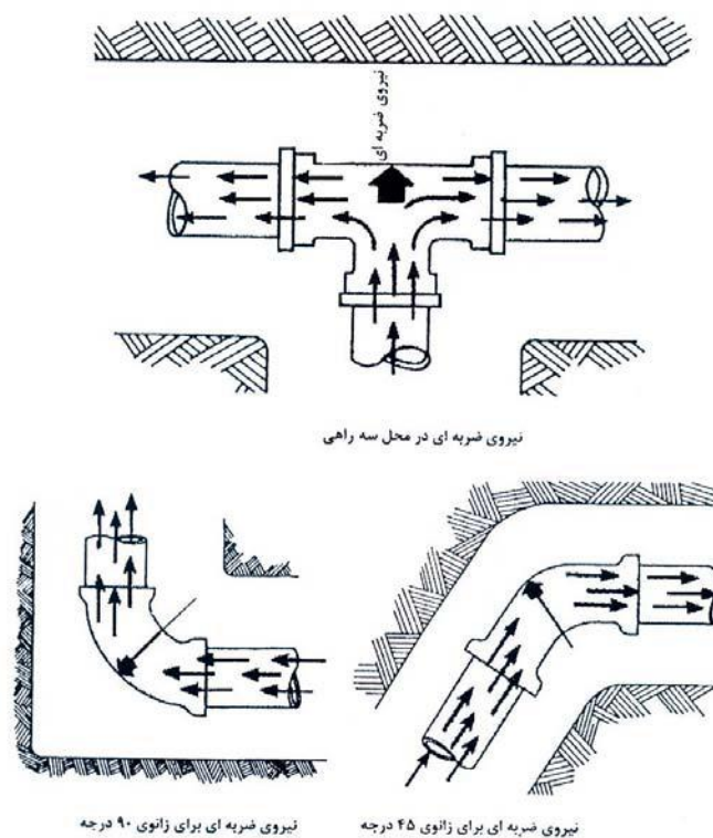
شکل ۱-۴-۹-۲-۱: نحوه اثر نیروی ضربه ای
