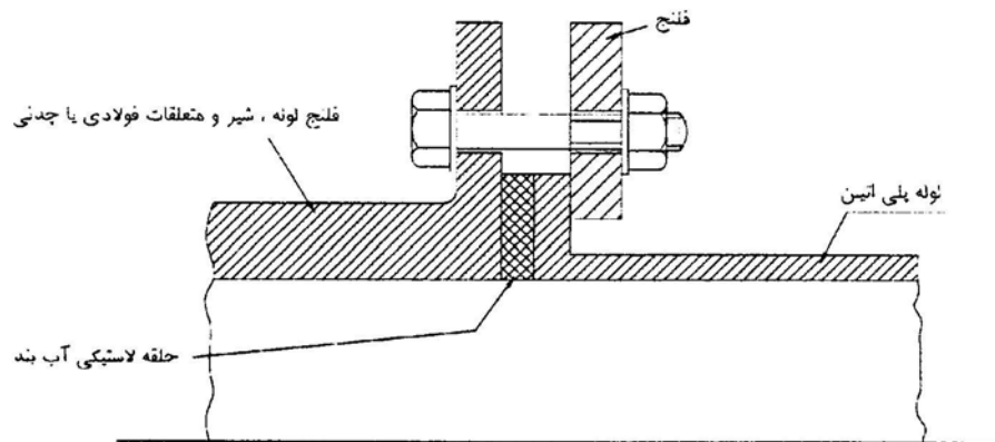
شکل ۲-۴: اتصال به روش فلنجی
