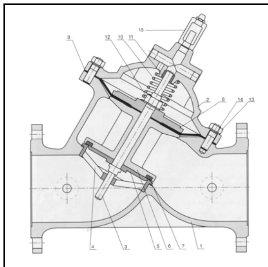
شکل ۴-۲-۱۹: شیر کنترل پایلوت دار با محفظه کنترل مایل
