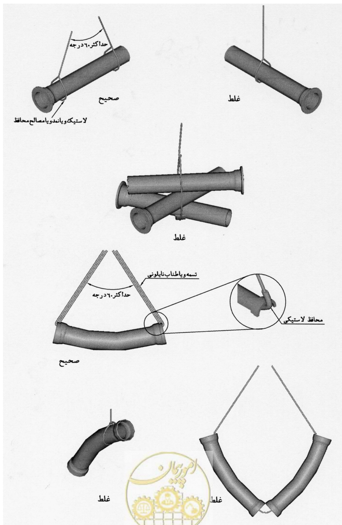
شکل ۷-۲-۲: نحوه بلند کردن لوله و متعلقات
