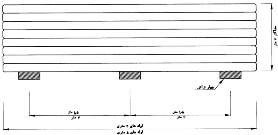
شکل ۲-۴-۶: چین طولی لوله
