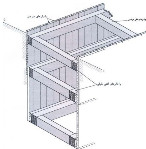
شکل ۱-۲-۱۱: اعضای اصلی یک چوب‌بست نمونه
