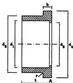
شکل ۴-۱-۵: بوشن پی.وی.سی با جدار خارجی صاف
