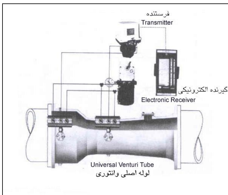
شکل ۴-۲-۵۶: اندازه گیر جریان وانتوری
