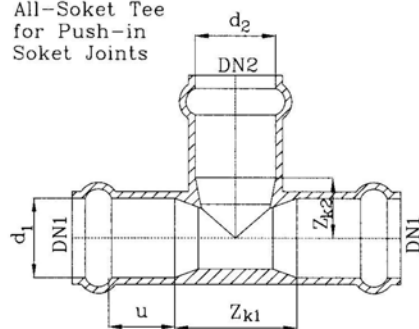
سه راهی سه سر کاسه
