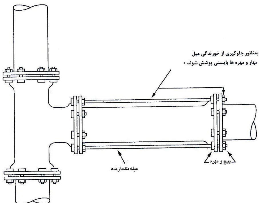
شکل ۱-۲-۱۰: جذب نیروی ضربه‌ای بوسیله میل مهر
