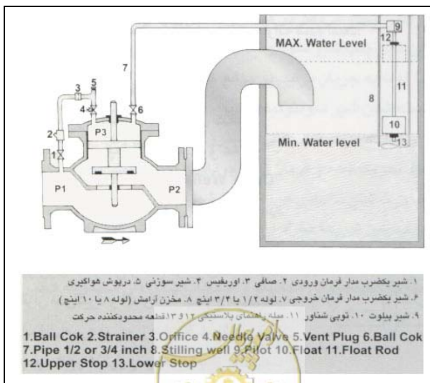
شکل ۴-۲-۳: شیر کنترل سطح آب در مخازن (فلوتر)
