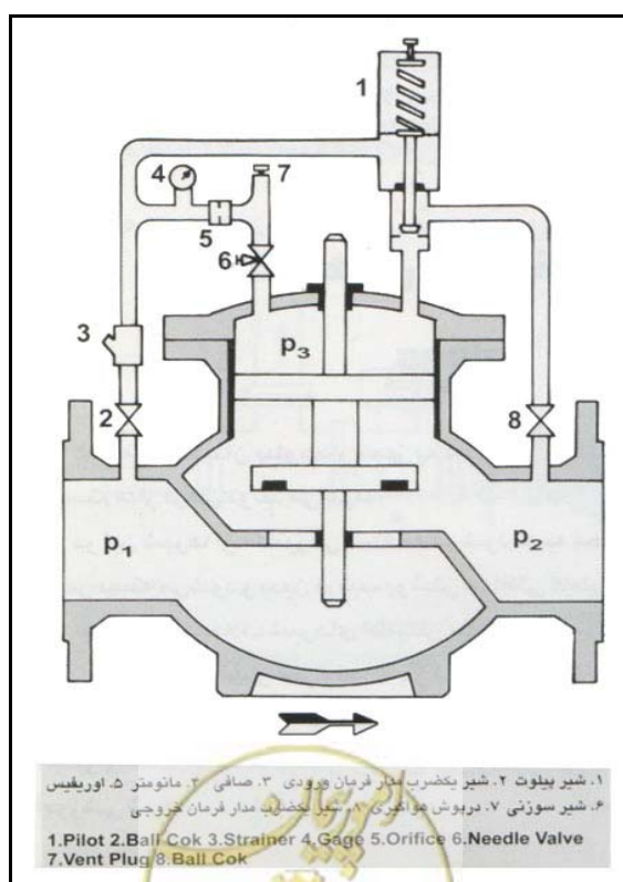
شکل ۴-۲-۲: شیر ثابت نگهدارنده فشار
