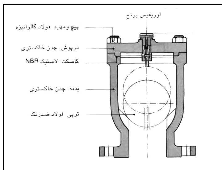
شکل ۴-۲-۳۷: شیر تخلیه هوای یک روزنه (با روزنه کوچک)
