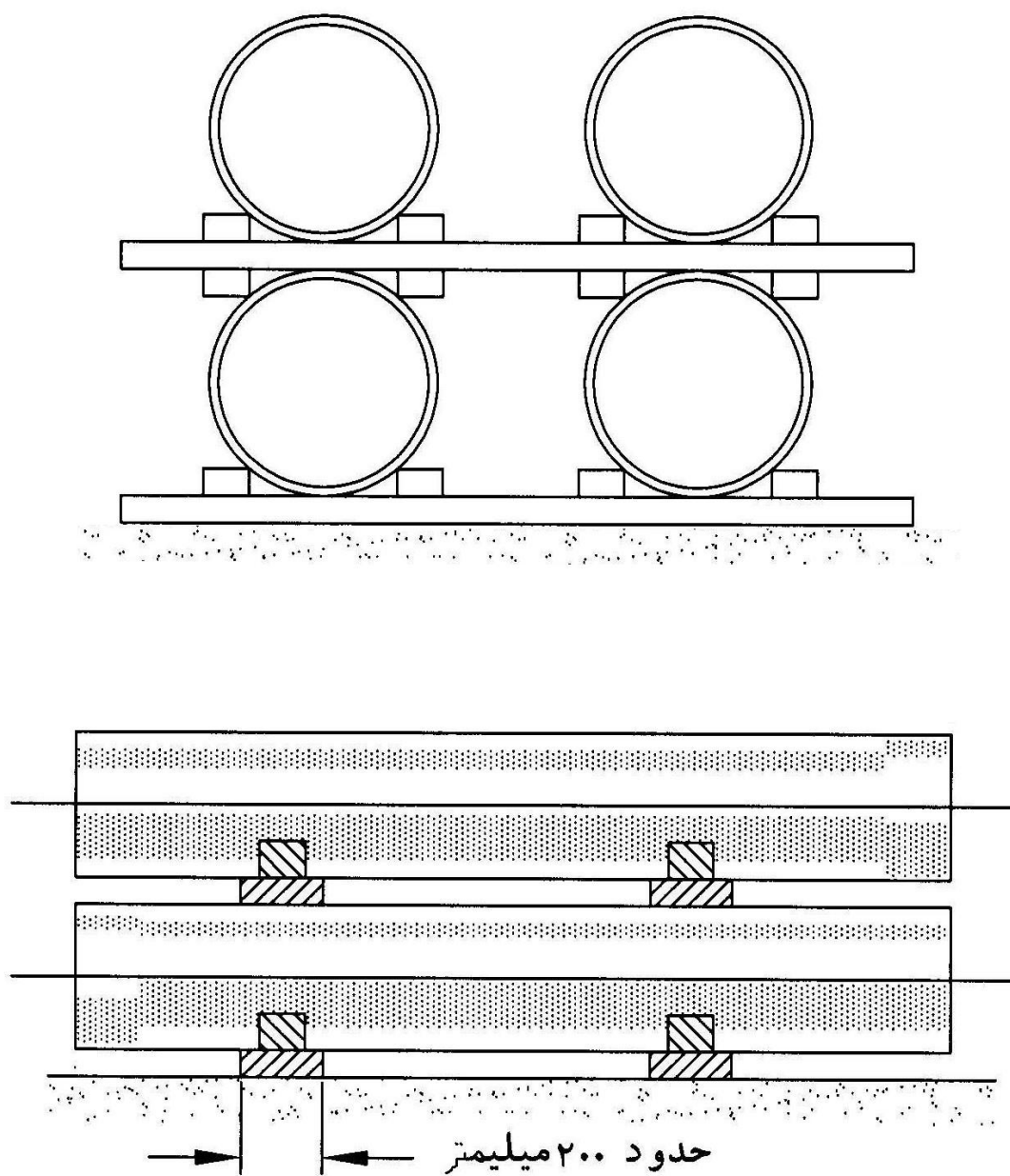
شکل ۲-۷-۱۴: انبار نمودن لوله‌های فایبرگلاس
