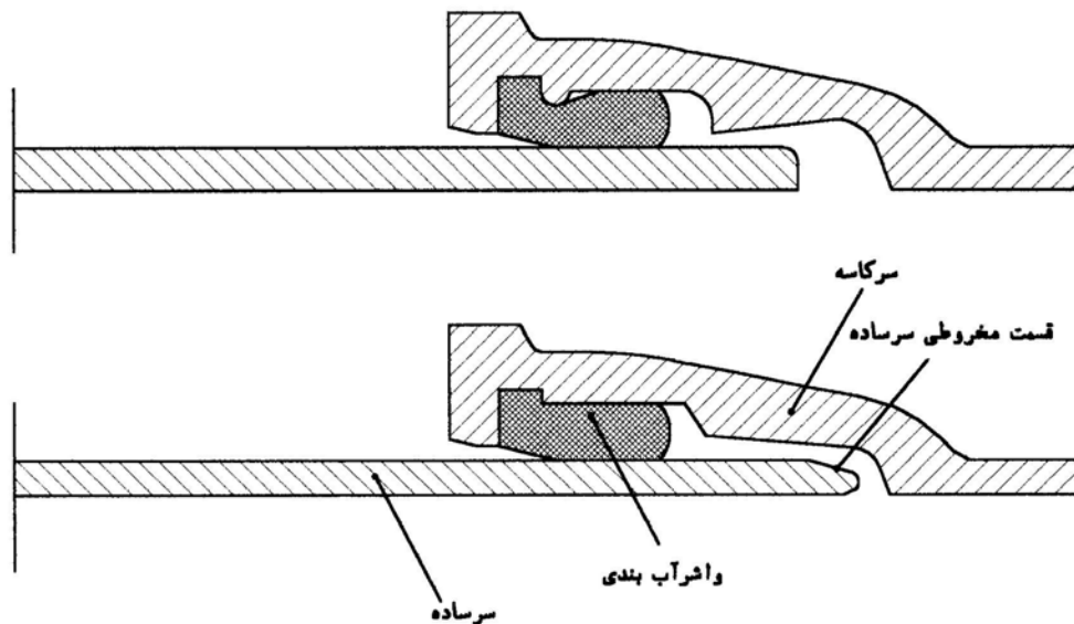
شکل ۲-۲-۱: نمونه‌هایی از اتصال نوع فشاری
