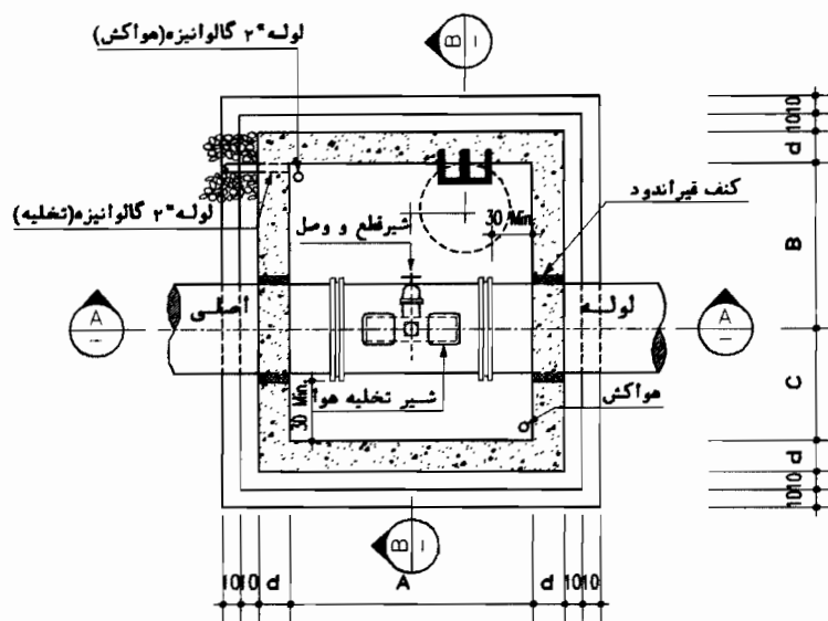
P L A N N.T.S
