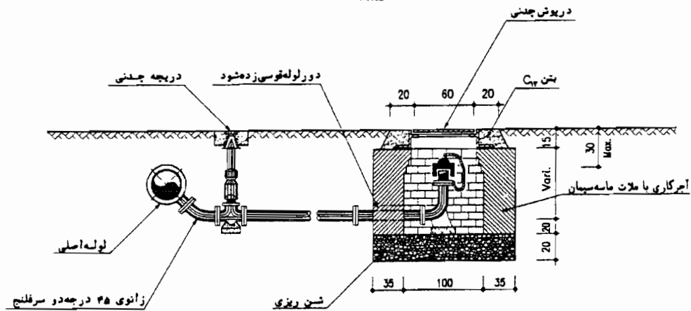
PLAN N.T.S.
