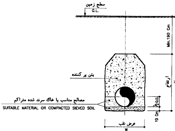
مقطع نوب
