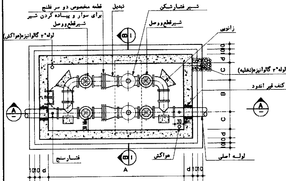
PLAN N.T.S
