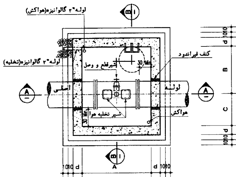
PLAN N.T.S
