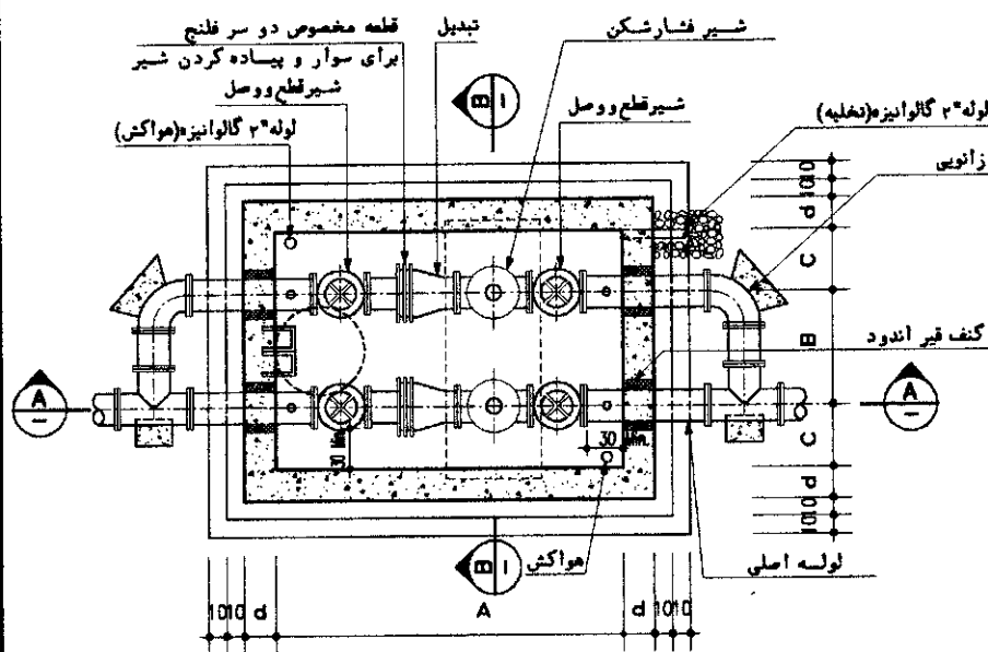
PLAN N.T.S
