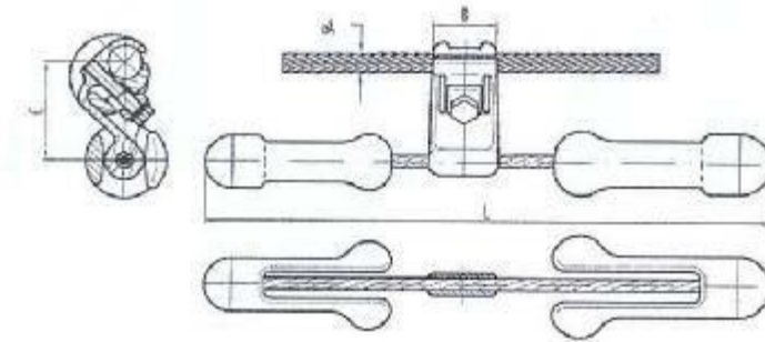
شکل ۵-۲: دمپر استوک بریج
