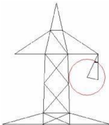
شکل ۸-۳: بررسی تأمین فاصله عایقی S_L در صورت افزایش مقاومت زمین
