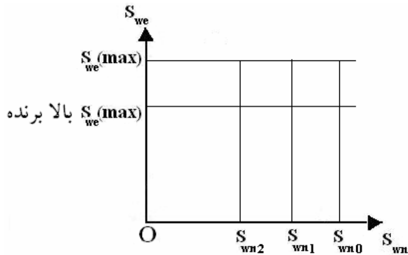
شکل ۲-۱۰: نمونه ای از منحنی کاربردی یک برج کششی
