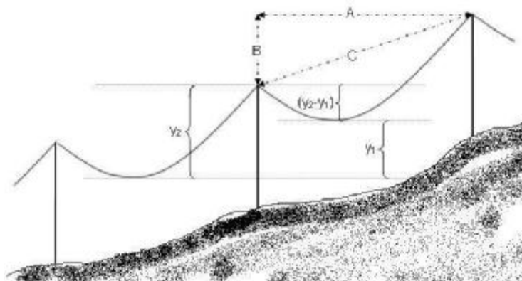
شکل ۱۴-۲: نمونه‌ای از پارامترهای موردنیاز در جدول افست
