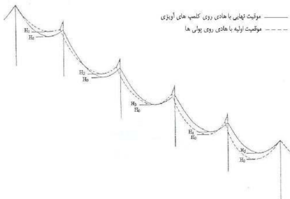
شکل ۱۱-۲: نمایش موقعیت اولیه و نهایی هادی روی پولی و کلمپ
