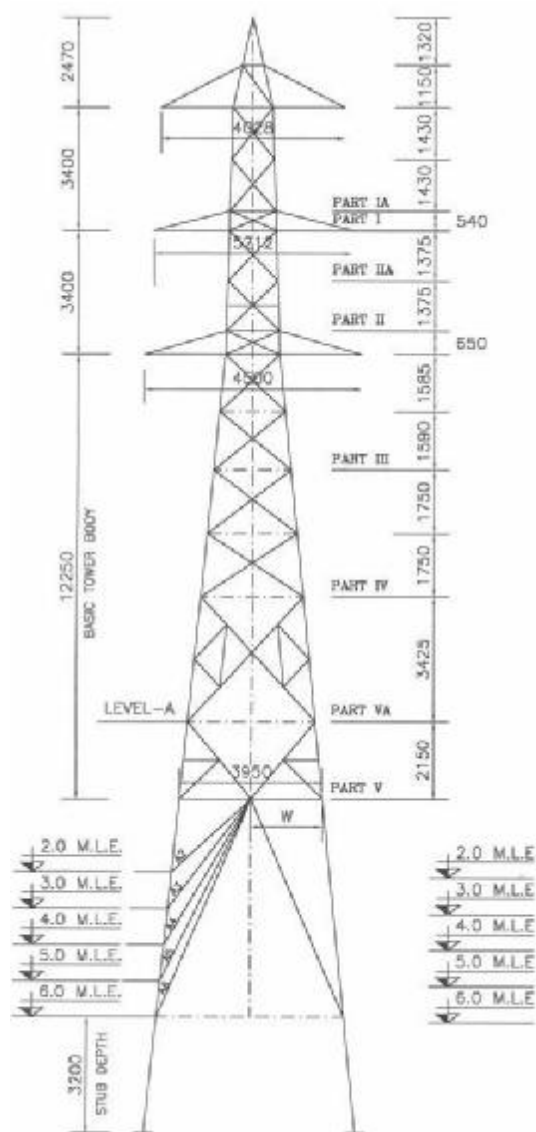
شکل ۳-۳: ابعاد برج NN مورد استفاده در طراحی
