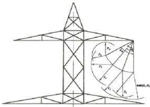
شکل ۲-۲: دیاگرام فواصل هوایی روی برج
