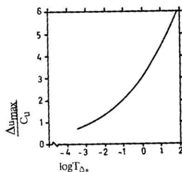
شکل شماره (۹-۱۱) - نمودار ارتباط عامل زمان ۵۰٪ تحکیم با فشار حفره ای حداکثر
