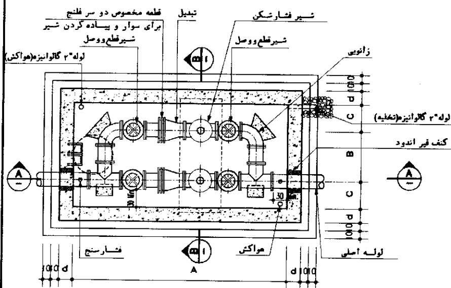
PLAN N.T.S
