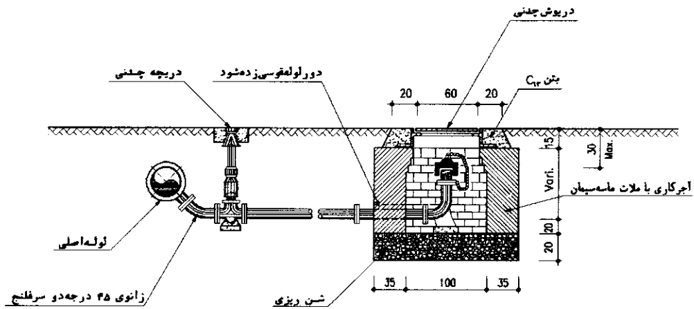
PLAN N.T.S
