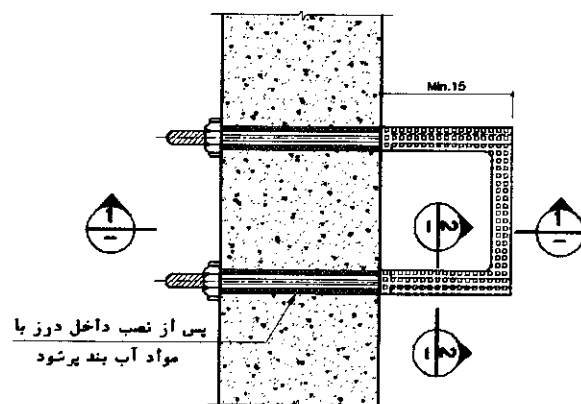
PLAN N.T.S
