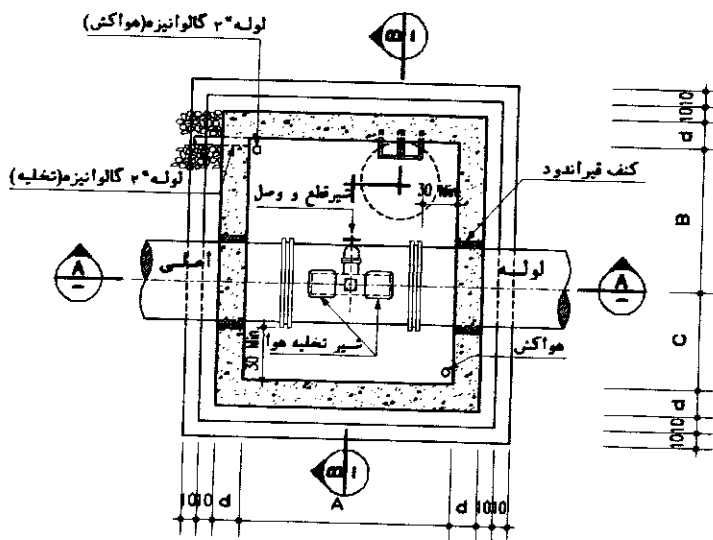
PLAN N.T.S.
