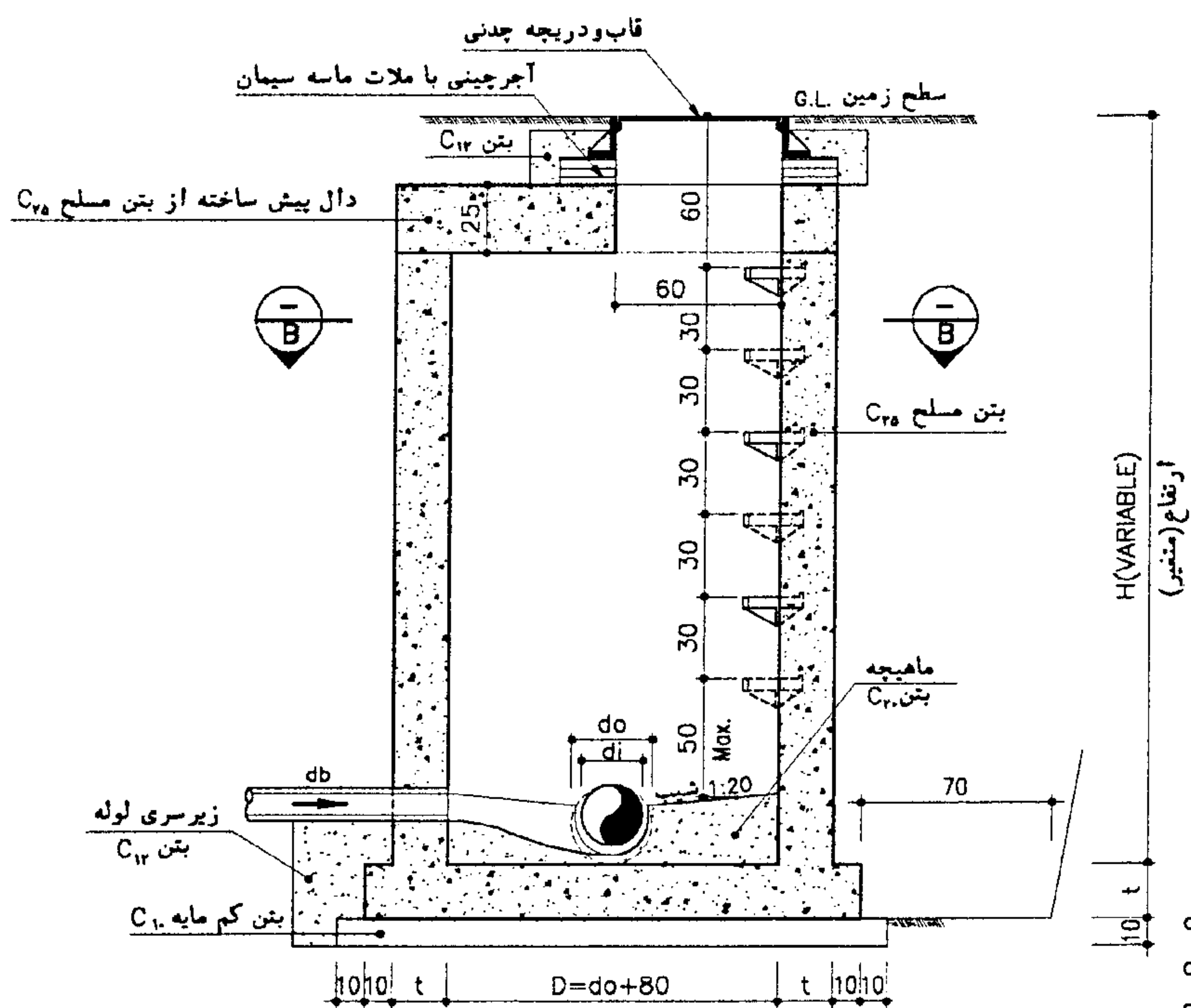
SECTION A-A
