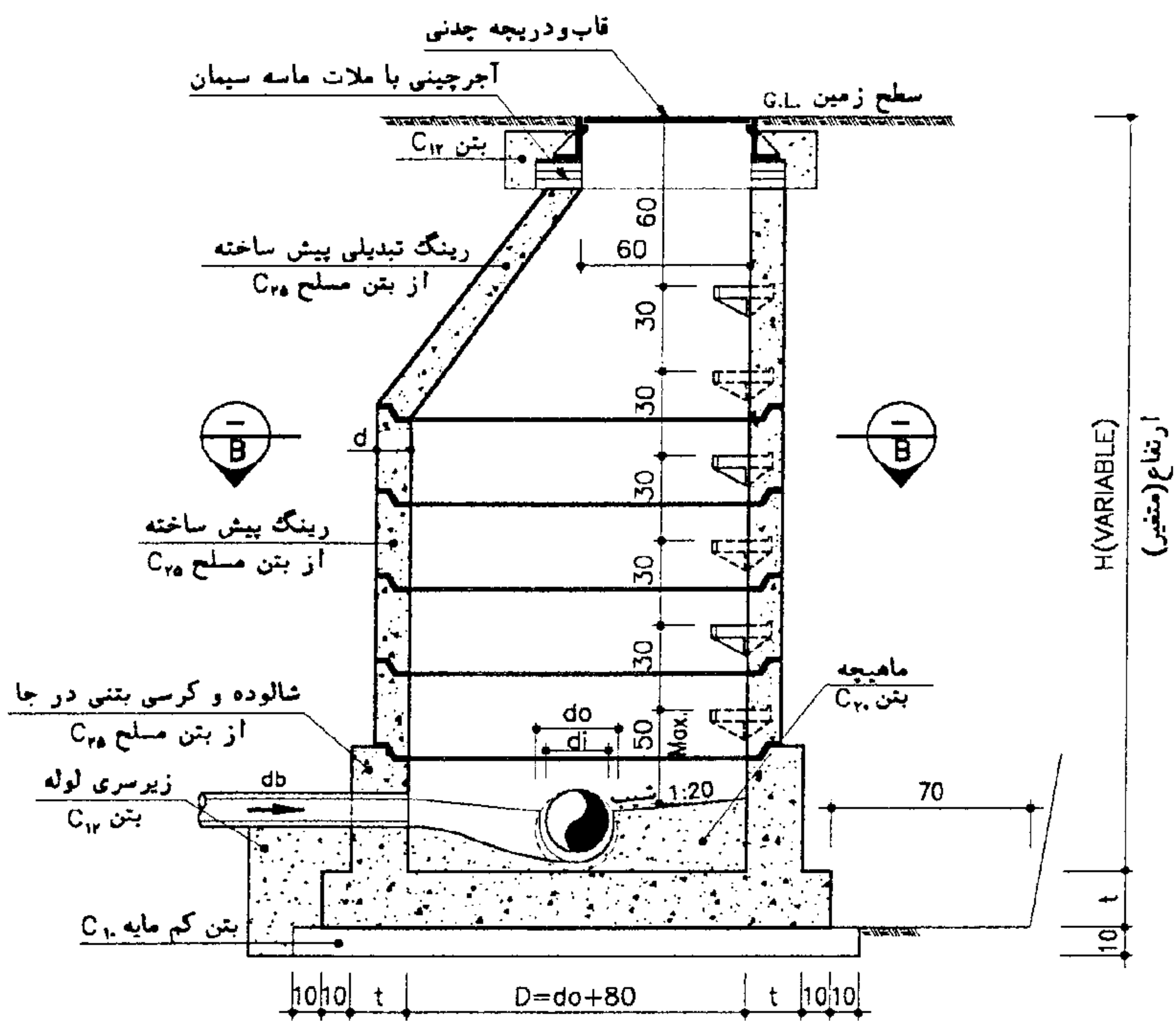
SECTION B-B N.T.S
