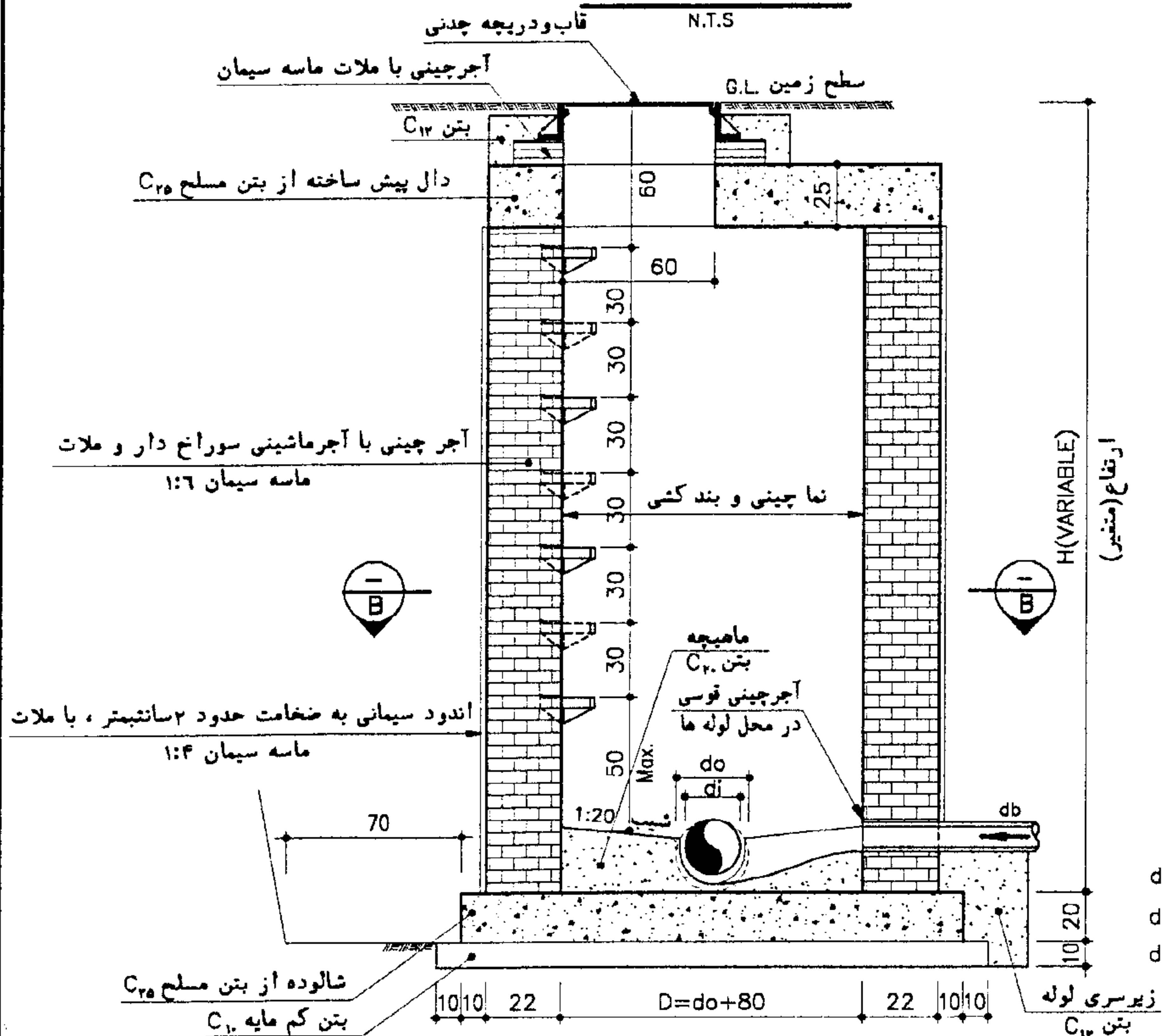
SECTION A-A
