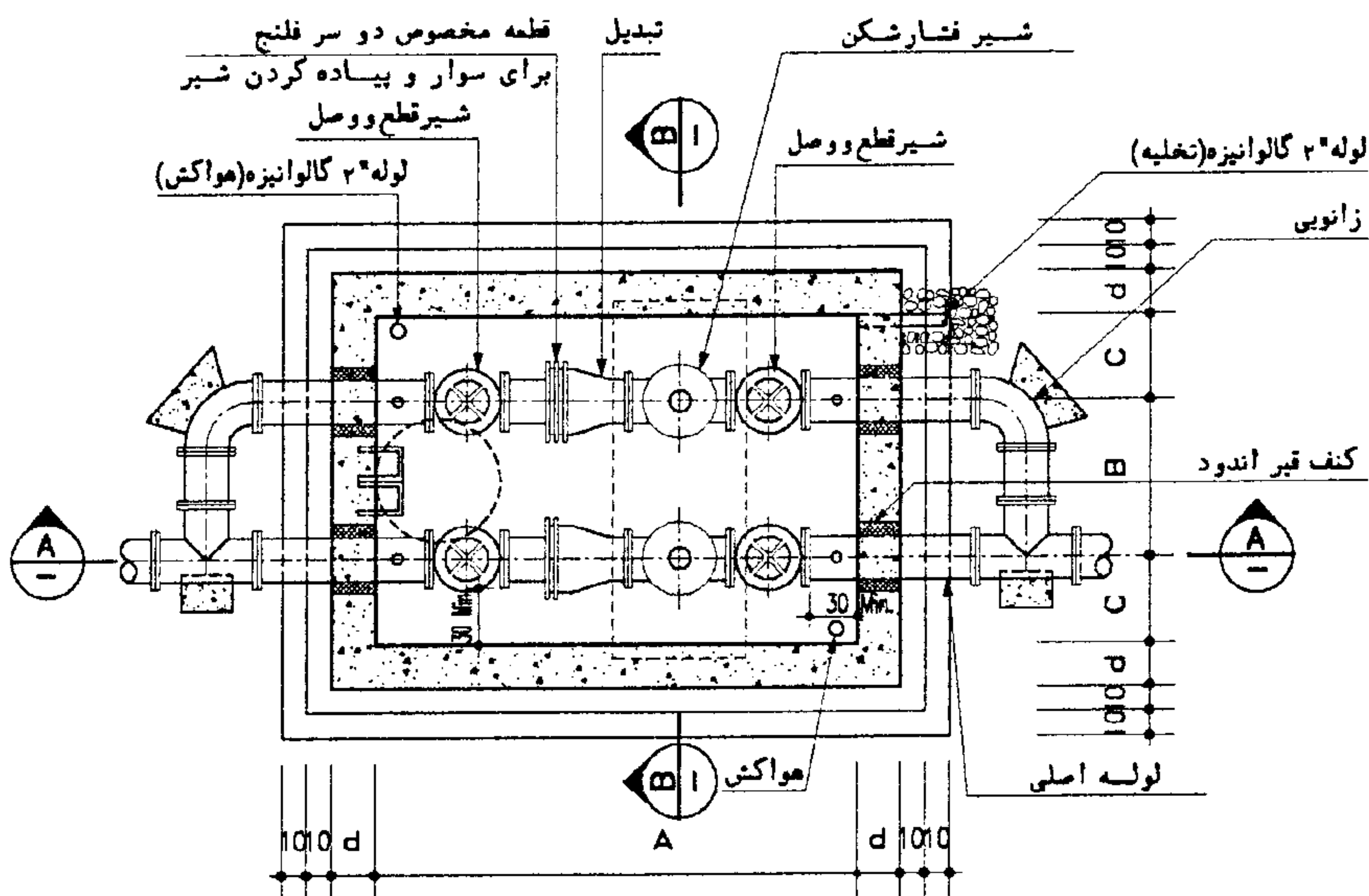
PLAN N.T.S
