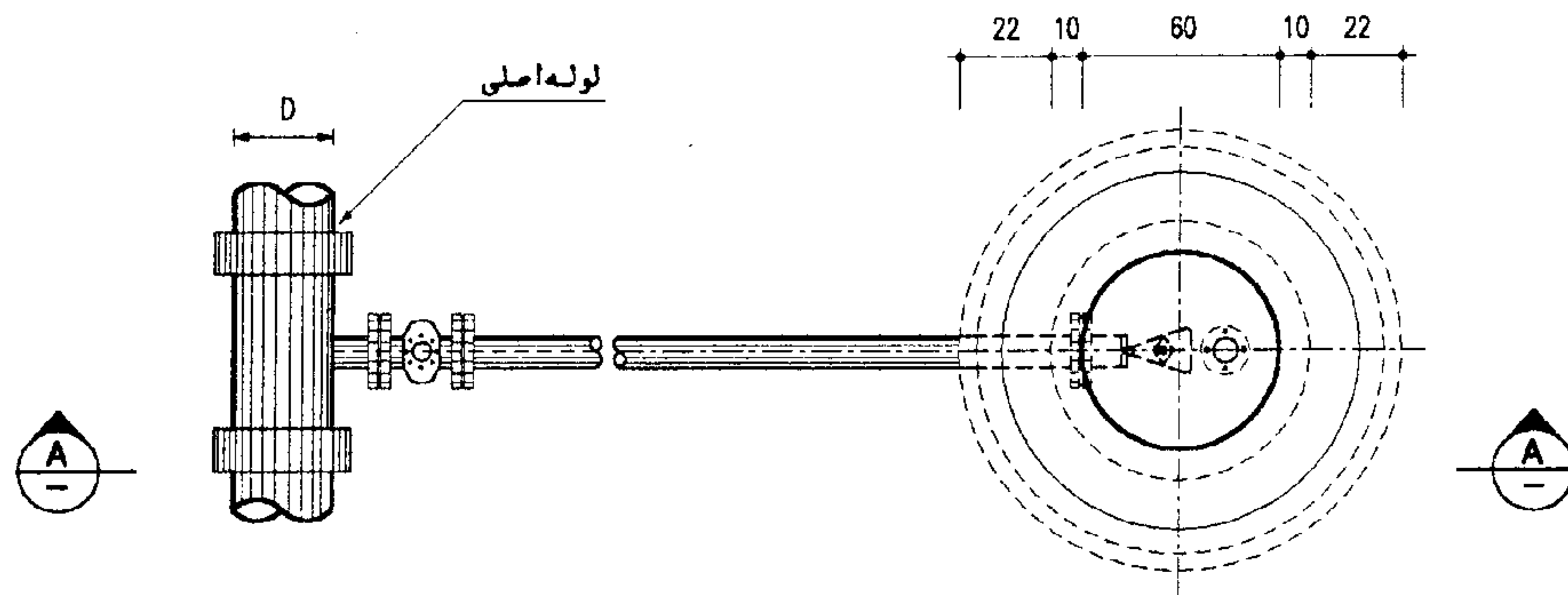
PLAN N.T.S
