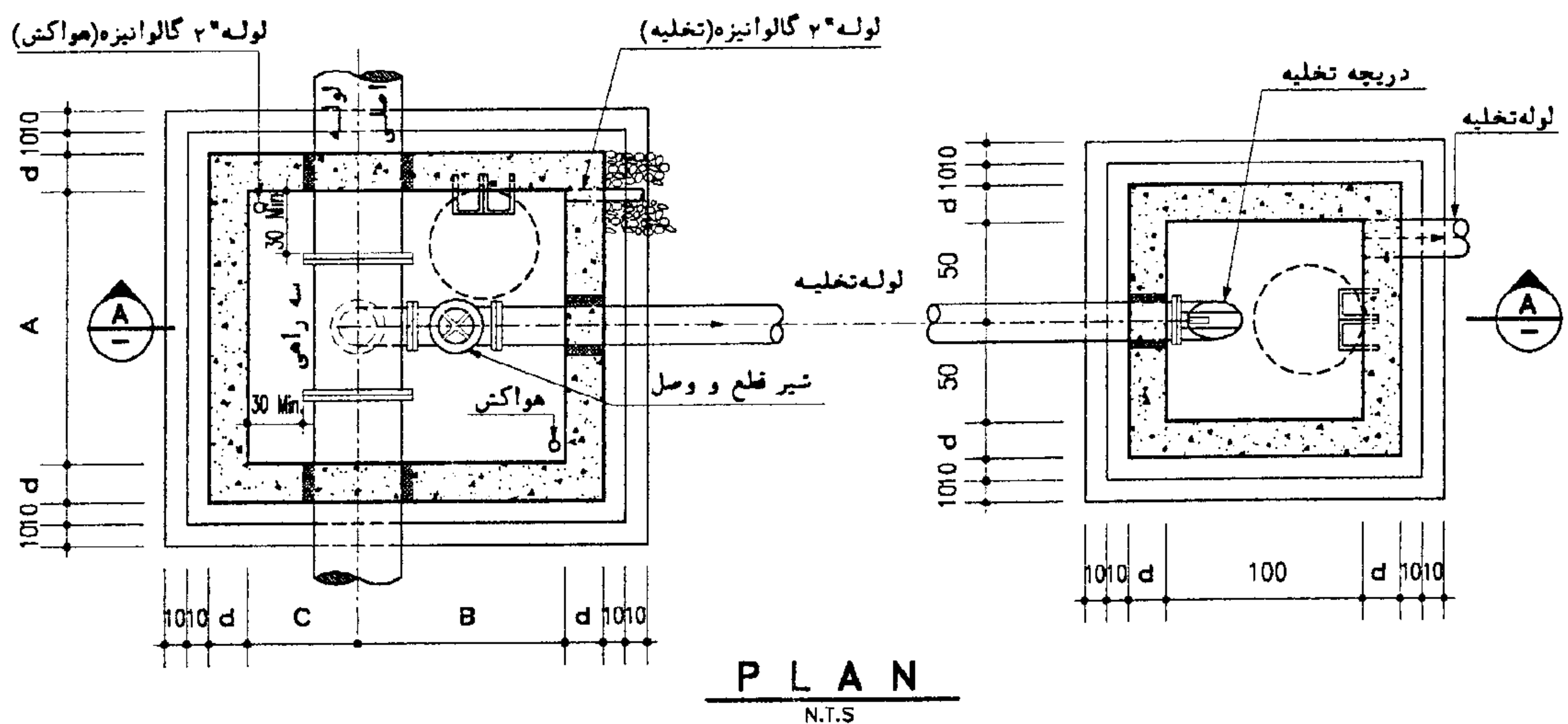
حوضچه شیر تخلیه آب
