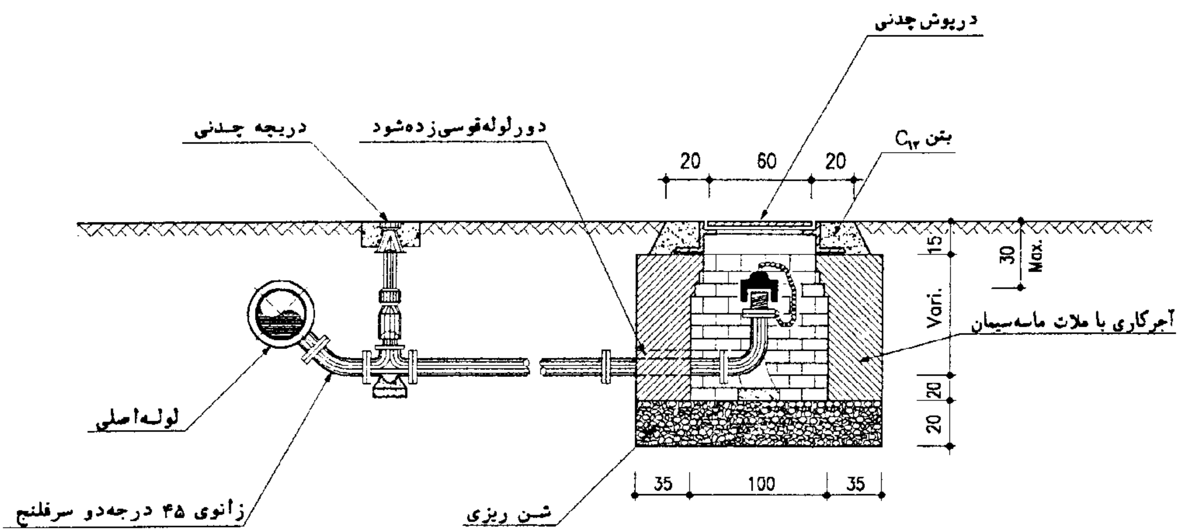
PLAN N.T.S
