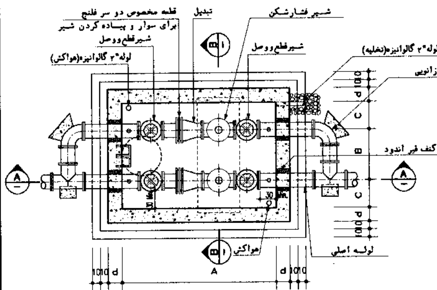
PLAN N.T.S
