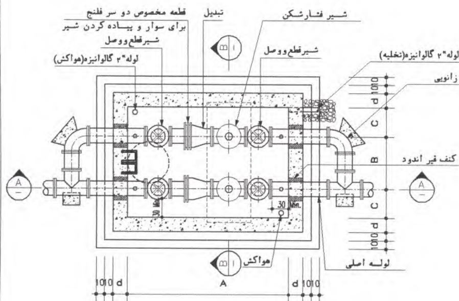
PLAN N.T.S
