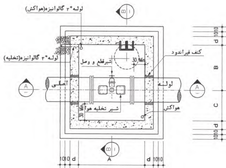
PLAN N.T.S
