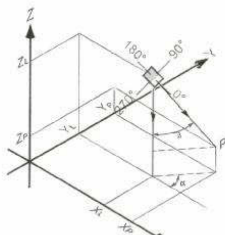
شکل ۲-۱۰: زوایای تابش
