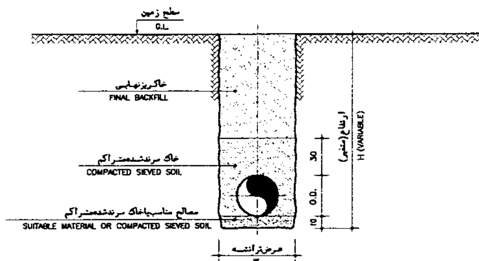
مقطع ترانسه TRENCH SECTION N.T.S
