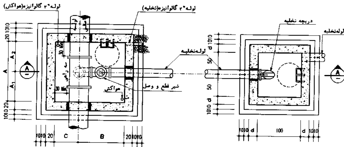
PLAN N.T.S.
