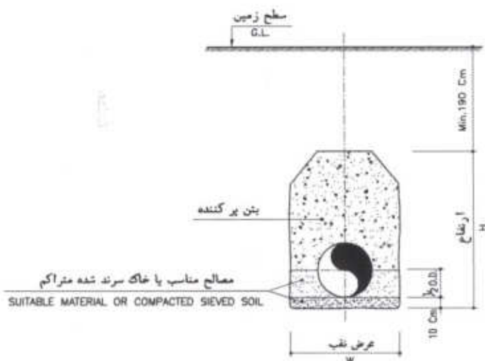
مقطع نخب
