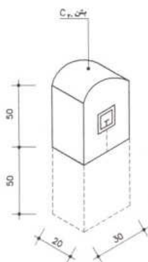
پایه بتنی مشخص کننده محل متعلقات خطلوله
