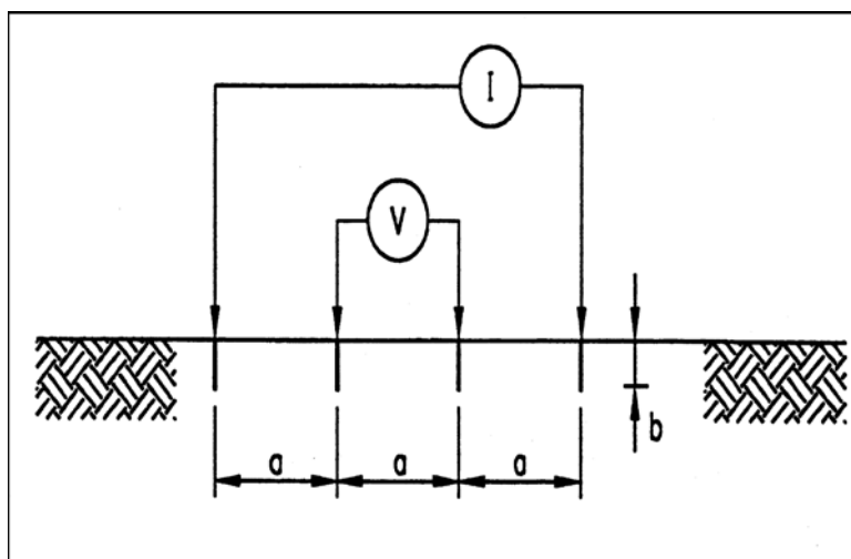
شکل ۲-۲: روش چهار نقطه‌ای ونر برای اندازه‌گیری مقاومت زمین
