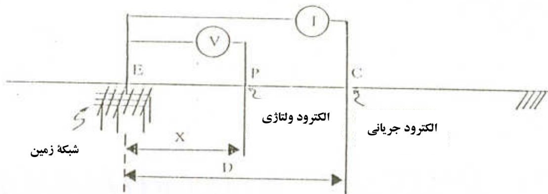
شکل ۳-۱: مدار آزمون اندازه‌گیری مقاومت زمین
