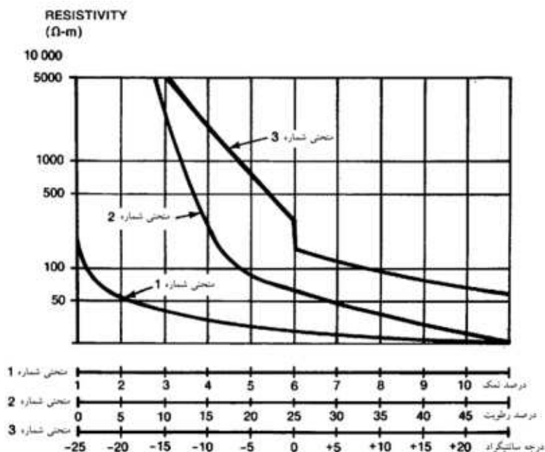
شکل (۲-۳): اثر رطوبت، دما و نمک بر روی مقاومت خاک
