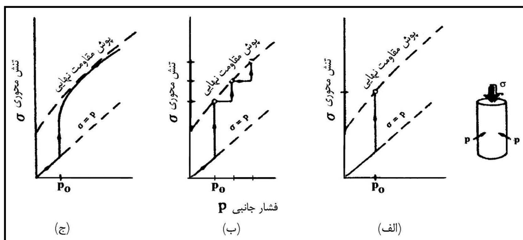
شکل ۲-۱۶- روش‌های مختلف آزمایش مقاومت فشاری سه محوری سنگ
