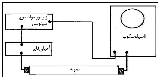
شکل ۱-۷- نحوه قرارگیری فرستنده و گیرنده روی نمونه در آزمایش بسامد تشدید
