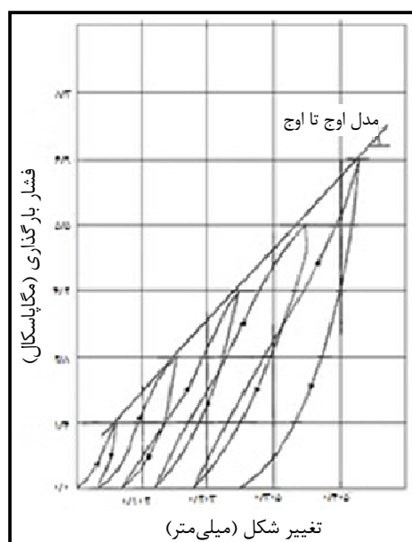
شکل ۳-۹- تغییر شکل سطح سنگ به صورت تابعی از فشار بارگذاری
