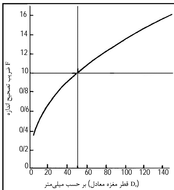
شکل 2-10- ضریب تصحیح شاخص بار نقطه‌ای بر حسب قطر مغزه معادل
