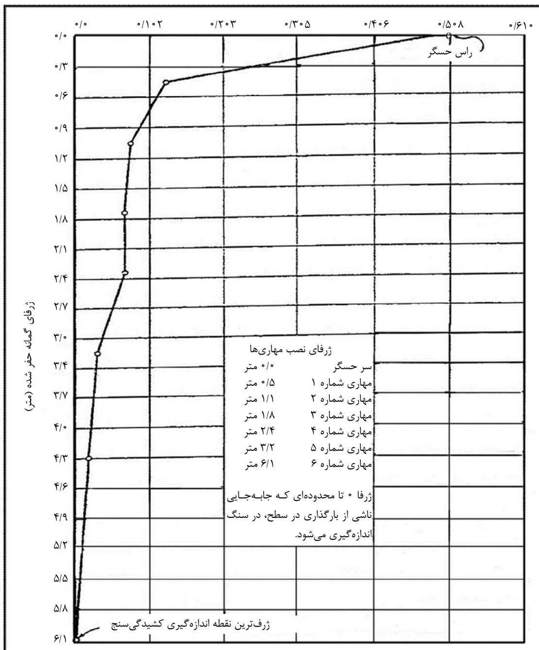
شکل ۳-۵- جابه‌جایی محوری بر حسب ژرفا، نسبت به ژرف‌ترین نقطه درگیر، زیر فشار ۶/۹ مگاپاسکال
