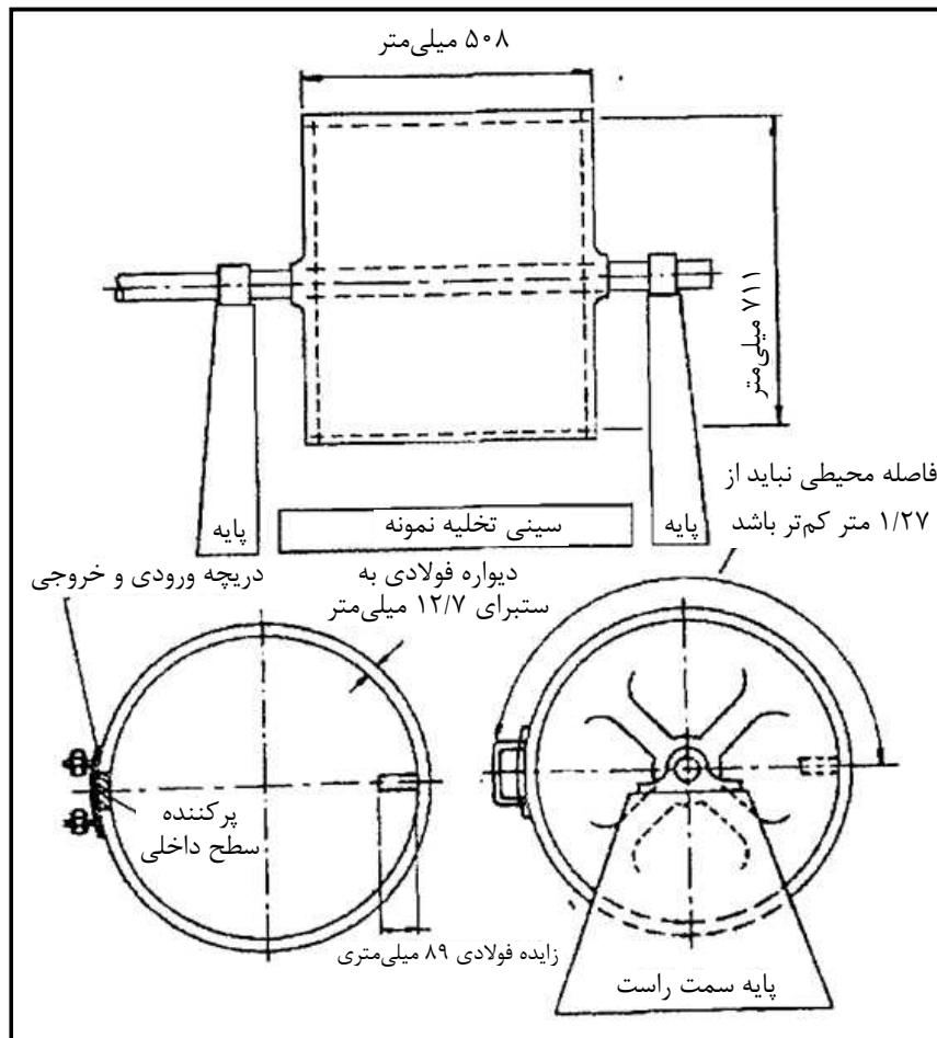
شکل ۱-۳- نمای شماتیک دستگاه لس آنجلس
