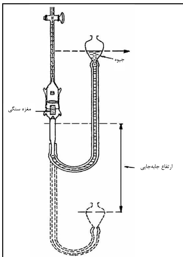
شکل 1-1- دستگاه تخلخل‌سنج با روش جابه‌جایی جیوه، نوع واشبرن - بونتینگ 1
