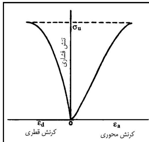
شکل ۲-۱- منحنی تنش محوری بر حسب کرنش‌های محوری و قطری
