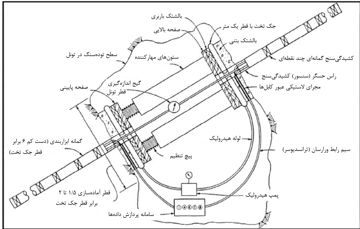
شکل ۱-۳- نحوه قرارگیری تجهیزات در داخل فضای زیرزمینی در آزمایش بارگذاری صفحه‌ای [۲]
