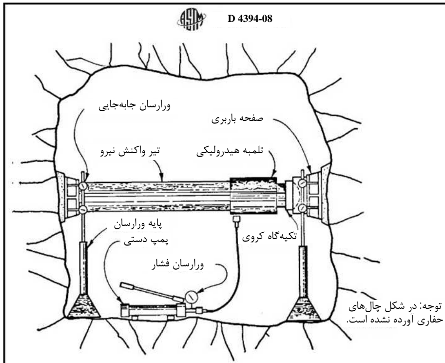
شکل 3-2-3- نحوه قرارگیری تجهیزات در آزمون بارگذاری صفحه‌ای صلب
