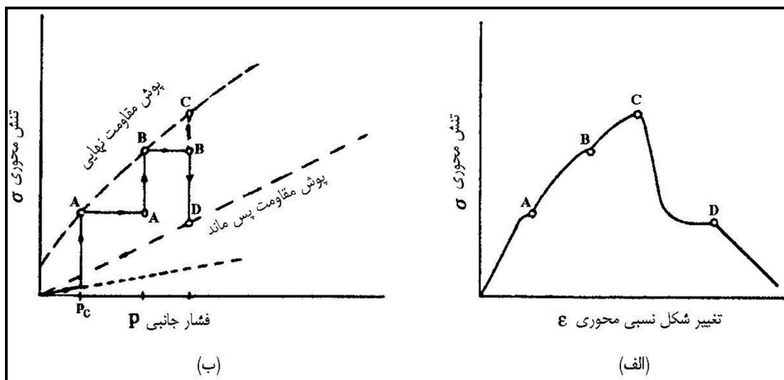
شکل ۲-۱۹- نمودار شماتیک نتیجه‌های آزمایش به روش ب (شکست چند مرحله‌ای)
