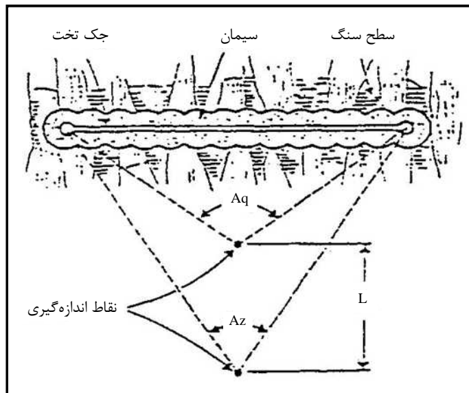
شکل ۳-۱۴- اصطلاحات هندسی در روش جک مسطح
