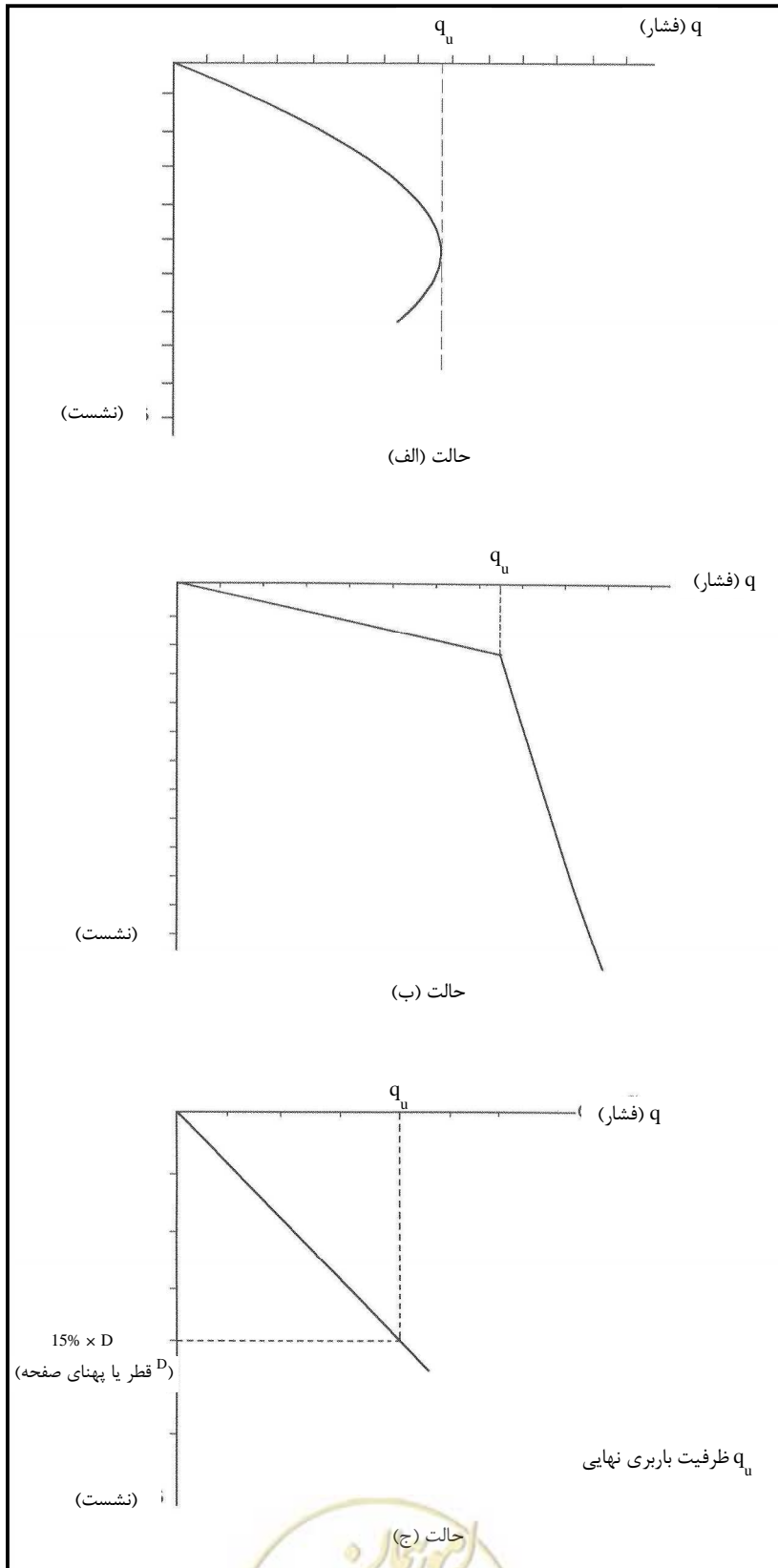
شکل ۳- نمودار فشار - نشست
