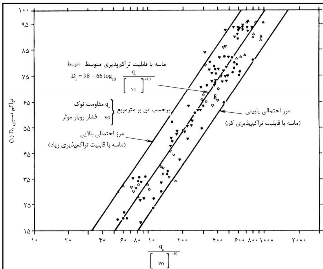
شکل ۳-۶- رابطه میان D_r و q_c برای ماسه عادی تحکیم یافته کوارتزی (دارای منشای کوارتزی) [۳]
