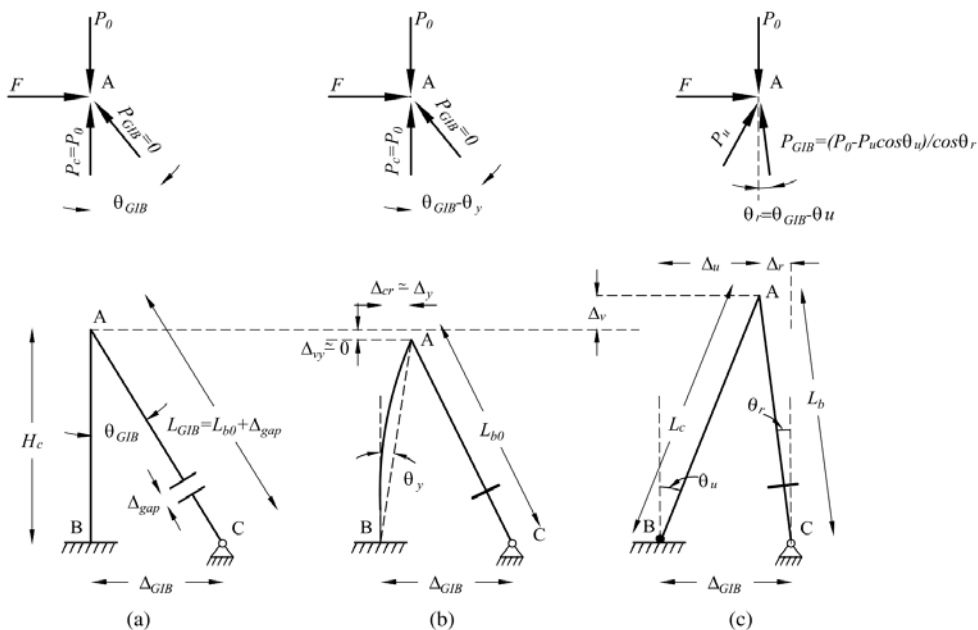
شکل ۴-۱ مکانیزم سیستم GIB: (a) حالت سکون، (b) حالت جاری شدن ستون، (c) حالت نهایی ستون
