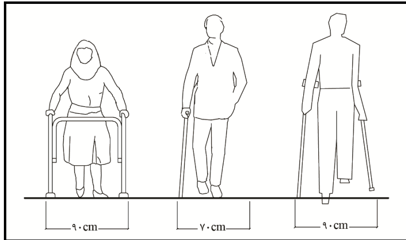
شکل ۱-۱۴- فضای مورد نیاز برای عبور افراد با سایر وسایل کمک حرکتی
