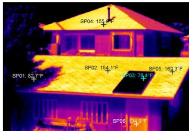
شکل ۲- میزان اتلاف انرژی از طریق سقف در ساختمان با سقف سبز
