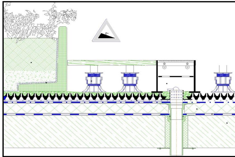
شکل ۲-۹- جزئیات نصب کفیوش در بام سبز
