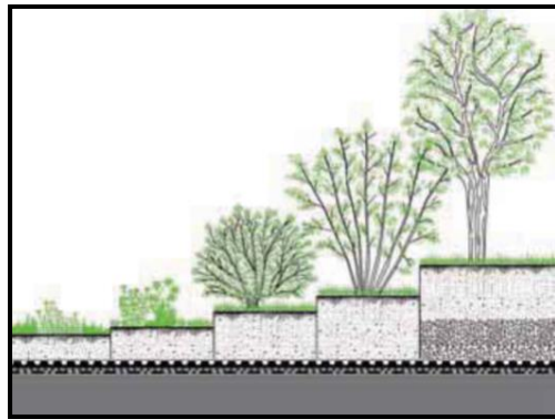
شکل ۱-۱- ضخامت لایه خاک و نوع گیاهان انواع بام سبز
