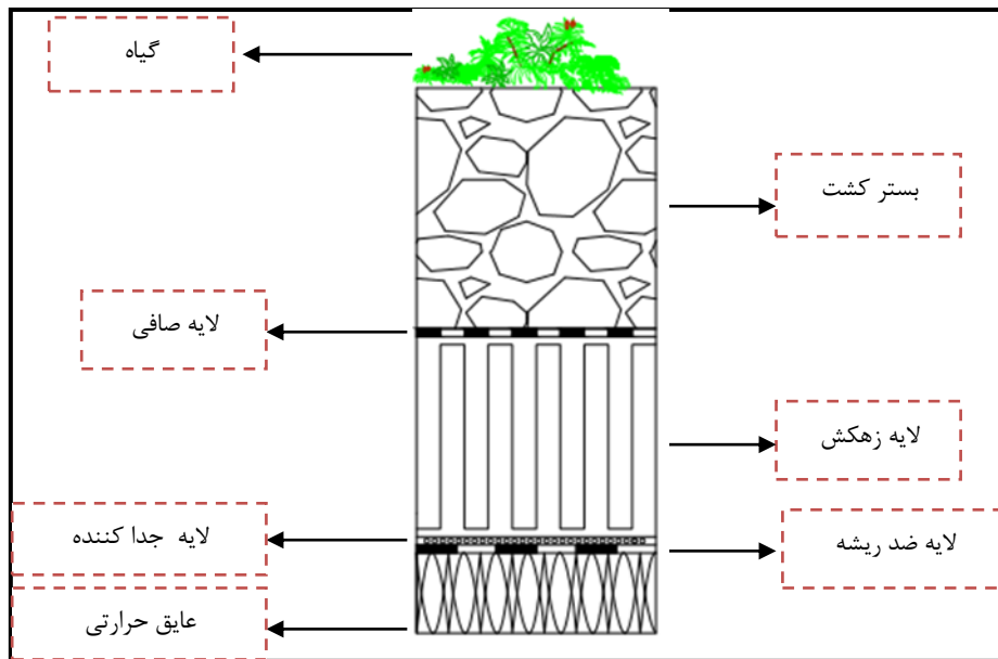
شکل ۱-۸-۱- اجزای بام سبز و مراحل اجرای آن
