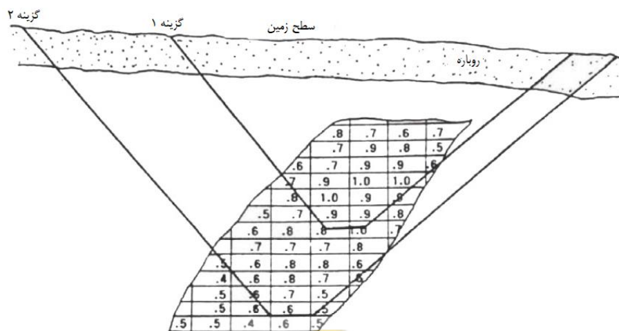
شکل ۴-۵- مقطع عرضی از معدن که کف معدن در ماده معدنی قرار دارد.
