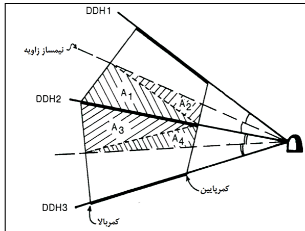
شکل ۴-۱۶- تعیین عیار متوسط پهنه‌های استخراجی به کمک چال‌های بادبزی
