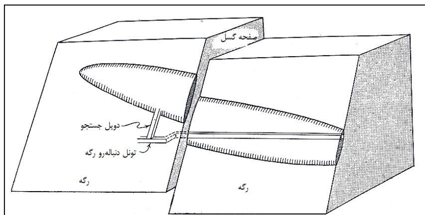
شکل ۵-۷- حفر دوینل برای یافتن بخش قطع شده ماده معدنی به وسیله یک گسل پرسیب
