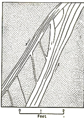
شکل ۵-۱۱- شکستگی‌های برشی در سنگ‌های اطراف گسل
