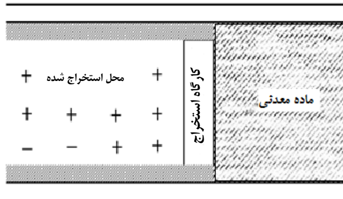
شکل ۱-۴- کارگاه استخراج
