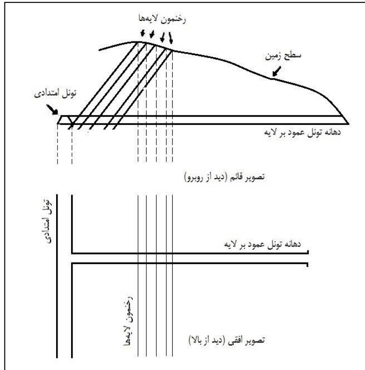
شکل ۲-۷- تونل امتدادی
