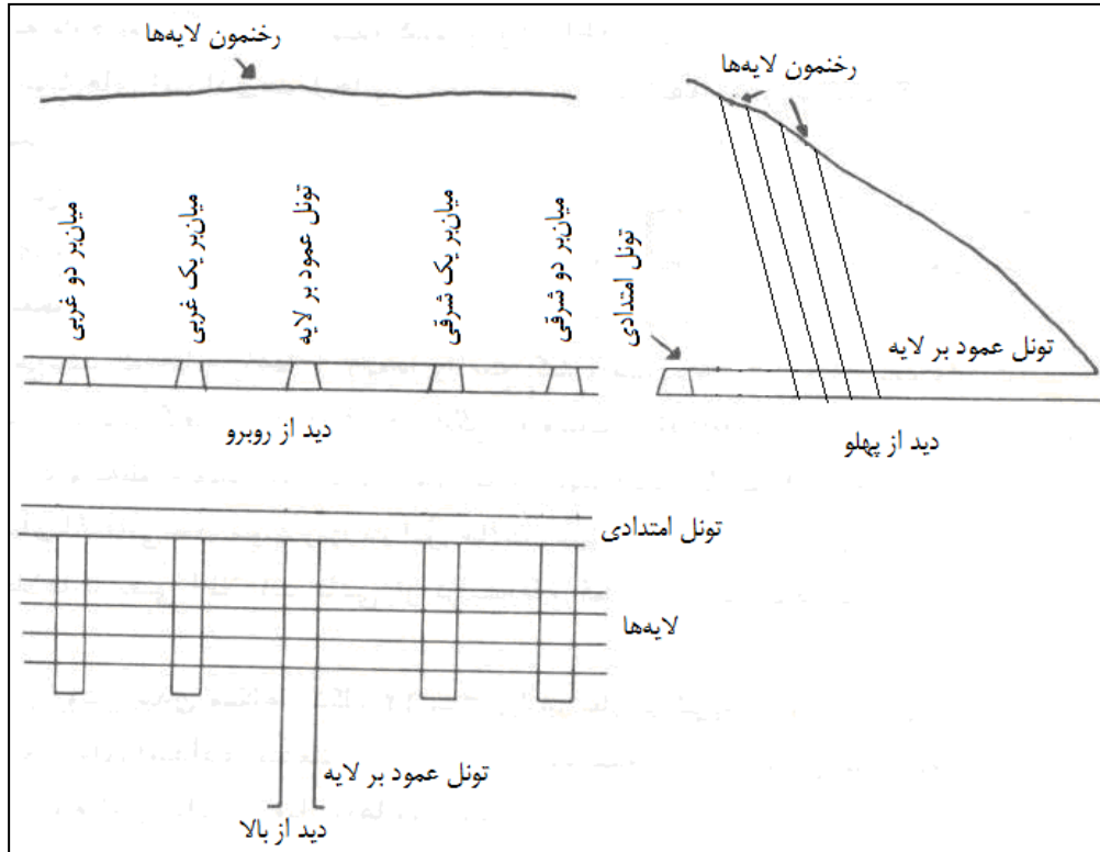
شکل ۲-۱۲- موقعیت میان‌برها
