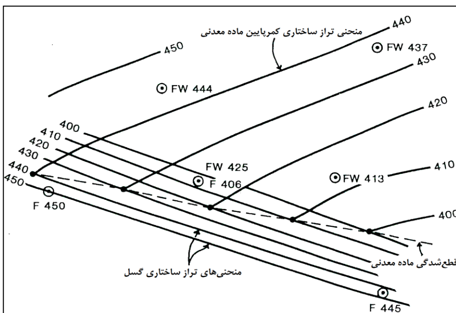
شکل ۴-۹- منحنی های تراز ساختاری کمربالین یک توده معدنی همراه با منحنی های گسلی که آن را قطع کرده است.
