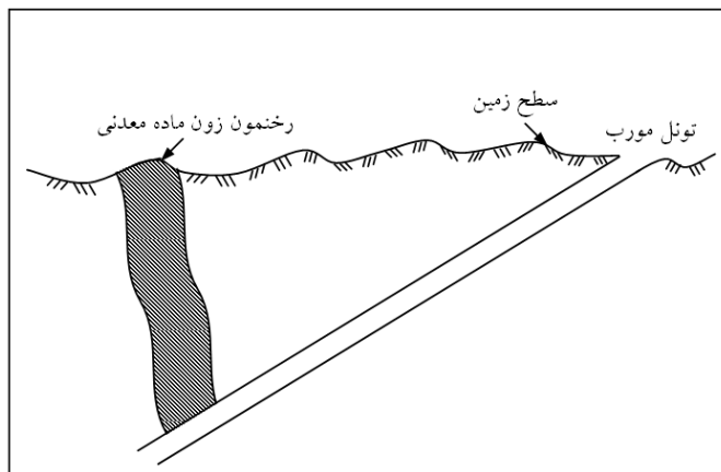
شکل ۱-۲- تونل مورب
