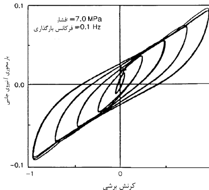
شکل (ت-2-10): حلقه‌های نیرو- تغییر شکل برای تکیه‌گاه لاستیکی با میرایی زیاد
