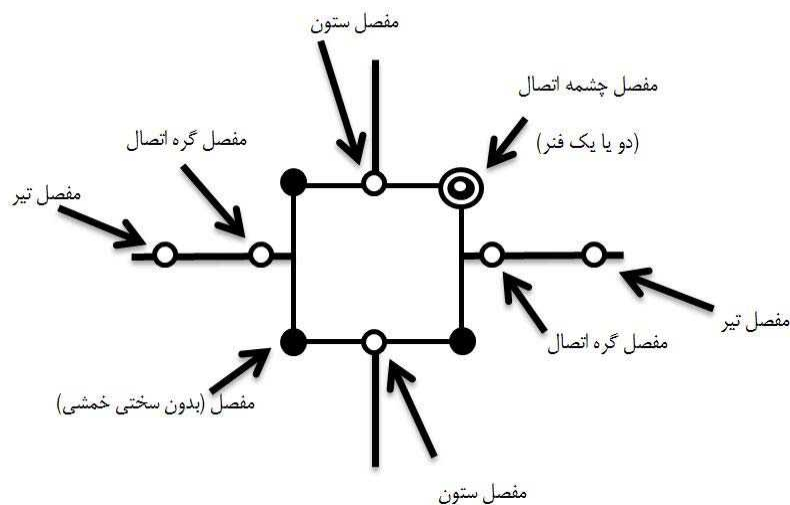
شکل (ت 5-1): نحوه مدلسازی چشمه اتصال
