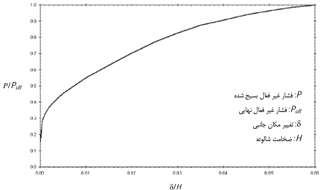
شکل (ت 4-5): نمودار میزان بسیج فشار مقاوم خاک.
