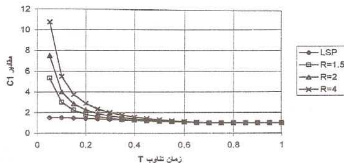
شکل (ت 3-5) - مقدار C_1 برحسب زمان تناوب اصلی سازه
