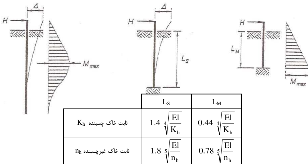
شکل (ت 5-10): مدل طره‌ی معادل برای تحلیل شمع‌ها
