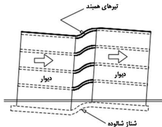
شکل ت 11-12: تیرهای همبند
