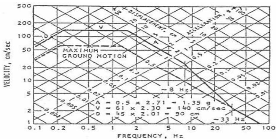
شکل (ت 1-2) : طیف نرمال شده برای PGA=0/5g و میرایی 5 %
