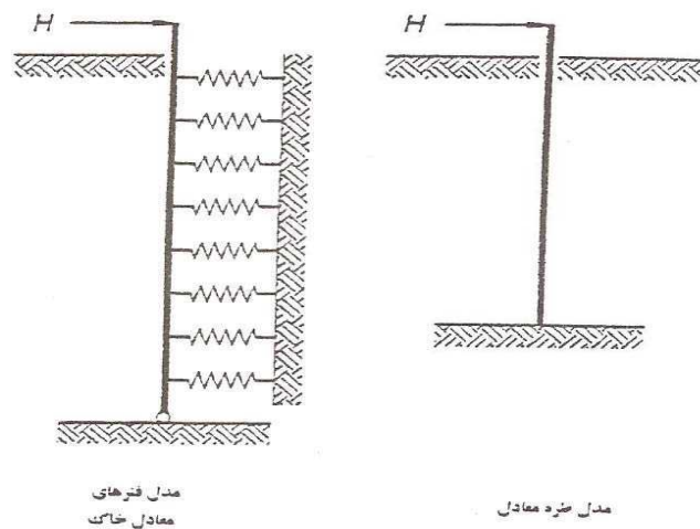
شکل (ت 5-9) : مدل‌های تحلیلی شمع‌ها
