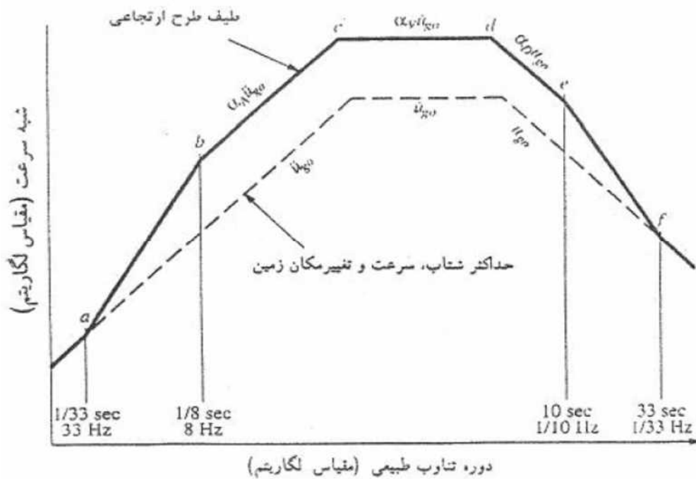
شکل (ت 1-1): طیف نرمال شده (نیومارک - هال)
