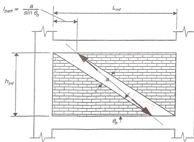
شکل (ت 7-8): تخمین نیروهای وارده بر تیرها
