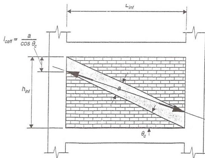
شکل (ت-8-6): تخمین نیروهای اعمال شده به ستونها
