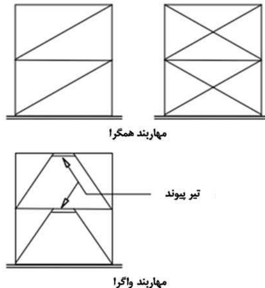
شکل ت 11-7: انواع سیستم مهاربندی
