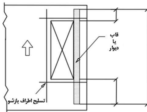
شکل ت 11-13: دیافراگم
