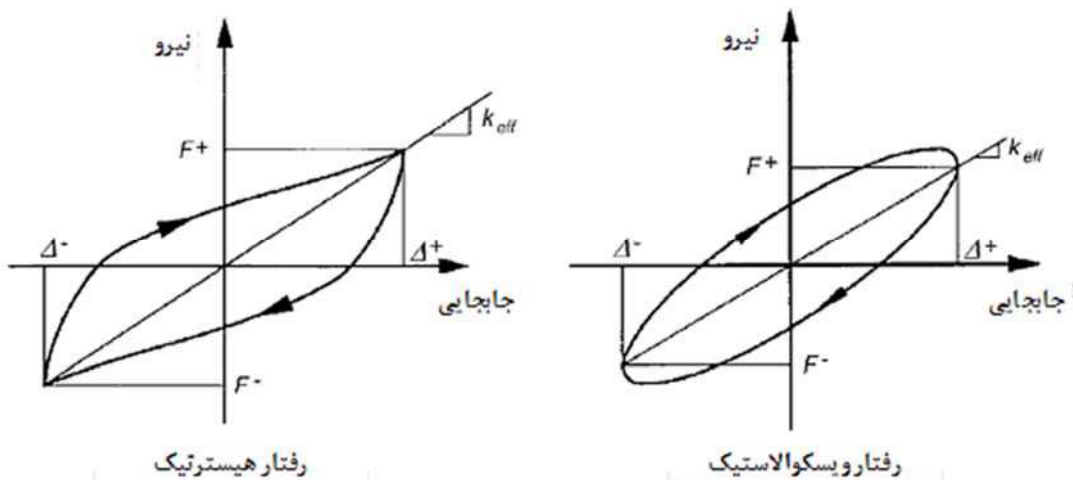
شکل (ت 10-7): سختی مؤثر جداسازهای لرزه‌ای با رفتارهای چرخه ای متفاوت
