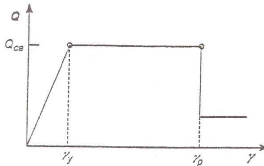
شکل (ت 5-8): تعریف ظرفیت تغییر شکلی تیر پیوند
