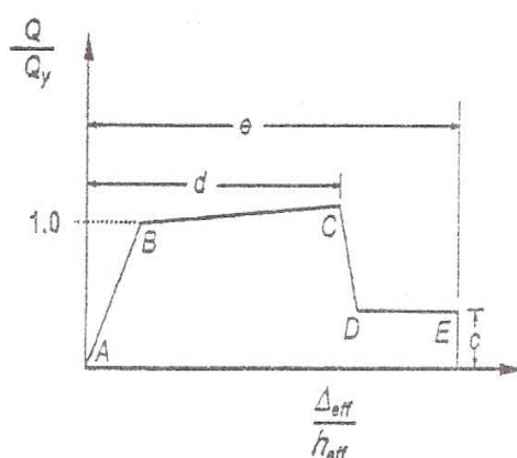
شکل (ت 8-8): رابطه ی کلی نیرو - تغییر مکان برای دیوارهای مصالح بنایی
