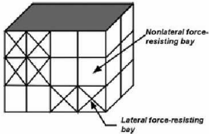
شکل (ت 2-3)-انقطاع سیستم باربر لرزه ای در صفحه
