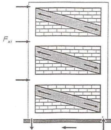
شکل (ت 8-4): شبیه سازی با دستکهای فشاری واگرا
