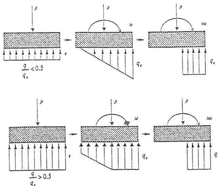
شکل (ت-4-4): توزیع ایده‌آل فشار در کف شالوده‌های صلب در معرض لنگر واژگونی
