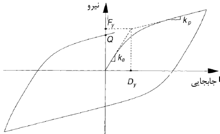
شکل (ت 10-1): منحنی نمونه نیرو - تغییر شکل برای تکیه گاه لاستیکی - سربی
