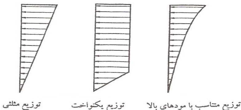
شکل (ت 3-6) - حالت‌های مختلف توزیع نیروی جانبی
