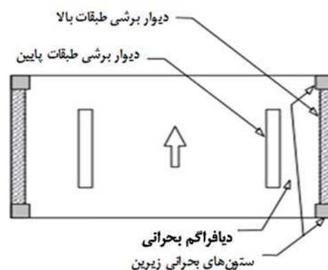
شکل ت 11-6: ناپیوستگی در ارتفاع در خارج از صفحه
