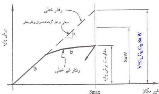
شکل (ت 3-4) - اختلاف روش خطی و غیر خطی
