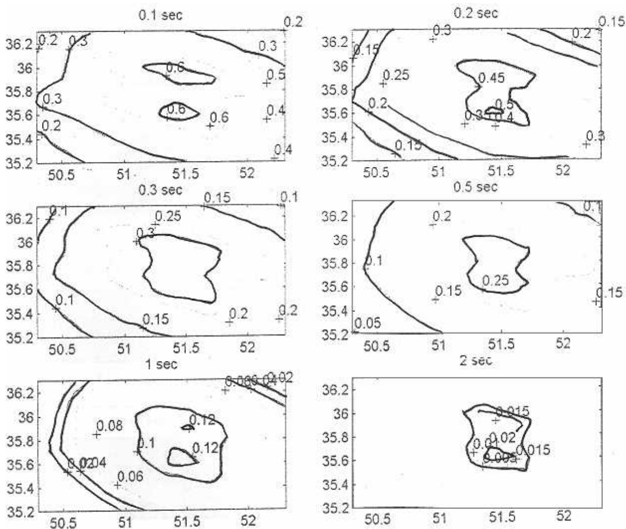
شکل (ت 1-6): نقشه‌های شتاب طیفی برای زمان تناوب 0/1، 0/2، 0/3، 0/5، 1 و 2 ثانیه برای ناحیه تهران
