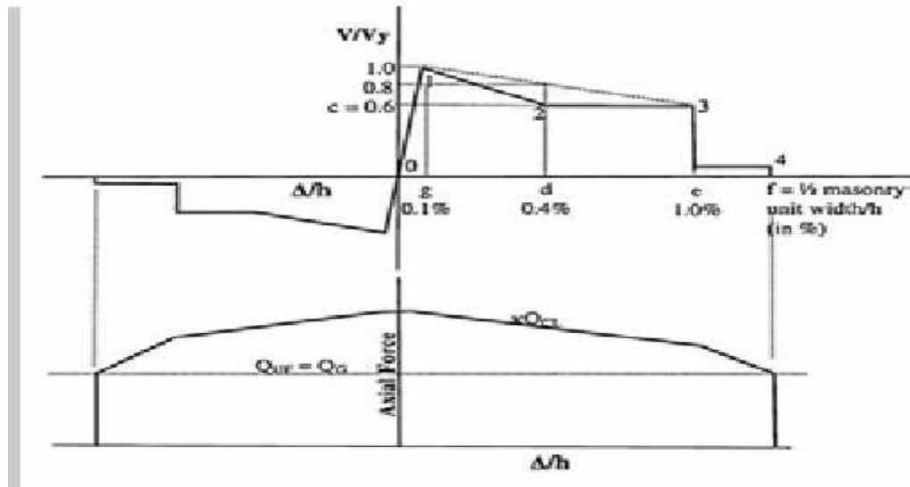
شکل ت 7-6-مود خرابی لغزش سطوح اتصال
