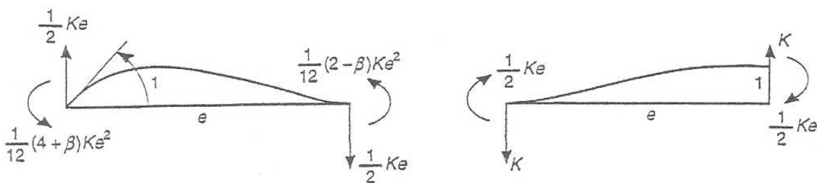
شکل (ت 5-5): ضرایب سختی برای تیر پیوند به طول e
