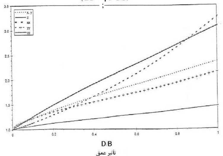
شکل (ت-3-4): اثرات شکل و عمق شالوده
