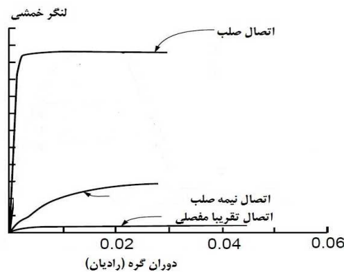
شکل (ت 2-5): مقایسه رفتار اتصالات صلب و نیمه صلب
