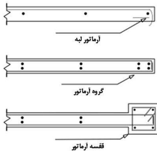
شکل ت 11-11: آرماتور گذاری دیوار برشی
