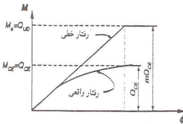
شکل (ت 3-10) - رفتار یک عضو تغییر شکل کنترل
