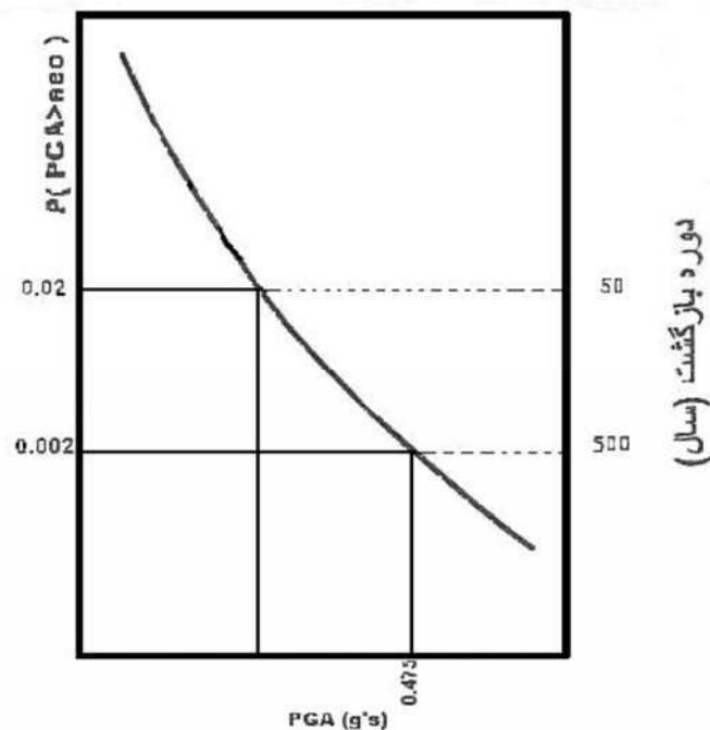
شکل (ت 1-10) : منحنی خطر براساس احتمال وقوع (یا دوره بازگشت به سال)
