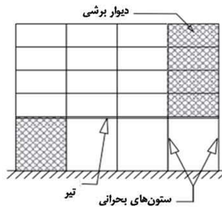
شکل ت 11-5: ناپیوستگی قائم
