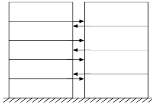
شکل ت 11-3: طبقات با دیافراگم های غیر هم تراز
