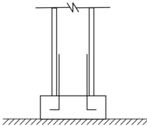
شکل ت 11-10: اتصال ستون بتنی در شالوده
