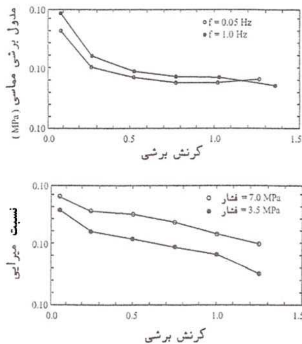
شکل (ت 10-3): مدول برشی مماسی و نسبت میرایی مؤثر تکیه‌گاه لاستیکی با میرایی زیاد
