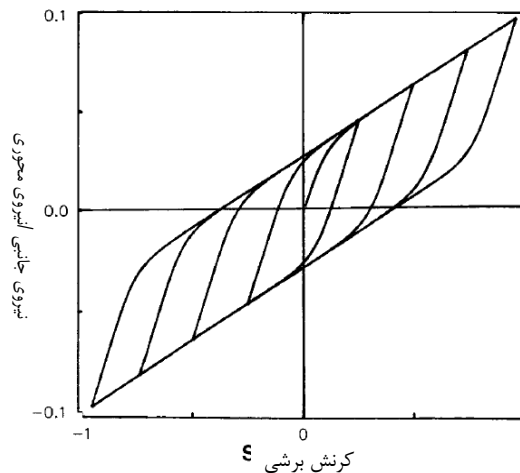
شکل (ت 10-4): نتایج تحلیلی حلقه‌های نیرو - تغییر مکان تکیه‌گاه لاستیکی بامیرایی زیاد
