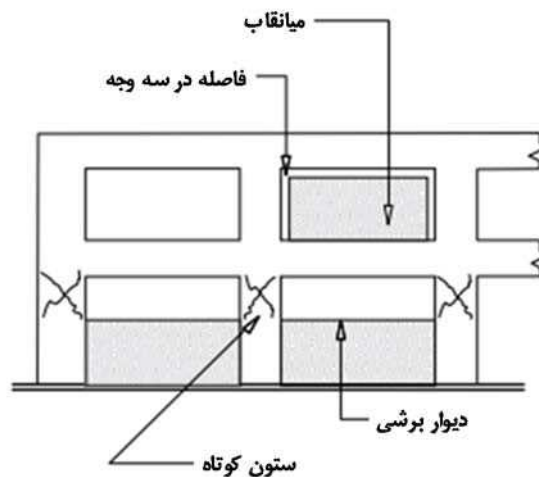
شکل ت 11-9: میانقاب ها
