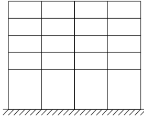
شکل ت 1-11: ساختمان با ارتفاع زیاد در طبقه اول
