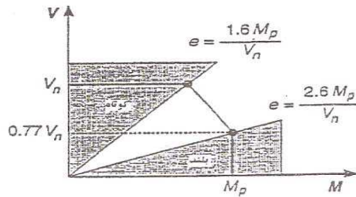
شکل (ت 5-6): اندرکنش برش و خمشی
