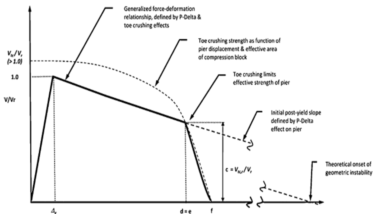
شکل ت 7-5- منحنی نیرو-تغییر شکل دیوارهای بنایی غیر مسلح
