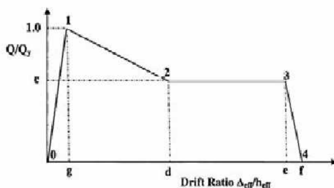
شکل ت-7-1- رابطه نیرو- تغییر شکل اعضای تغییر شکل کنترل
