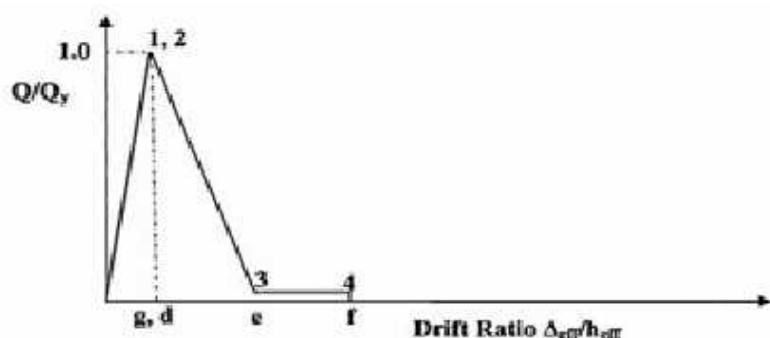
شکل ت-7-2- رابطه نیرو- تغییر شکل اعضای نیرو کنترل
