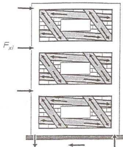
شکل (ت 8-5): شبیه سازی با دستکهای فشاری - میانقاب‌های دارای بازشو
