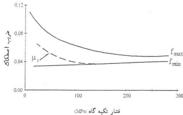
شکل (ت 10-6): پارامترهای مدل تکیه‌گاه لغزشی اصطکاکی از جنس PTFE در تماس با فولاد صیقلی در دمای معمولی
