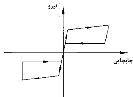
وسيله اصطکاکی-فنری با قابلیت تامين
