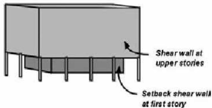
شکل (ت 3-3)-انقطاع سیستم باربر لرزه ای در خارج از صفحه
