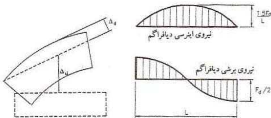
شکل (ت-3-1) - تعریف تغییر شکل دیافراگم و نحوه توزیع نیروی اینرسی در آن
