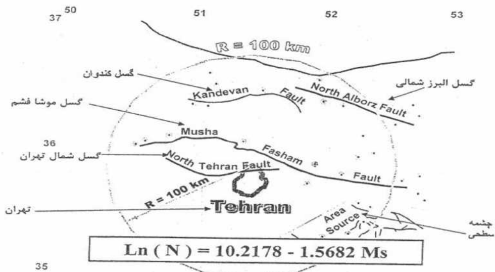
شکل (ت 9-1): تعیین گسلهای فعال به شعاع 100 کیلومتر در اطراف تهران
