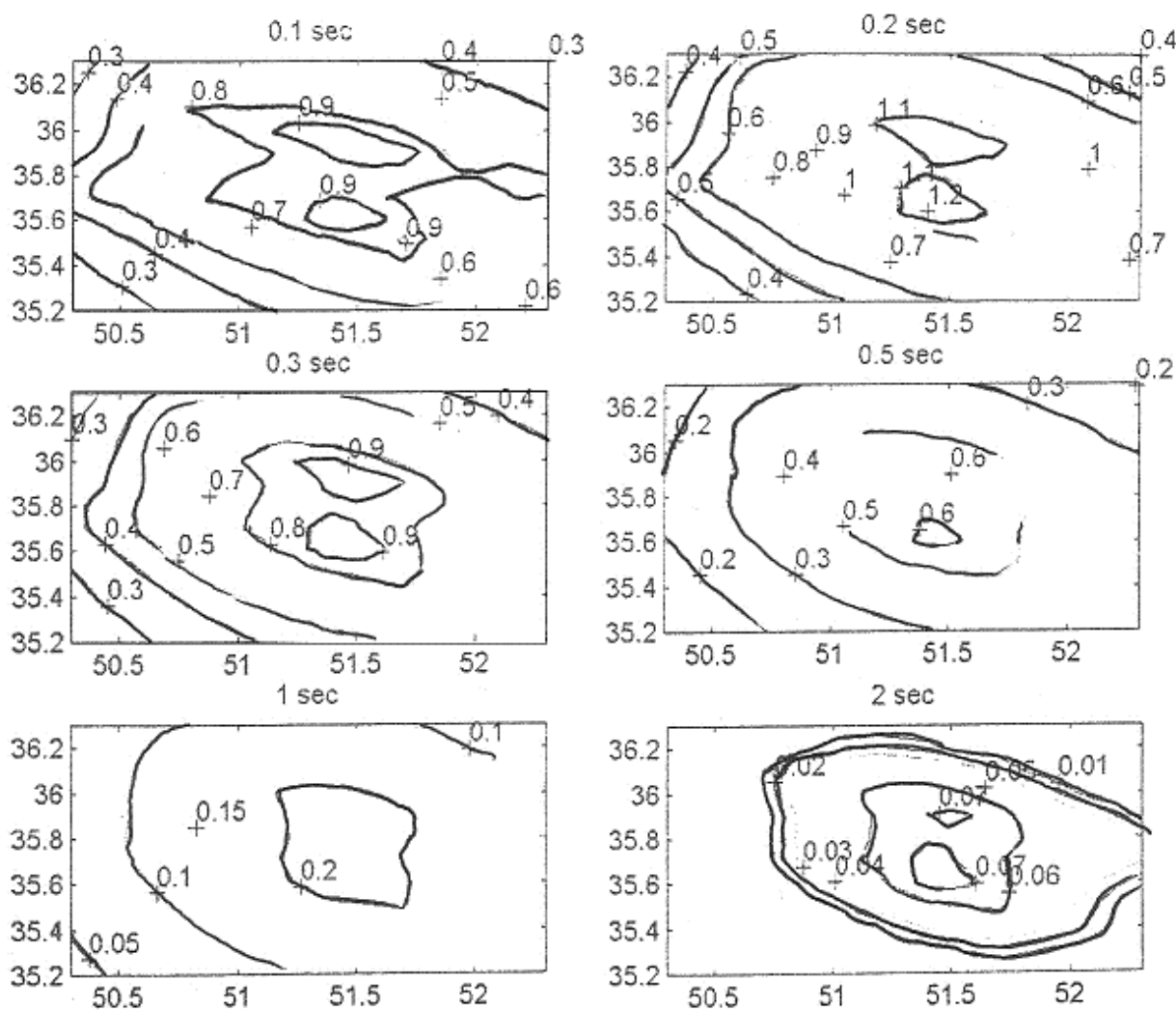
شکل (ت 5-1): نقشه‌های شتاب طیفی برای زمان تناوب 0/1، 0/2، 0/3، 0/5، و 2 ثانیه برای ناحیه تهران (مؤلفه افقی - رابطه ایران - 1999) در دوره بازگشت 475 سال
