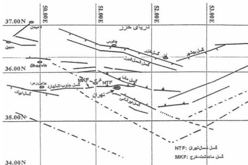
شکل (ت 3-1): گسلهای بنیادی ناحیه تهران
