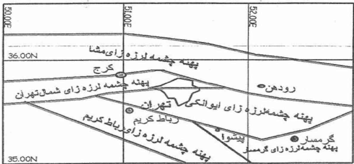
شکل (ت-4): پهنه های چشمه های لرزه زا در ناحیه تهران
