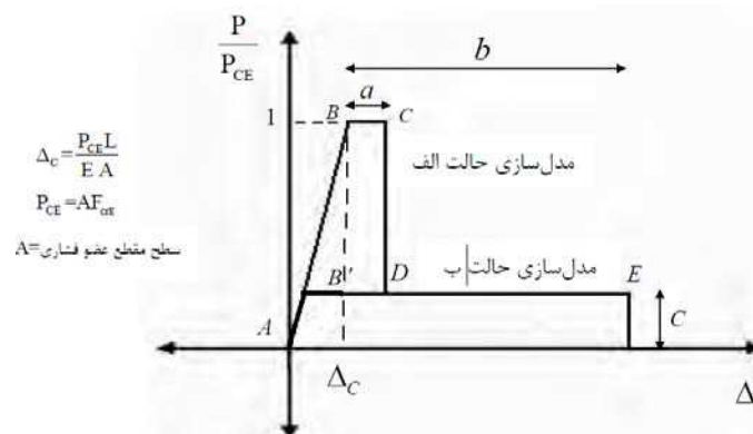
شکل (ت3-5): منحنی نیرو- تغییر شکل برای مهاربند فشاری در دو حالت الف و ب
