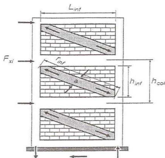
شکل (ت 3-8): شبیه سازی با دستکهای فشاری همگرا
