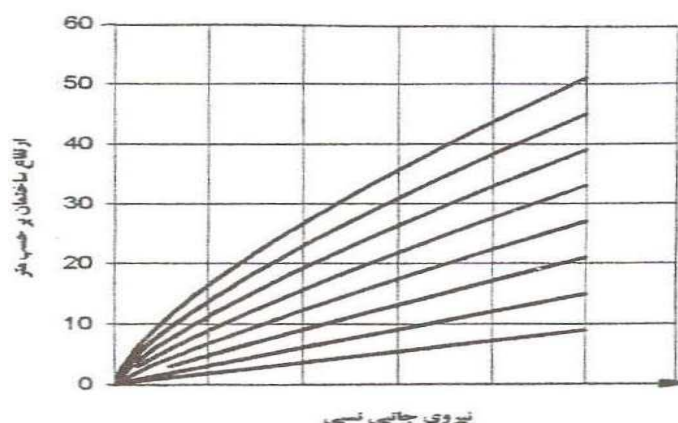
شکل (ت 3-7) - توزیع نیروی جانبی را برای قاب خمشی بتنی با فرض توزیع یکنواخت جرم در ارتفاع
