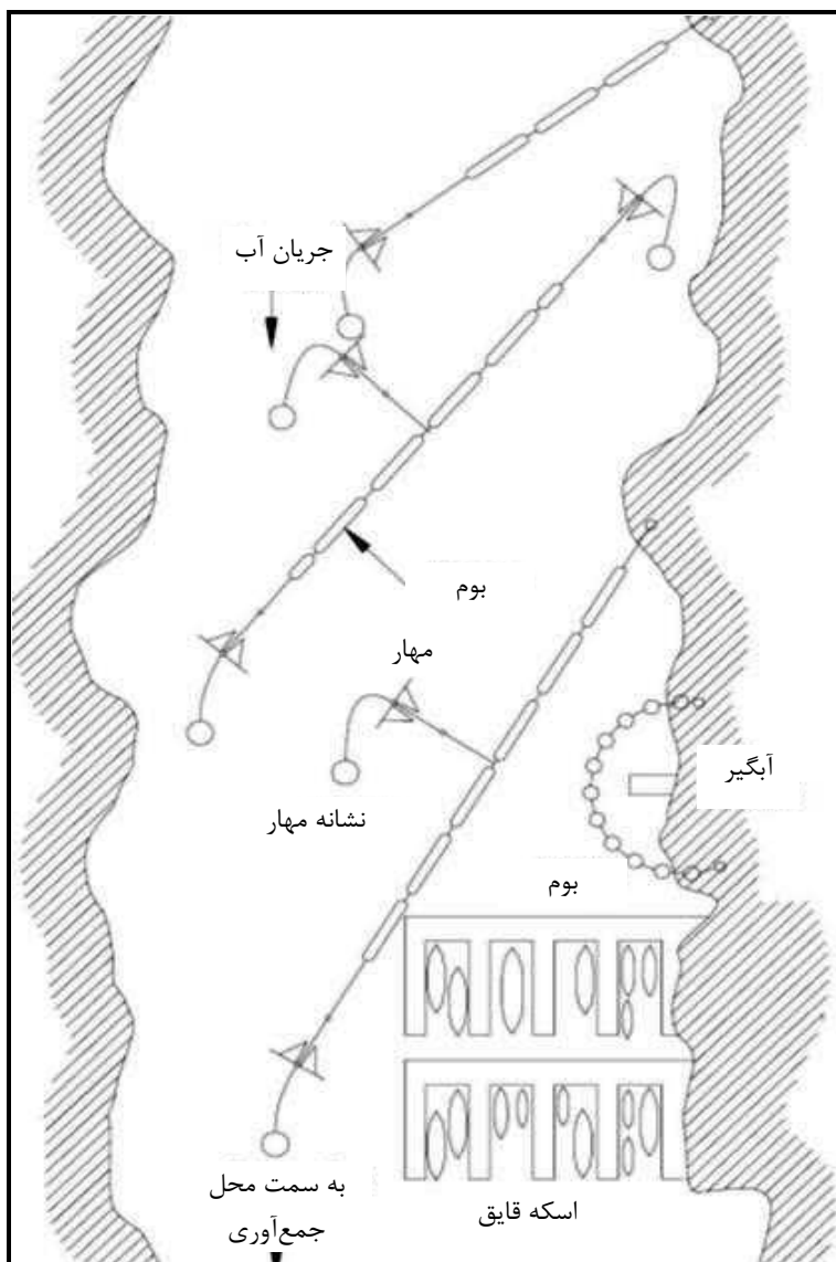
شکل پ.۴-۲۳- نمای از به کارگیری بوم‌ها برای تغییر جهت مسیر نفت و محدودسازی نفت بر سطح آب
