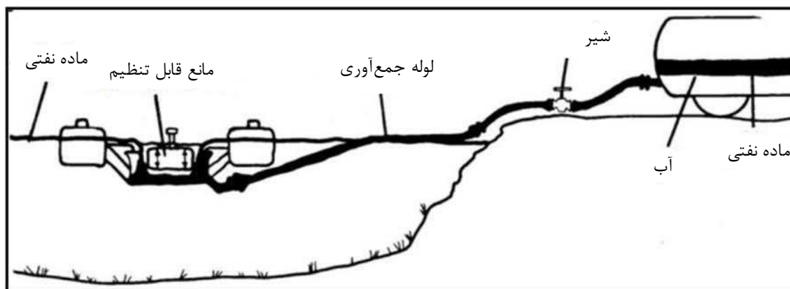
شکل پ. ۴-۳- نمای کلی از روش جمع‌آوری آلودگی نفتی با کمک بوم‌ها و اسکیمرها
