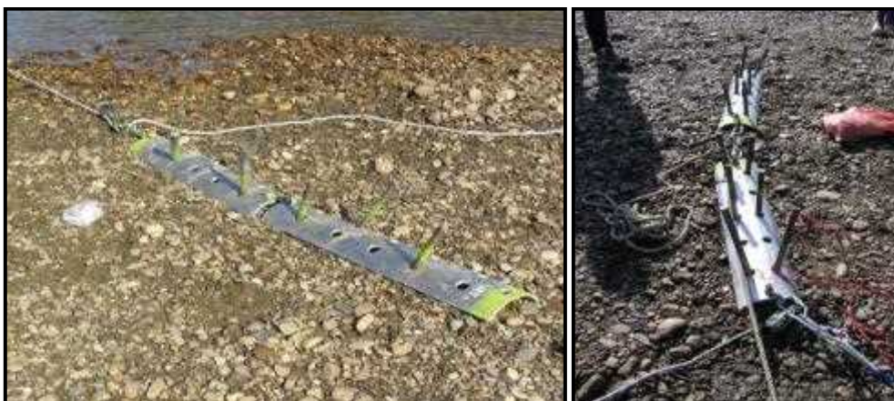
شکل پ.۴-۴- انواع تکیه‌گاه‌ها در بوم گذاری (تکیه‌گاه موقت در ساحل)
