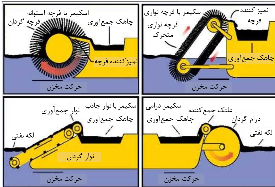
شکل پ. ۴-۵۳- انواع مختلف اسکیمرها (غلتنکی، نواری، پره‌ای و برسی)
