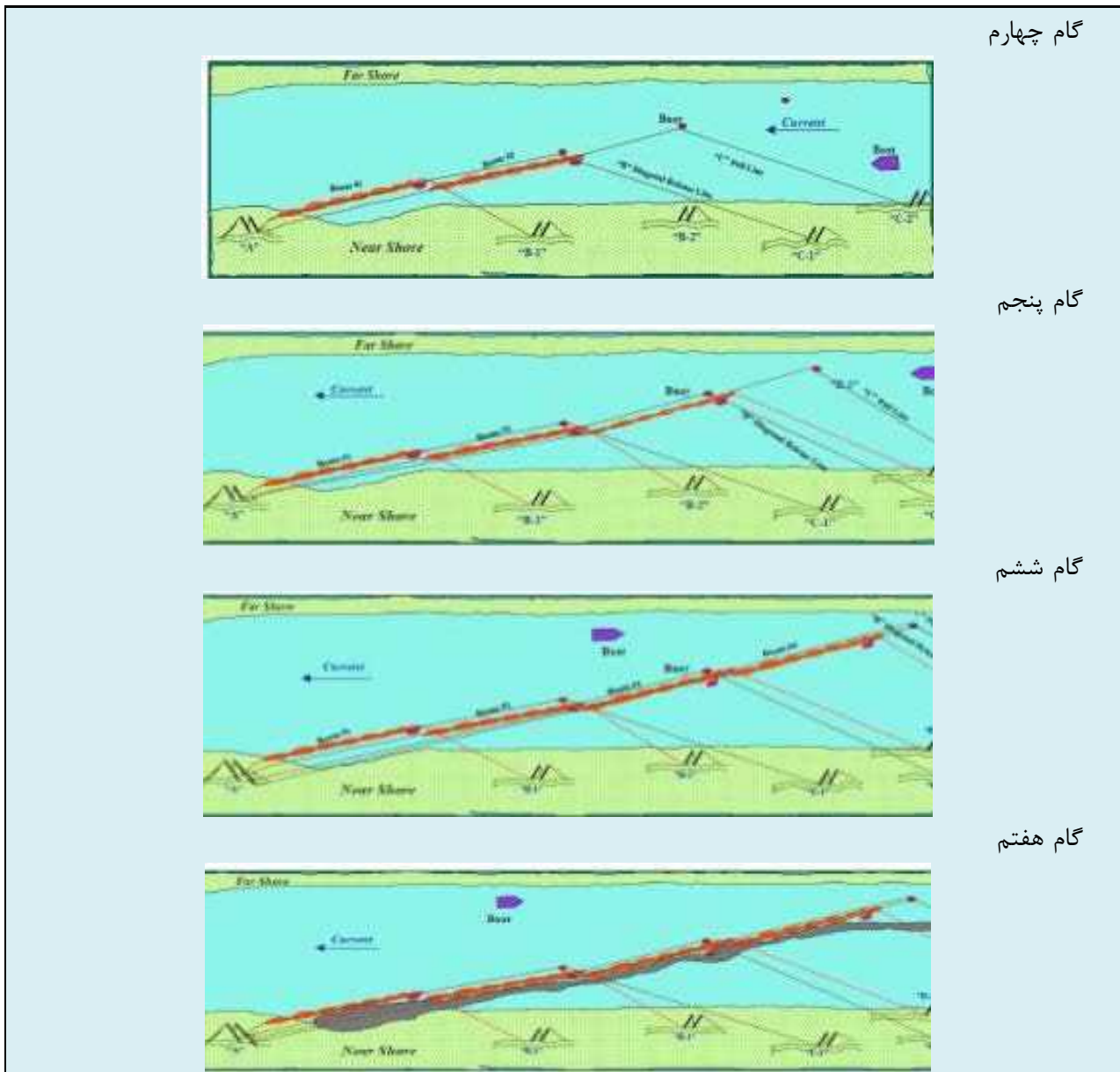
ادامه شکل پ.۴-۴- تکنیک بوم‌گذاری در رودخانه با آب سریع (ساحل به ساحل با تکیه‌گاه در آب)
