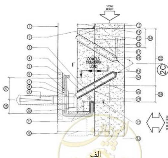
شکل ۴-۷- مقطعی از نمای سنگی متصل به دیوار بنایی با بلوک سیمانی به کمک لقمه‌های پشتیبان
