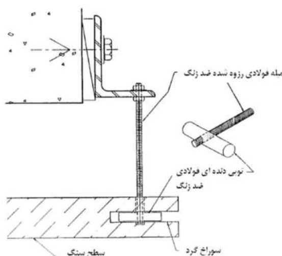
شکل ۴-۲۲ - مهار میله‌ای (Rod and plug anchor)
