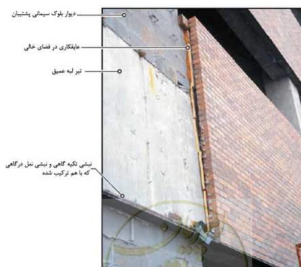
شکل ۵-۲۷- استفاده از نیشی‌های تکیه‌گاهی به جای نیشی‌های نعل درگاهی در نماهای آجری دارای پنجره‌های پیوسته
