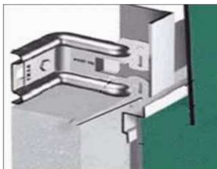
شکل ۴۹-۶- اجرای زیرسازی با استفاده از قطعات فولادی گالوانیزه شکل داده شده قابل تنظیم بر روی دیوارهای خارجی
