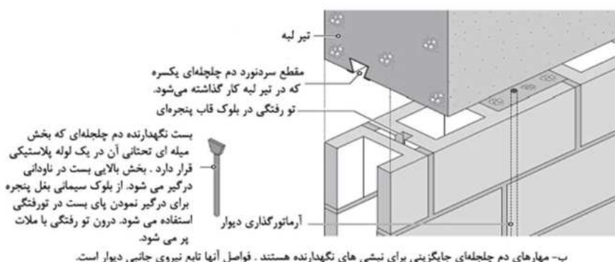
شکل ۵-۲۶- دو روش متداول برای ایجاد مقاومت در برابر بار جانبی در قسمت فوقانی دیواره های پشتیبان بلوک سیمانی
