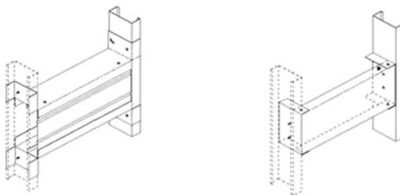
شکل ۵۰-۶- اجرای پشت‌بند برای تقویت موضعی زیرقاب و صفحات سیمانی
