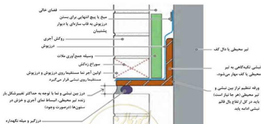
شکل ۵-۹- تکیه‌گاه‌ها جهت تحمل بار ثقیلی نما
