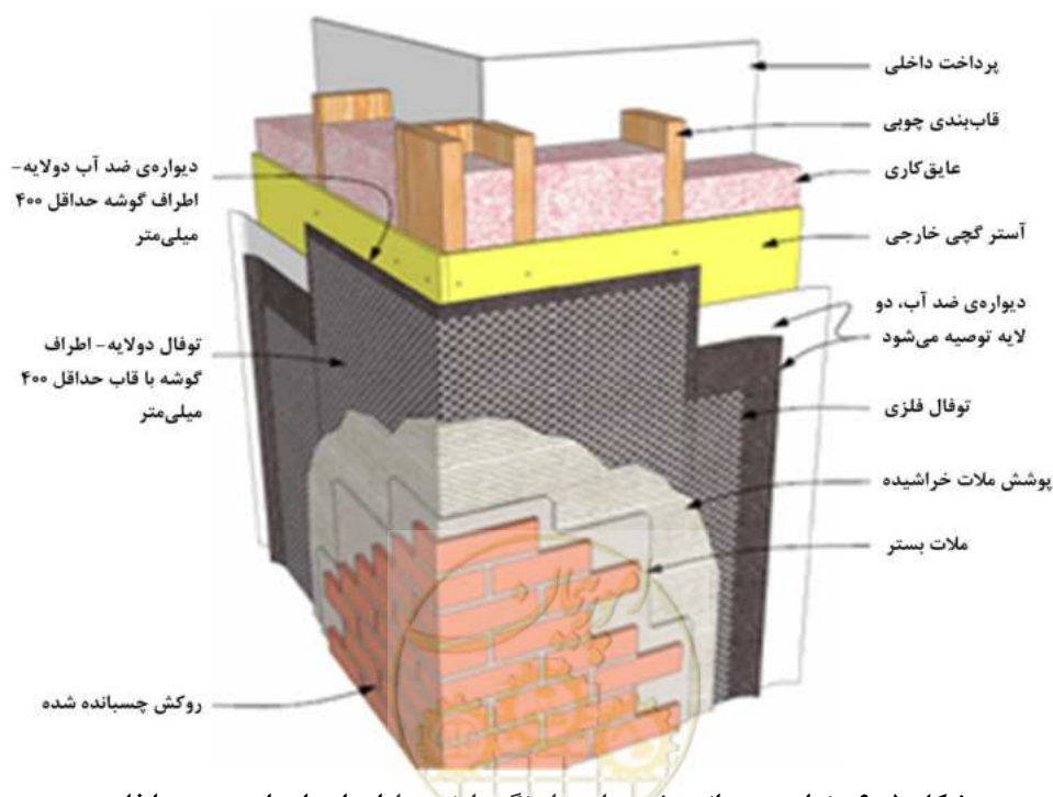
شکل ۵-۶- نمای چسبانده شده به دیوار نگهدارنده دارای استادهای چوبی یا فلزی
