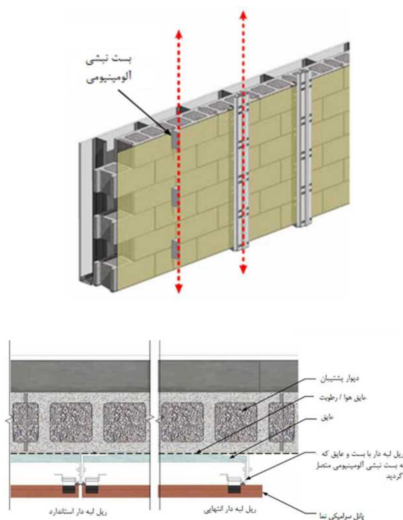
شکل ۷-۹- اتصال ریل لبه‌دار به وسیله پست نبشی شکل آلومینیومی به دیوار پشتیبان
