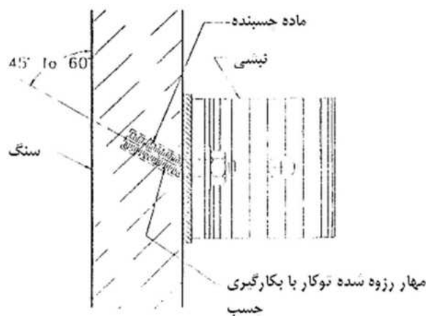
شکل ۴-۲- مهار رزوه شده توکار با بکارگیری چسب
