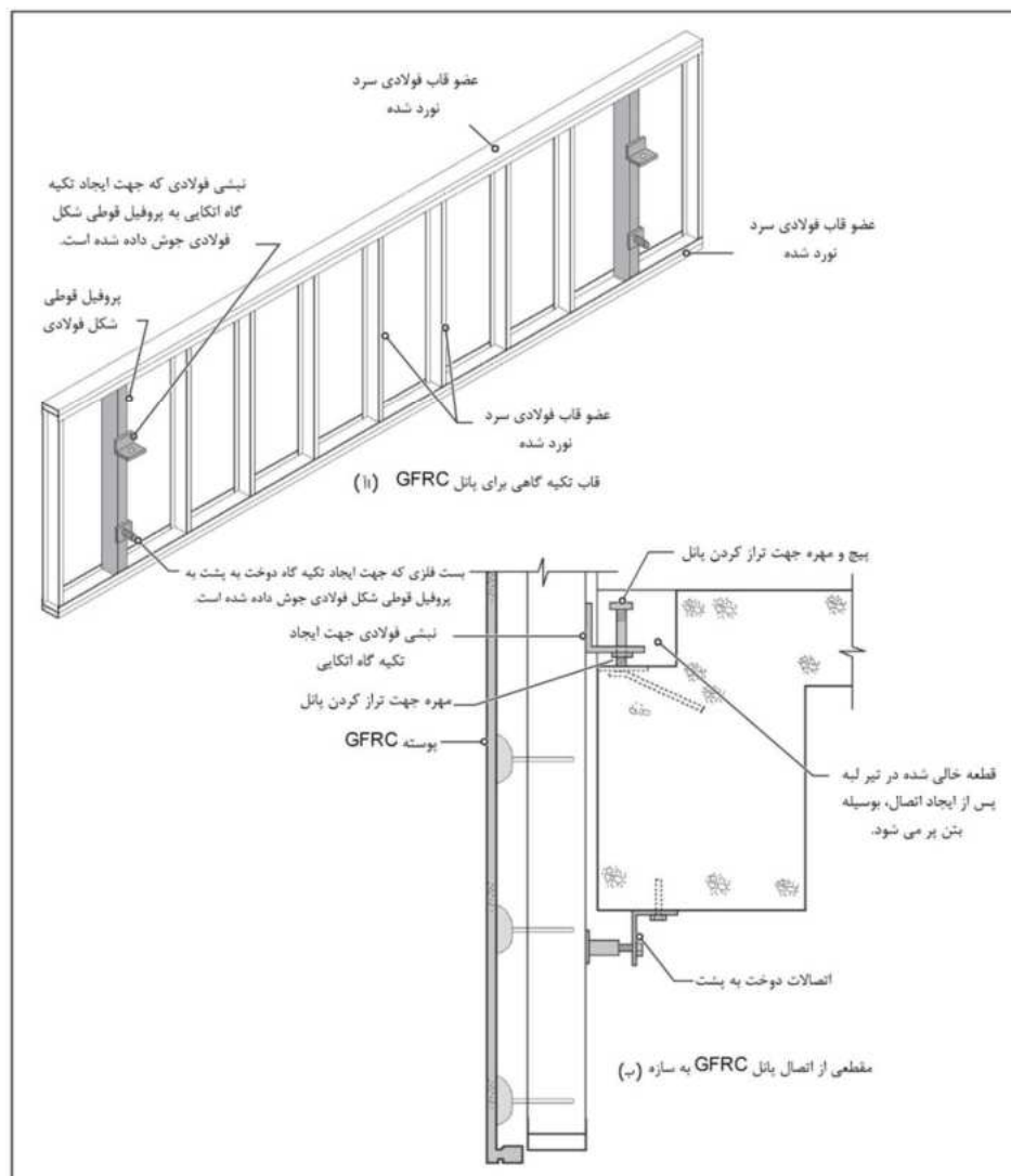
شکل ۶-۴۴ - تصویری شماتیک از جزئیات اتصالات اتکایی و دوجفت به پشت در پانل‌های پیرامونی GFRP
